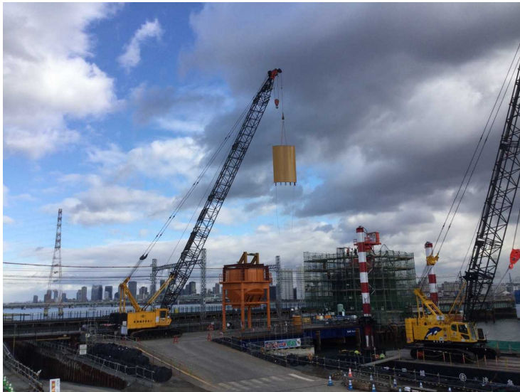
①ニューマチックケトン基礎工（側壁構築）
