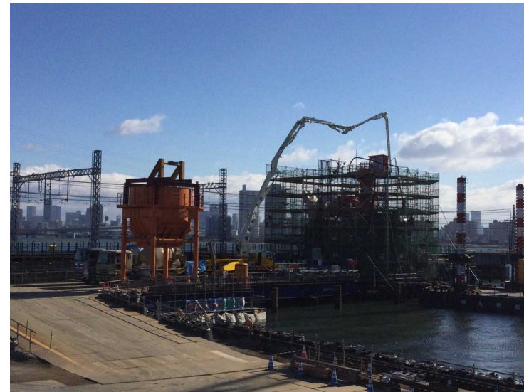
②ニューマチックケトン基礎工（側壁構築）
