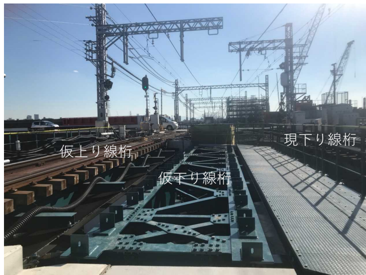
③仮線桁架設工
