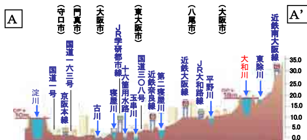
大阪平野断面図
