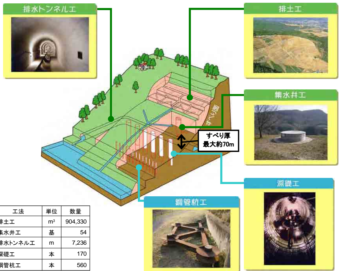
図 1.18 亀の瀬地すべり対策工模式図
