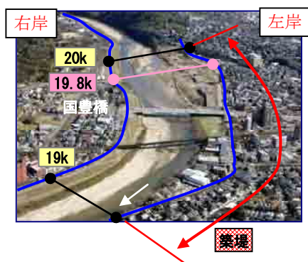
図 4.6 国分片山地区の河道整備イメージ
