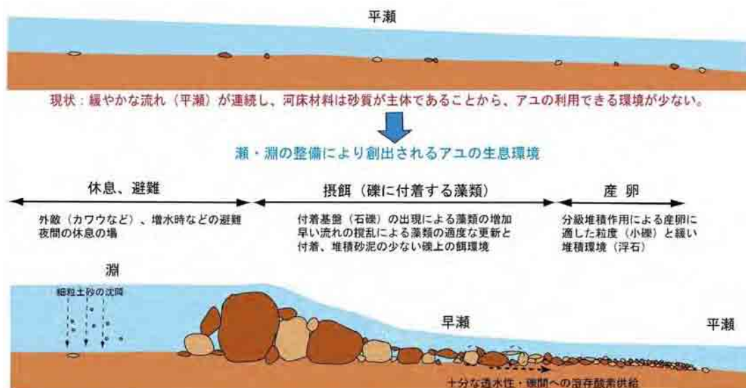
図 4.25 瀬・淵の再生のイメージ
