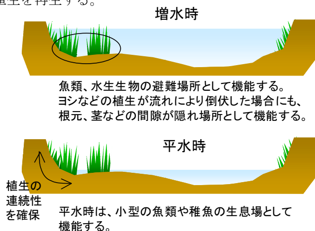
図 4.26 支川の河川水を利用した水際植生の再生イメージ(大和川7.2km)
