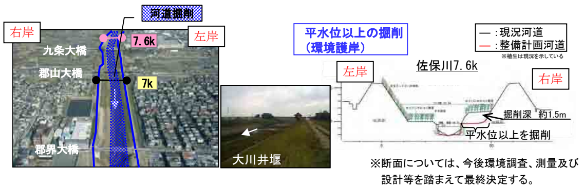
図 4.16 西九条地区の河道整備イメージ
