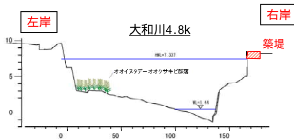
図 4.5 遠里小野地区の河道整備イメージ
