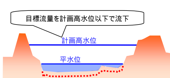
図 3.6 河道掘削のイメージ
