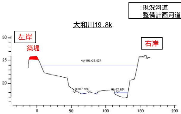
図 4.6 国分片山地区の河道整備イメージ
