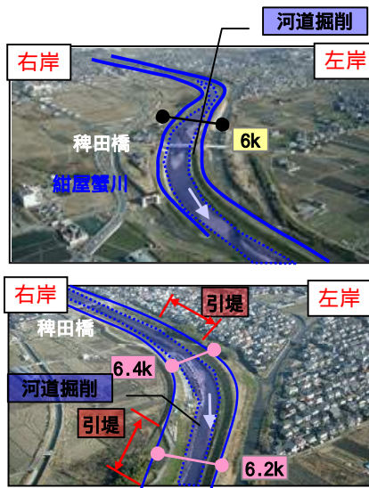
図 4.15 稗田・下三橋地区の河道整備イメージ
