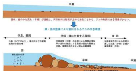
図 4.25 瀬・淵の再生のイメージ
