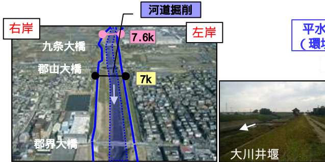
図 4.16 西九条地区の河道整備イメージ
