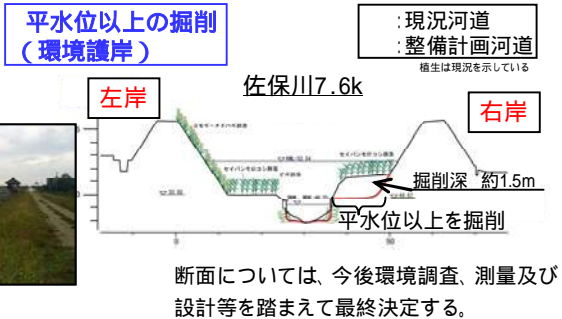
図 4.16 西九条地区の河道整備イメージ
