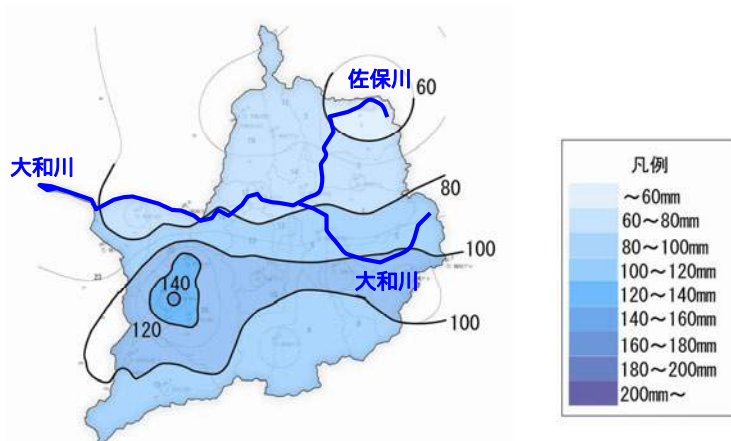
図 1.15 12 時間雨量分布図(平成 19 年 7 月洪水)
