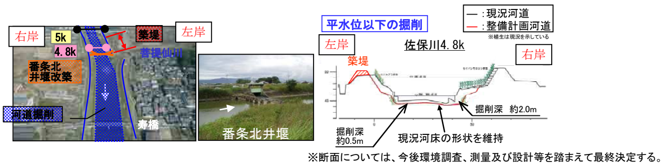
図 4.14 番条北地区の河道整備イメージ
