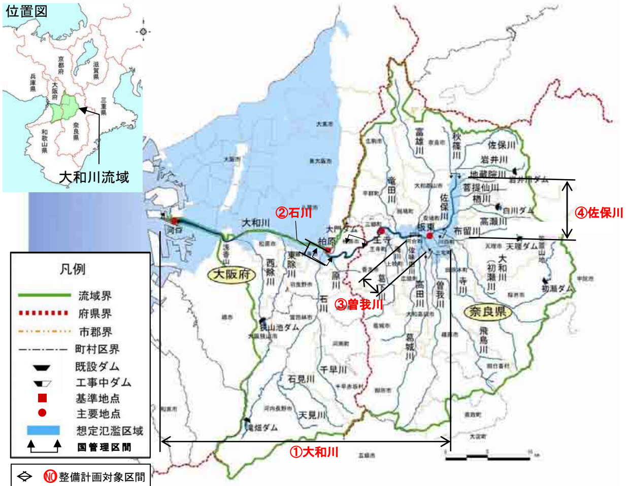
図 3.5 河川整備計画対象区間
