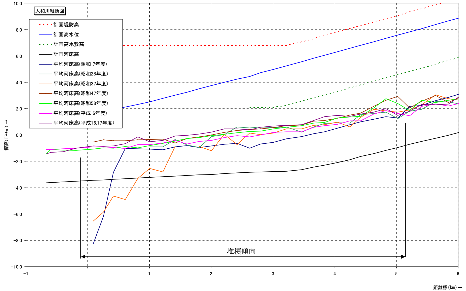
図 2.3 大和川河口部の河床高の経年変化
