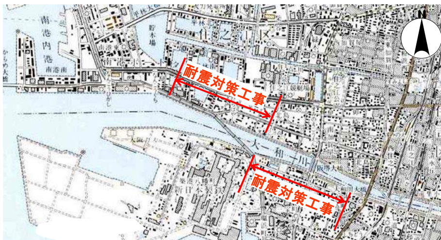
図 4.19 これまでの耐震対策工事区間
