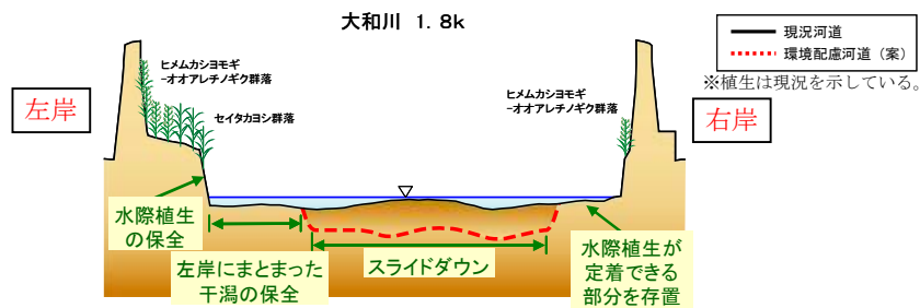
図 4.24 河口部の河道掘削イメージ
