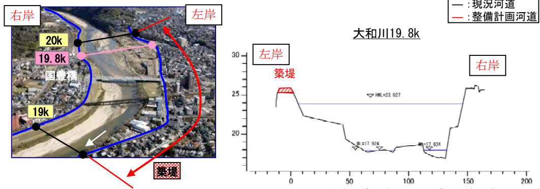
図 4.6 国分片山地区の河道整備イメージ
