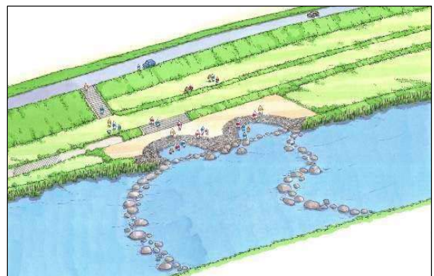
図 4.29 若林地区水辺空間整備(案)イメージ
