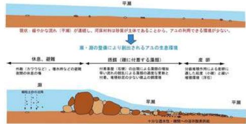
図 4.26 瀬・淵の再生のイメージ
