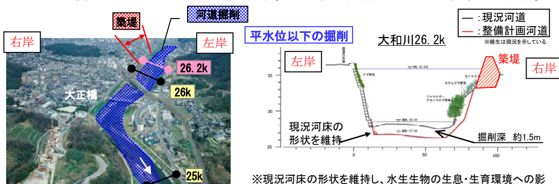
図 4.9 藤井、 さんごう 三郷地区の河道整備イメージ
