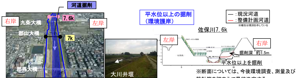
図 4.16 西九条地区の河道整備イメージ
