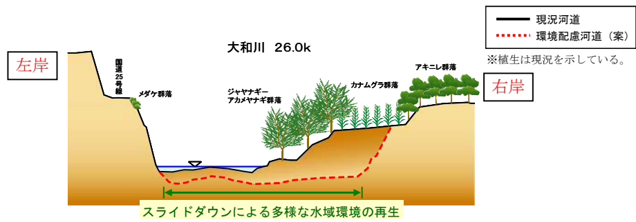
図 4.22 中流部の河道掘削イメージ
