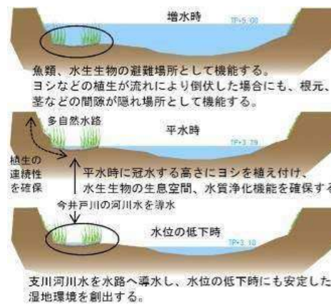
図 4.27 支川の河川水を利用した水際植生の再生イメージ
