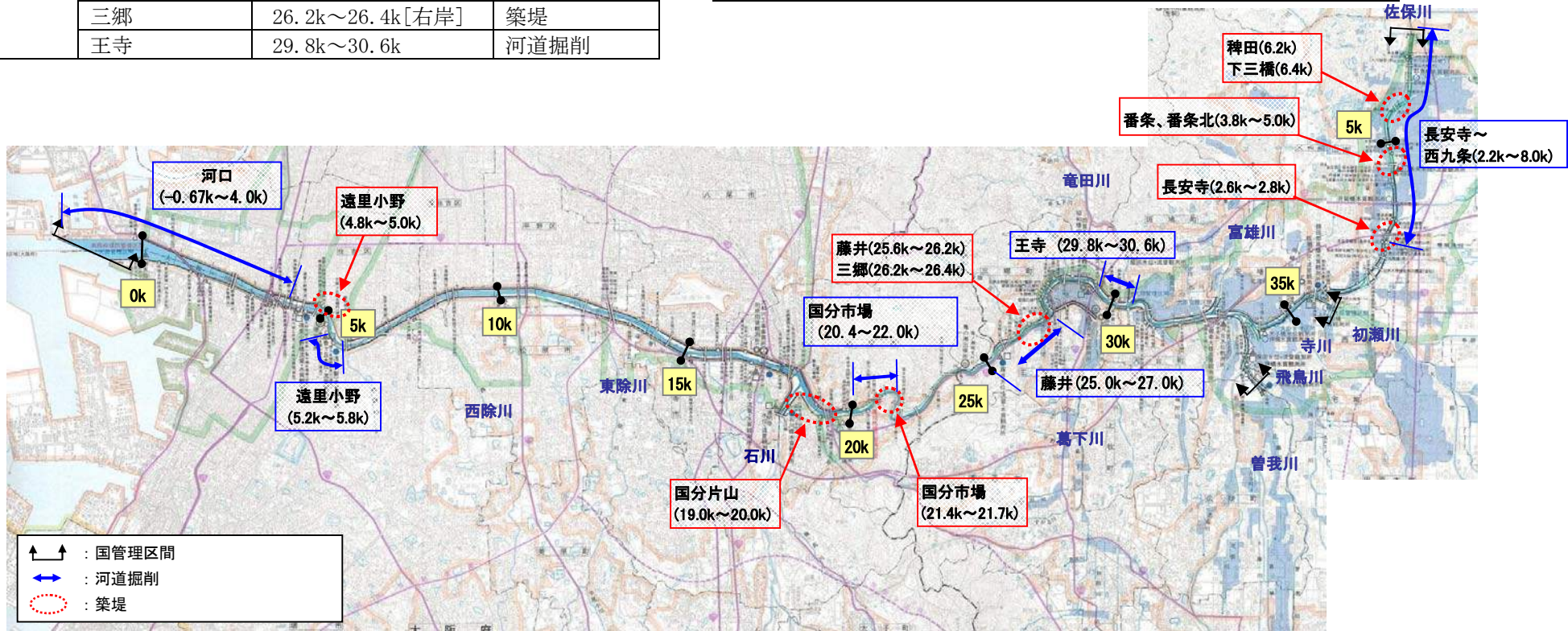
図 4.17 河道整備箇所位置図
