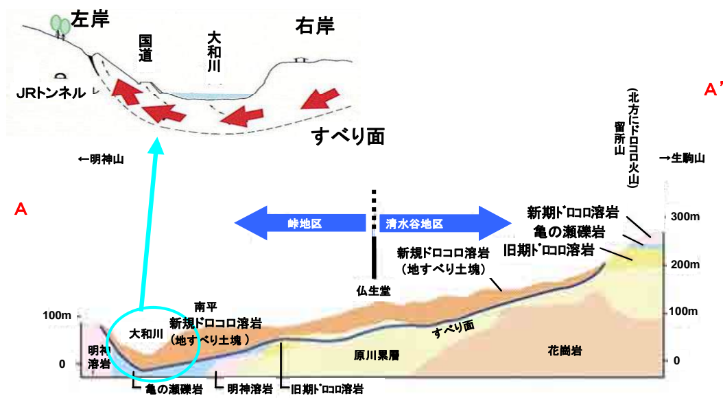
図 1.7 亀の瀬地すべり地帯の断面図
