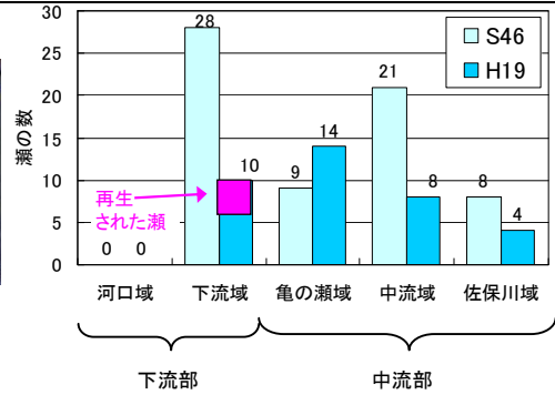
図 2.5 瀬の減少
