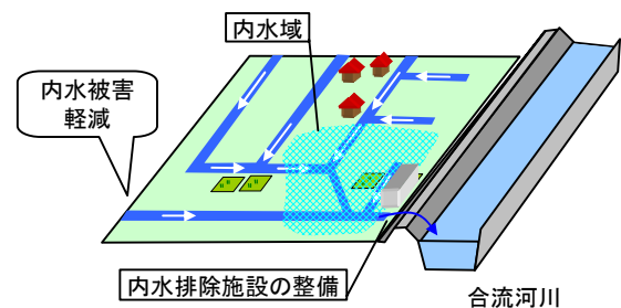
図 3.10 内水対策のイメージ
