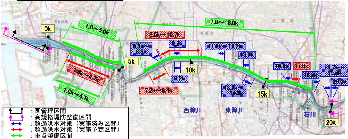
図 4.21 超過洪水対策の整備箇所位置図(平成 22 年 6 月現在)
