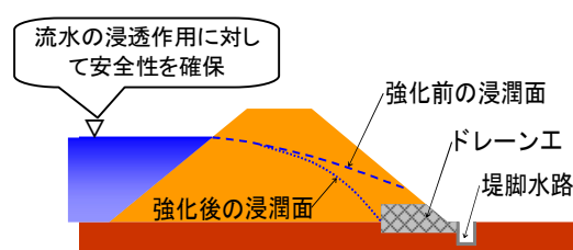
図 3.11 堤防浸透対策(ドレーン工法)のイメージ
