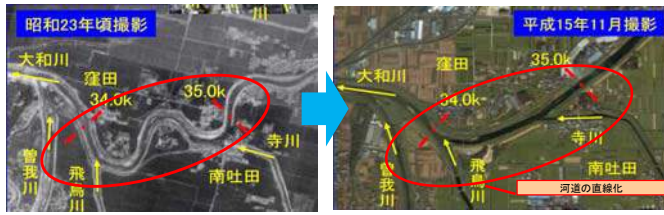
図 2.4 捷水路による瀬淵の減少(大和川 35k 付近)
