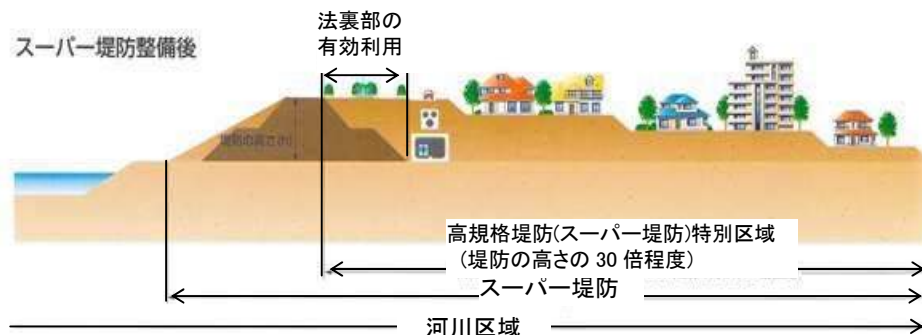
図 4.20 高規格堤防イメージ図
