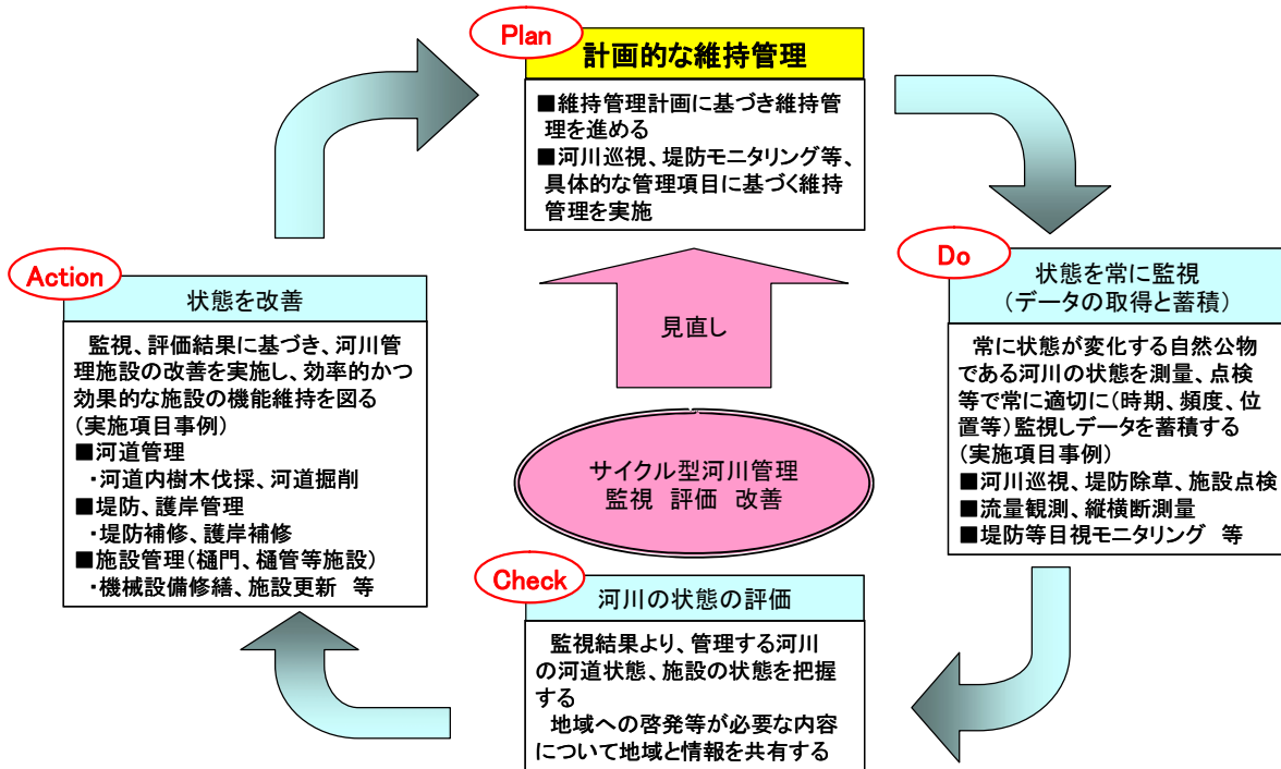
図 4.31 サイクル型維持管理の体系図
