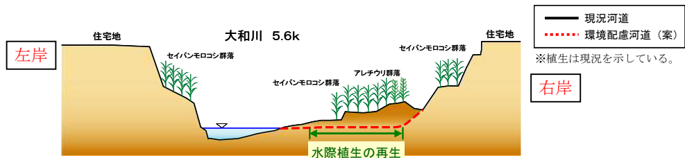
図 4.23 下流部の河道掘削イメージ
