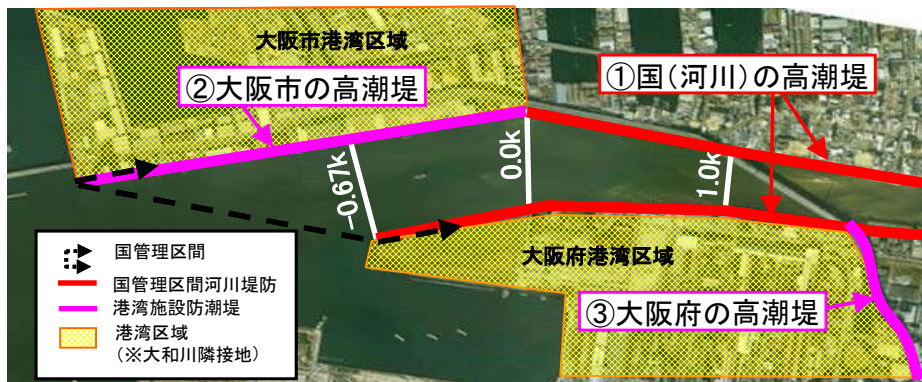
図 4.35 河口付近の高潮対策
