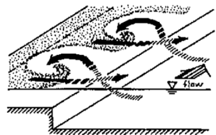
大規模平面渦に伴う流れの三次元構造
