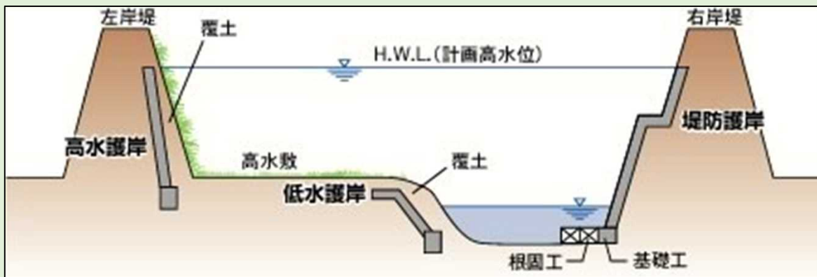
高水護岸工事のイメージ図
