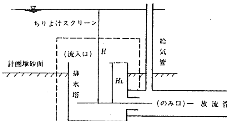
図3-5 放流施設流入部構造
