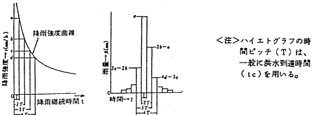
図2-1 ハイトグラフの作り方
