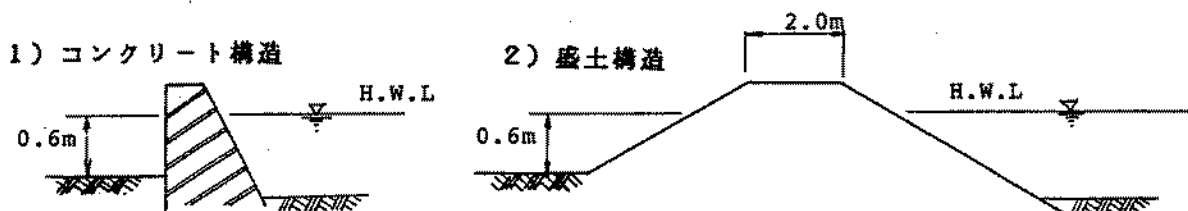
図3-1 小堤・小掘込式
