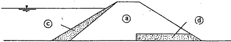
(1) 均一形ダム
