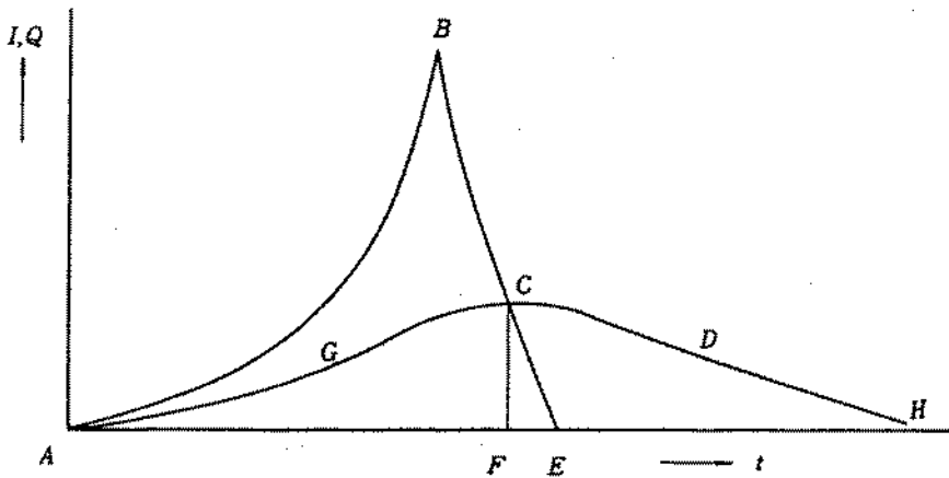
図 2-5 流入流出ハイドログラフ
