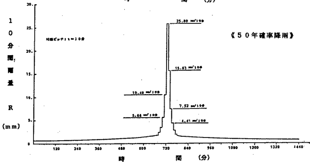
図2-2 中央集中型確率降雨波形
