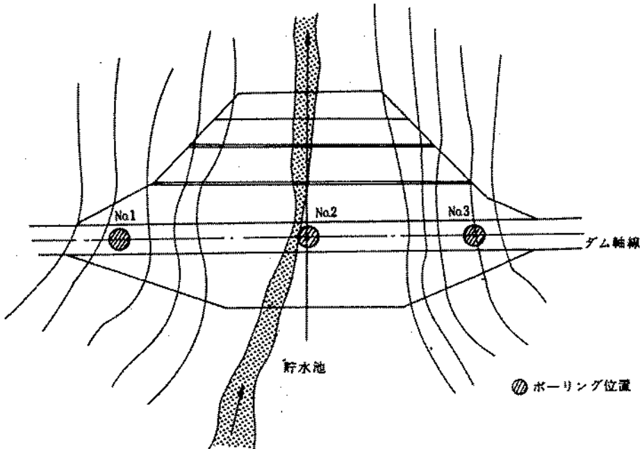
図 3-3 ボーリング位置図
