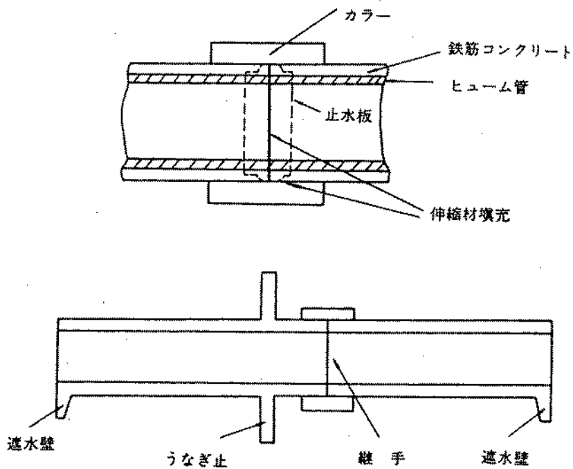
図3-6 継手・遮水壁の設計例
