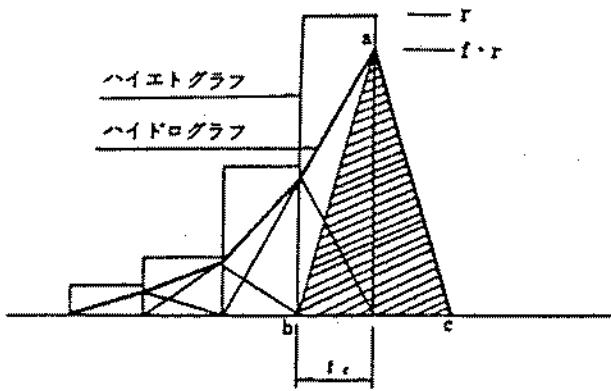
図 2-4 流出ハイドログラフの計算法
