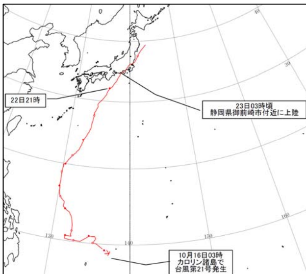
台風経路図
