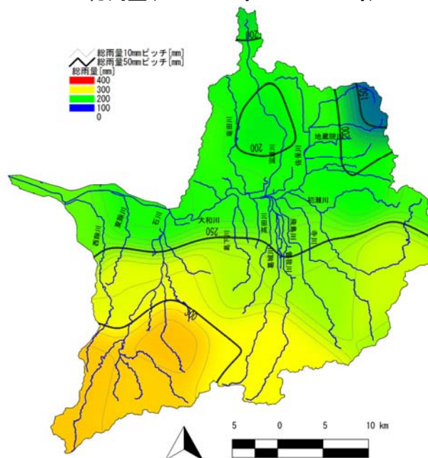
雨量の分布
