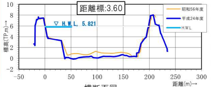
横断面図
