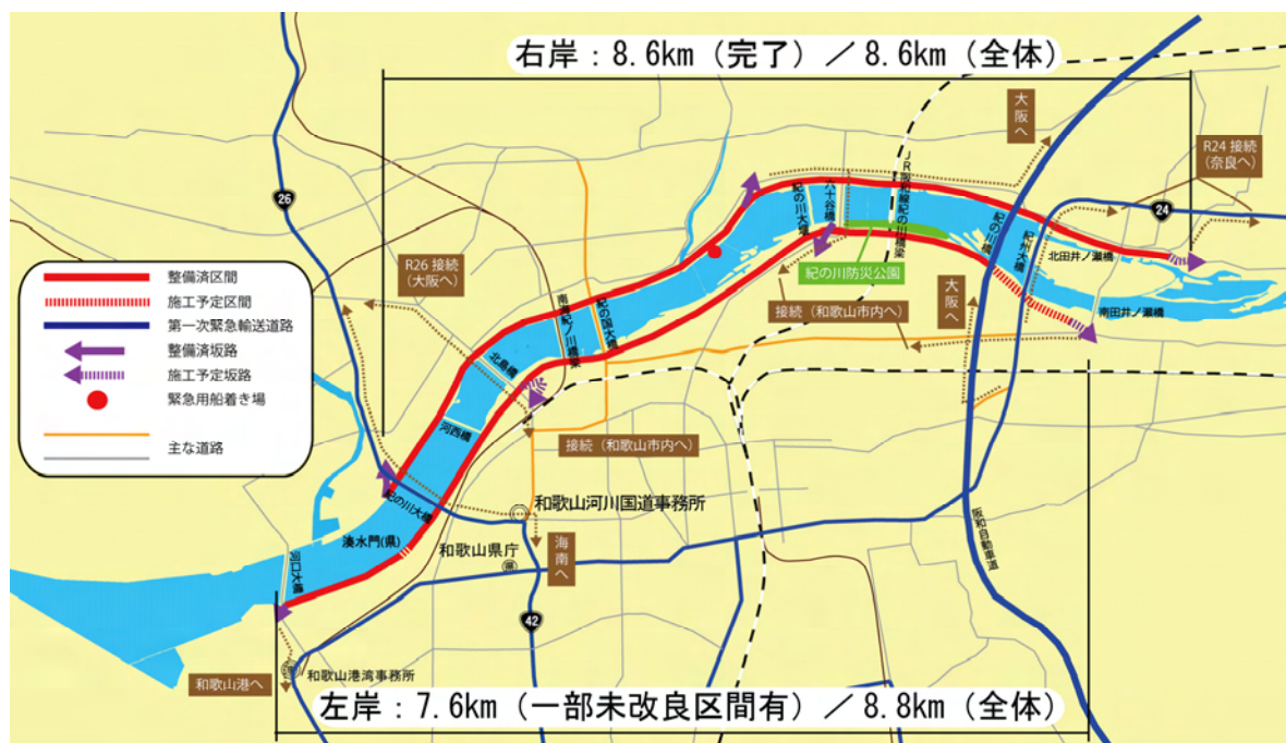
図 4.1.6 緊急用河川敷道路施工予定図
