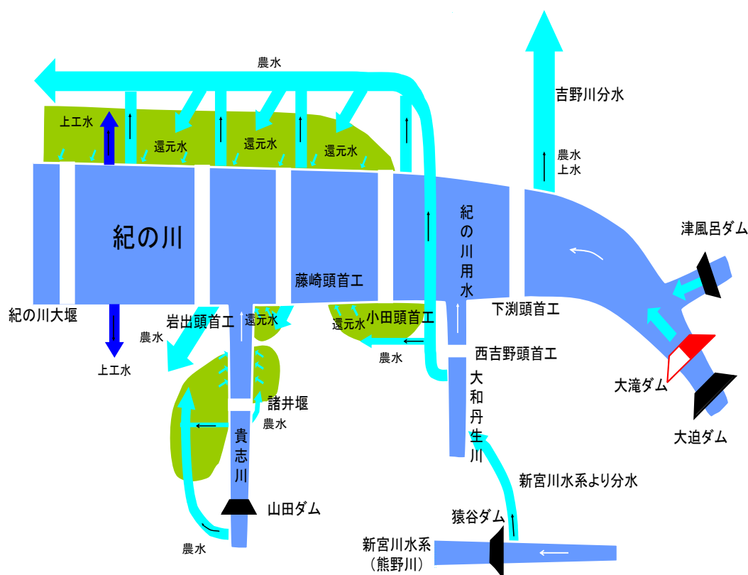
図 1.2.2 利水概要図
