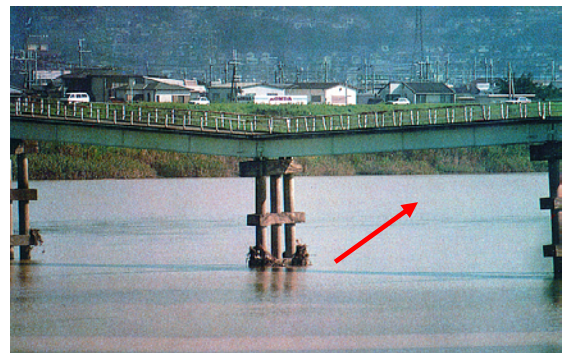
写真 1.2.6 川底がえぐり取られて陥没した南海橋（平成 2 年台風 19 号）
