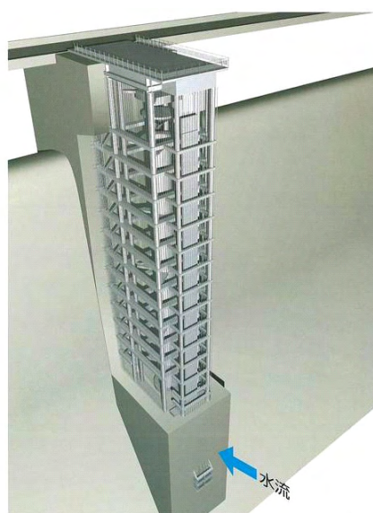
図 2.4.7 大滝ダム-選択取水設備
