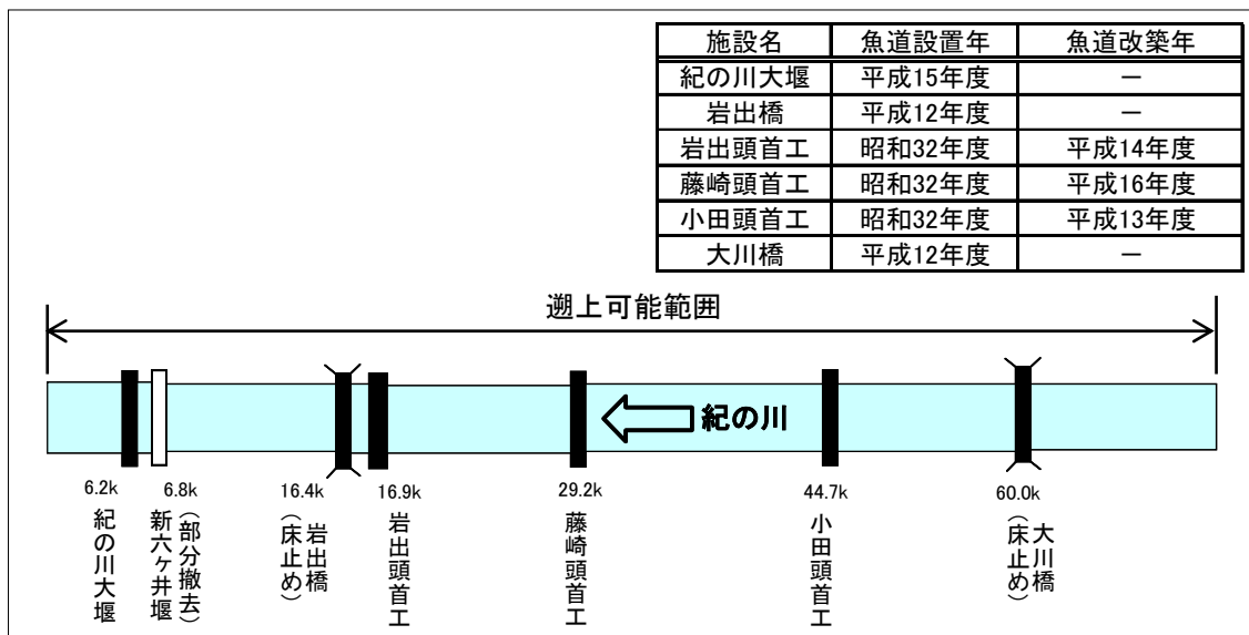
図 2.3.1 魚道の現状
