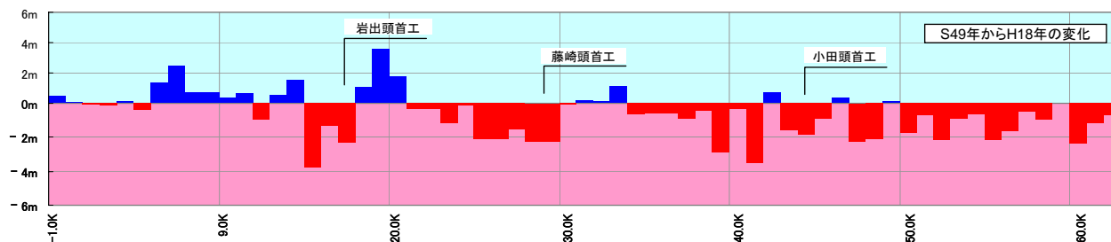
図 2.4.5 砂利採取禁止以降の最深河床の変化量
