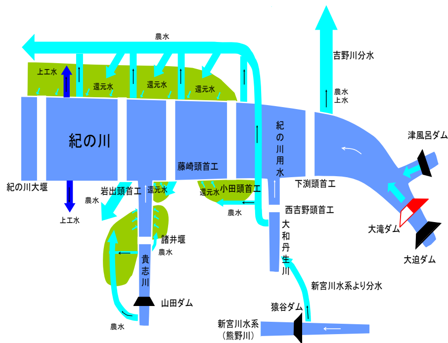
図 2. 2. 2 利水概要図
