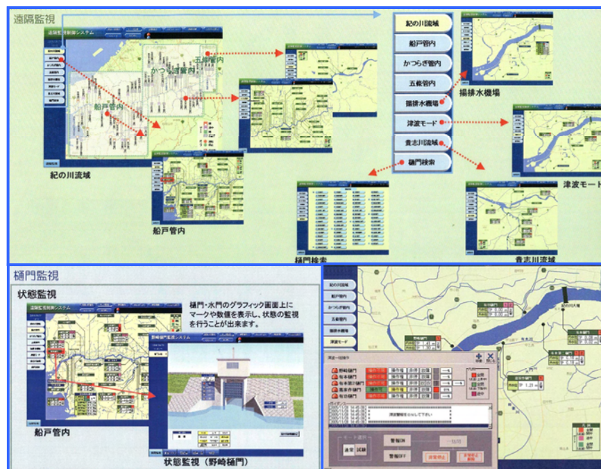
図 4.4.1 運転支援システム（樋門監視と遠隔操作）
