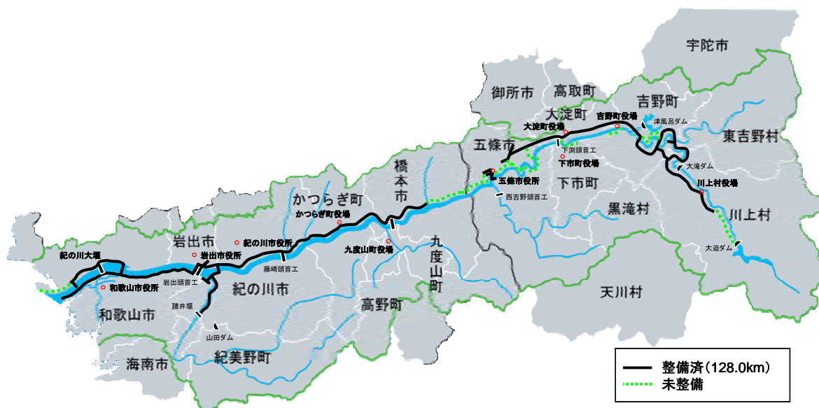
図 4.1.8 紀の川の光ファイバーネットワーク
