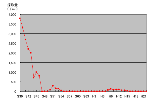
図 2.4.3 砂利採取の推移
