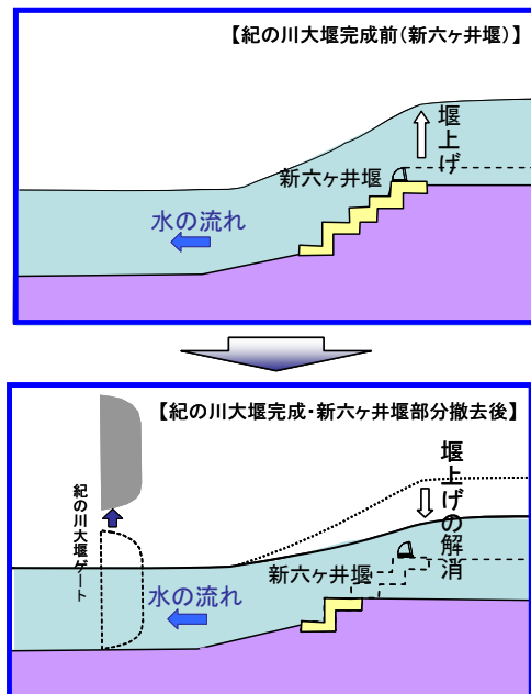
図 2.1.3 紀の川大堰による効果
