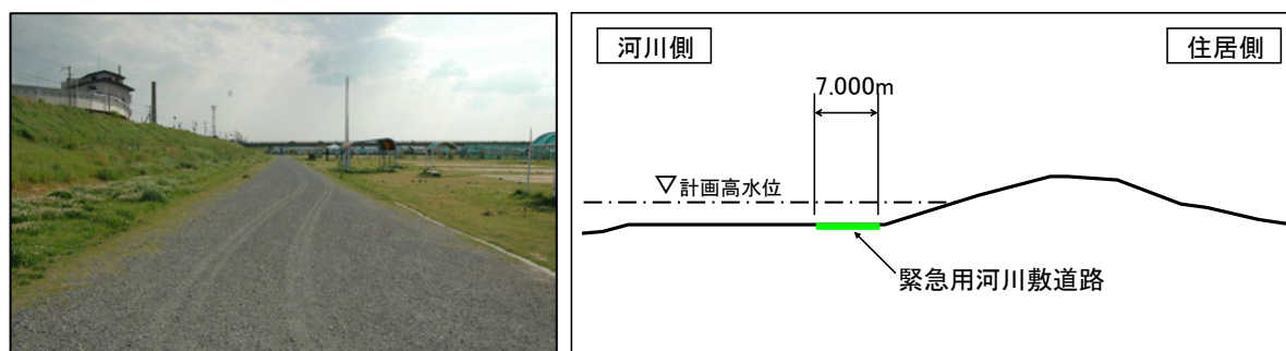
図 4.1.7 緊急用河川敷道路（左岸 3.4k 付近）（左）と横断図（右）
