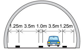
【標準断面図】
