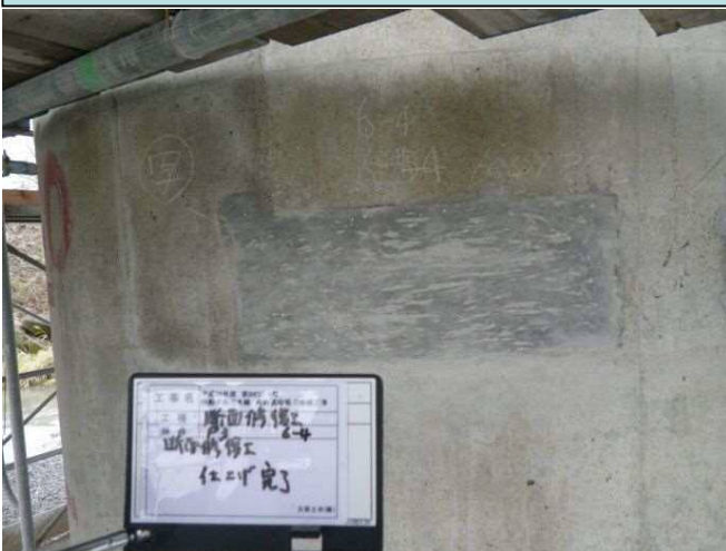
断面修復
