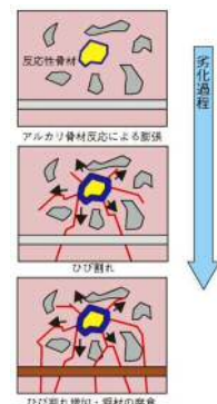
アルカリ骨材反応のメカニズム
