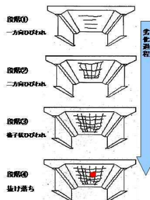
床版の疲労損傷のメカニズム
