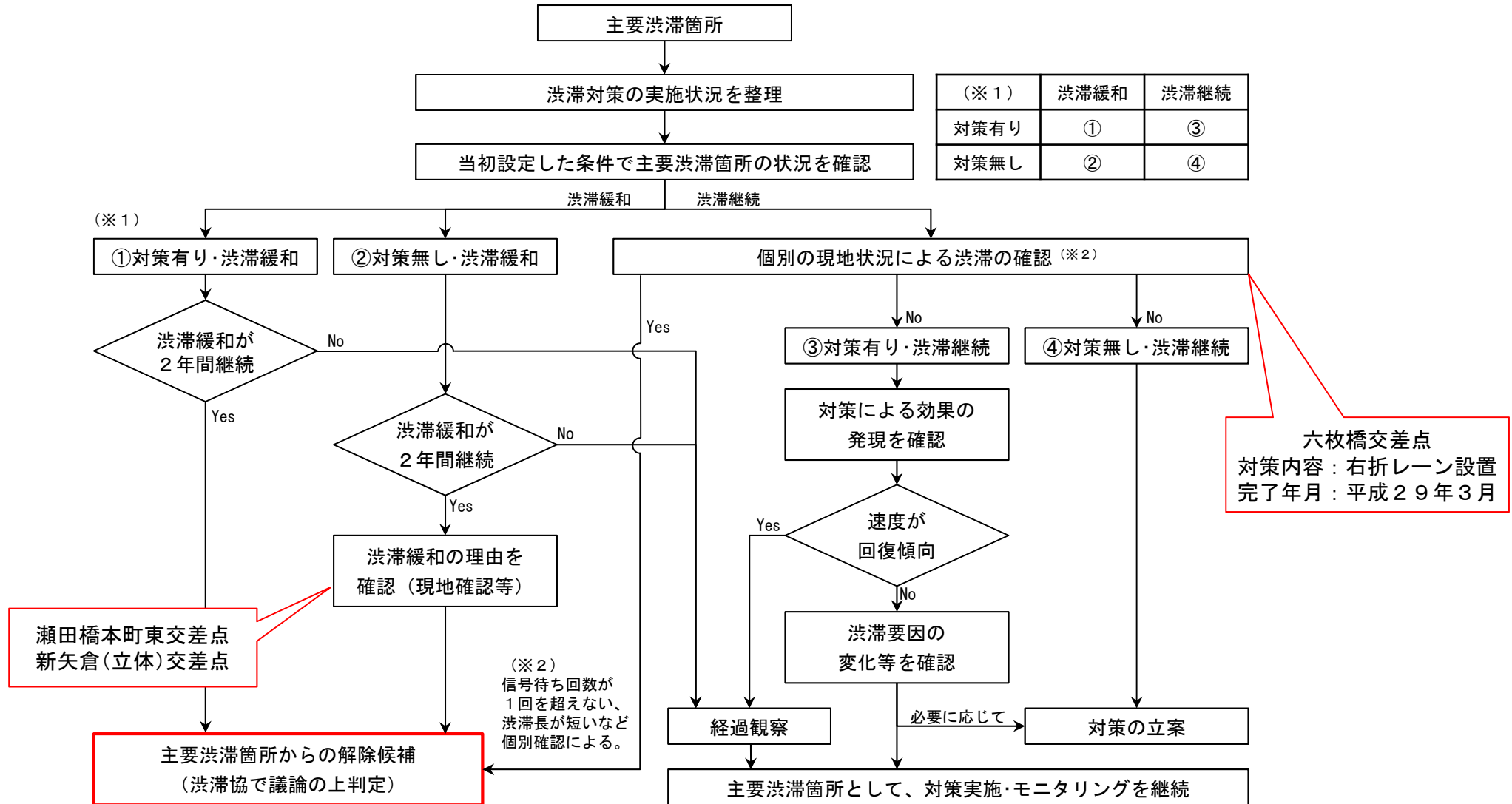
▲主要渋滞箇所の特定解除フロー
