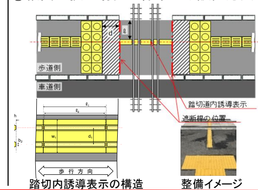
踏切道内誘導表示の構造 整備イメージ
