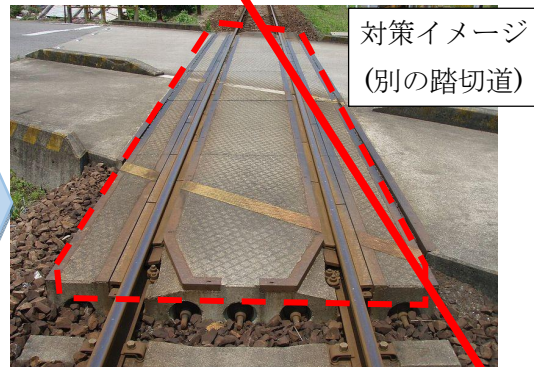
写真 2-1-32 踏切内の平滑化のイメージ
