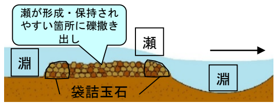
図 瀬淵タイプの使い分けイメージ
