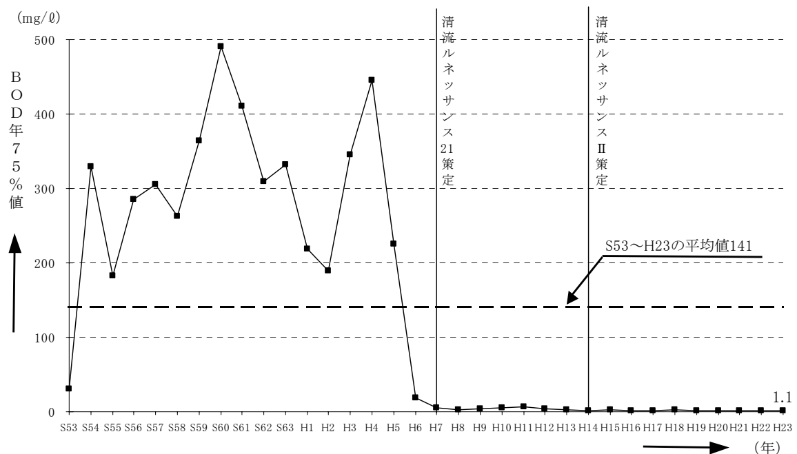
図-5.23 揖保川水系林田川 かまえ 構地点（真砂橋）における水質の経年変化
