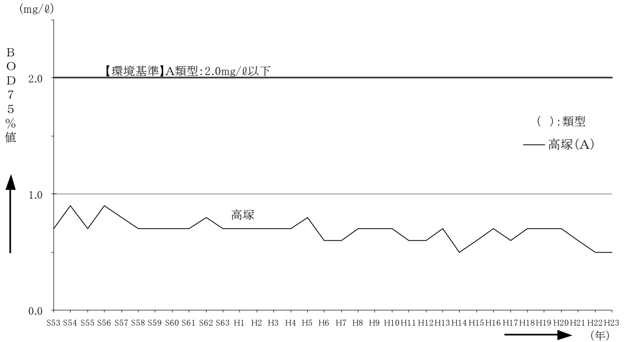
図-5.50 北川水系の環境基準地点の水質経年変化（BOD75%値）
