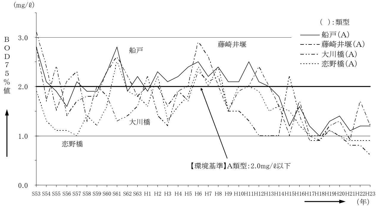
図-5.31 紀の川水系の環境基準地点の水質経年変化（BOD75%値）
