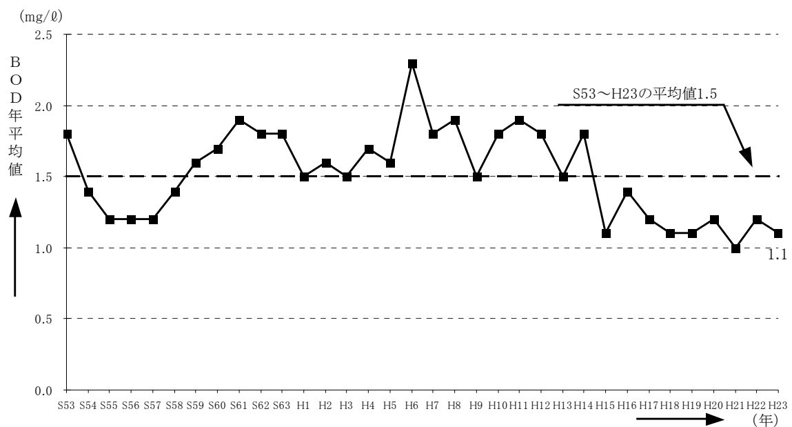
図-5.10 紀の川の水質経年変化 (BOD年平均値)
