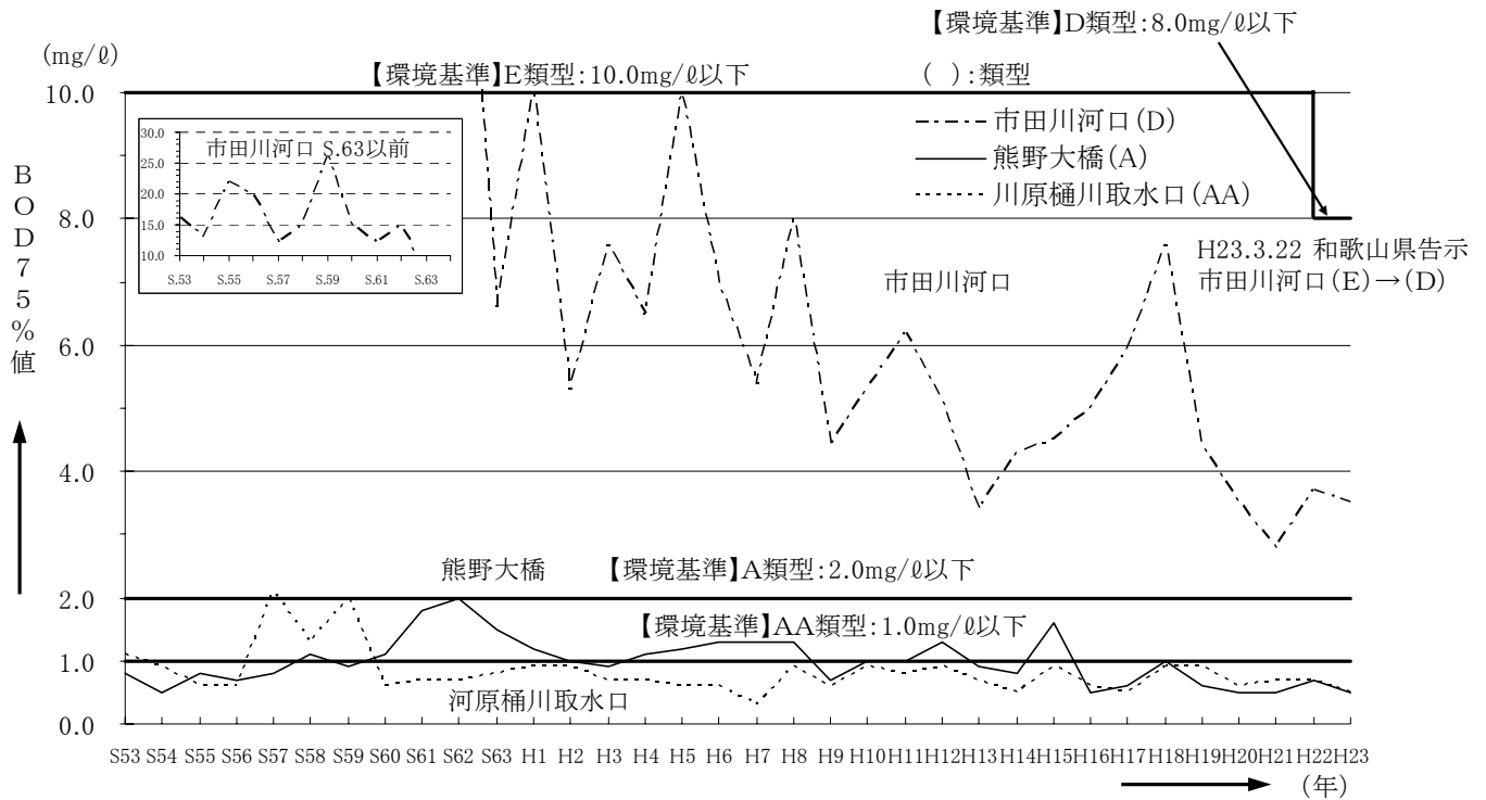
図-5.29 新宮川水系の環境基準地点の水質経年変化 (BOD75%値)
