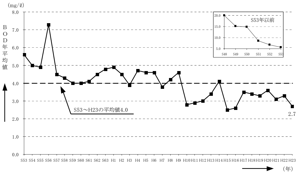
図-5.20 猪名川の水質経年変化 (BOD年平均值)
