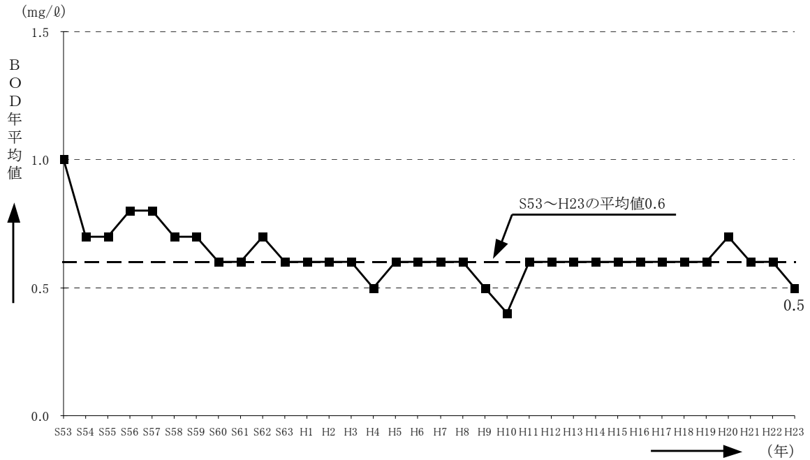
図-5.26 北川の水質経年変化 (BOD年平均值)
