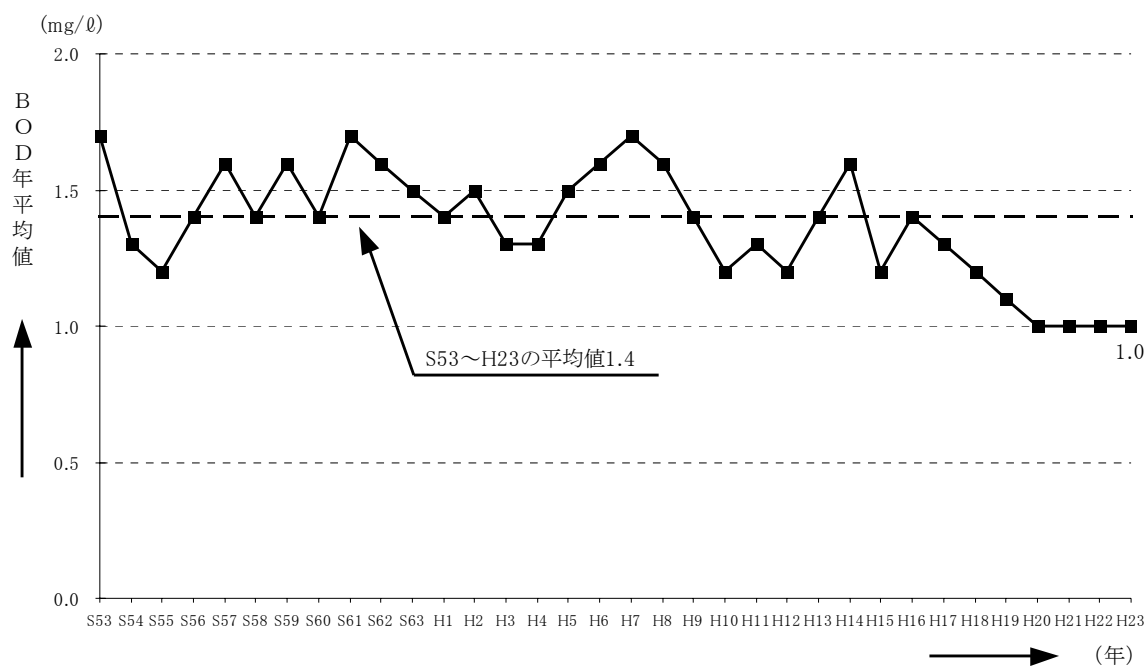
図-5.18 名張川の水質経年変化 (BOD年平均值)
