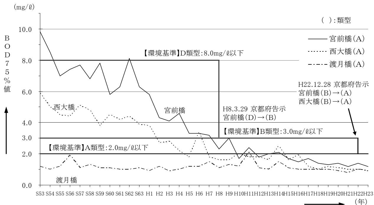
図-5.38 淀川水系（桂川）の環境基準地点の水質経年変化（BOD75%値）
