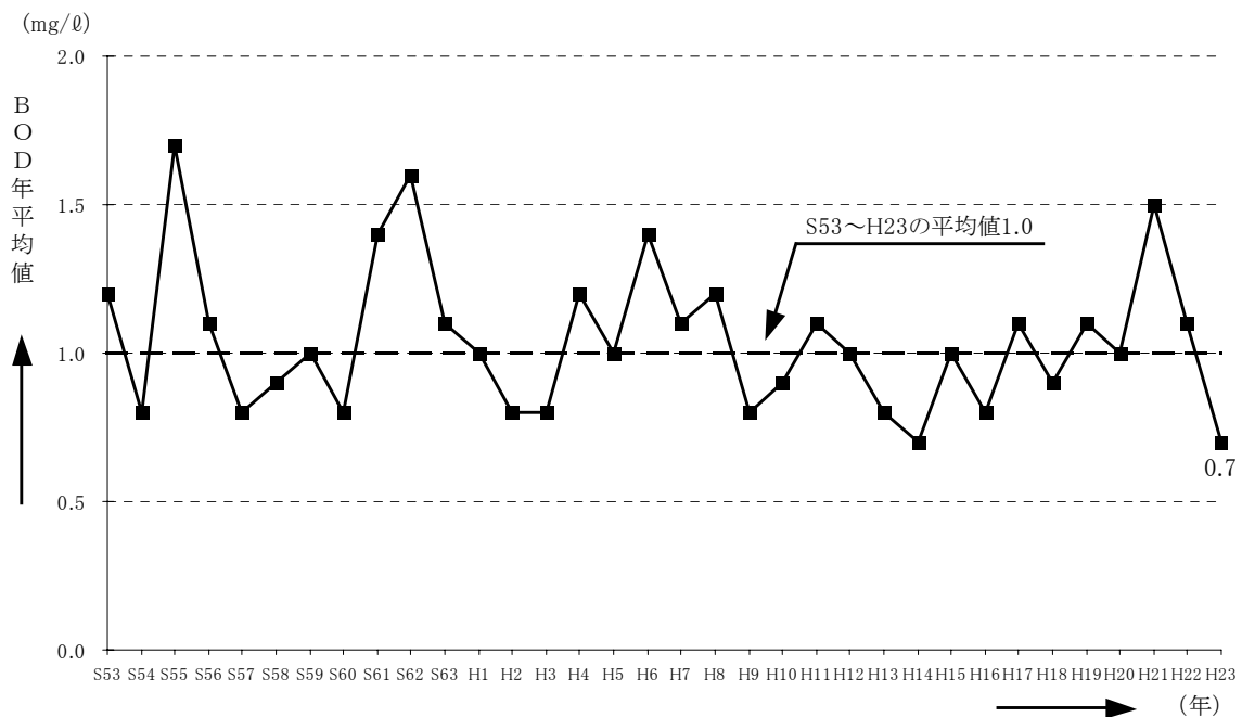
図-5.9 熊野川の水質経年変化 (BOD年平均値)
