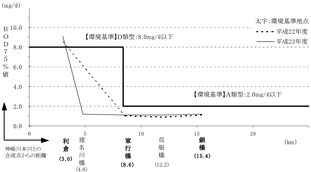
図-5.43 猪名川の水質縦断図（BOD75%値）
