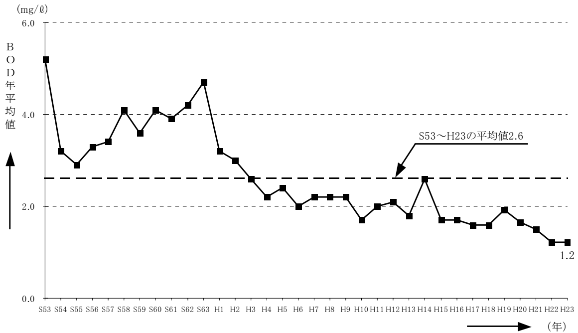
図-5.13 淀川本川（三川合流点下流）平均水質の経年変化
