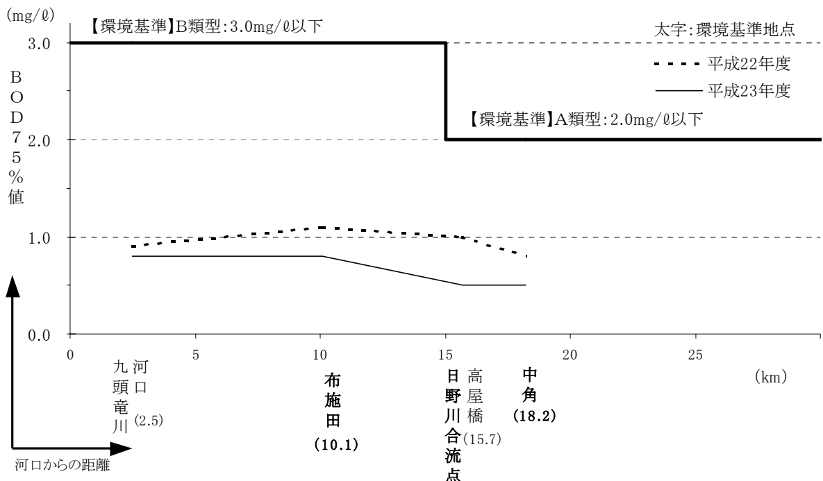
図-5.49 九頭竜川の水質縦断図（BOD75%値）
