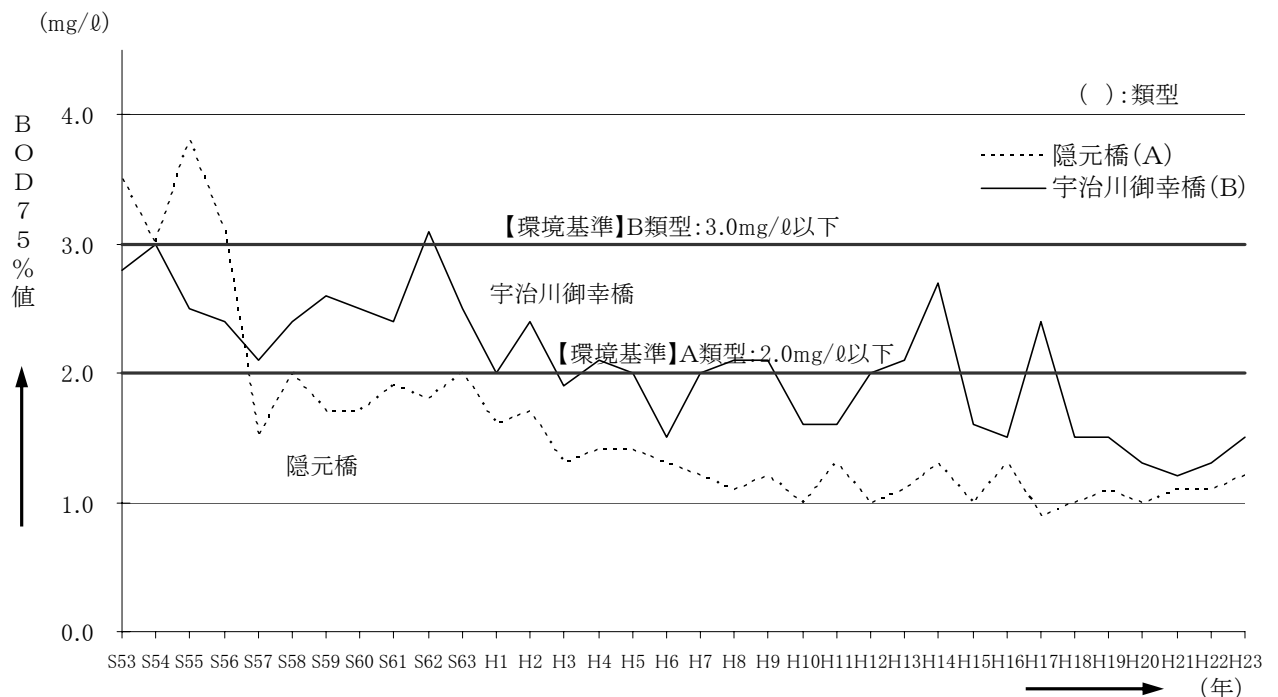
図-5.36 淀川水系（宇治川）の環境基準地点の水質経年変化（BOD75%値）
