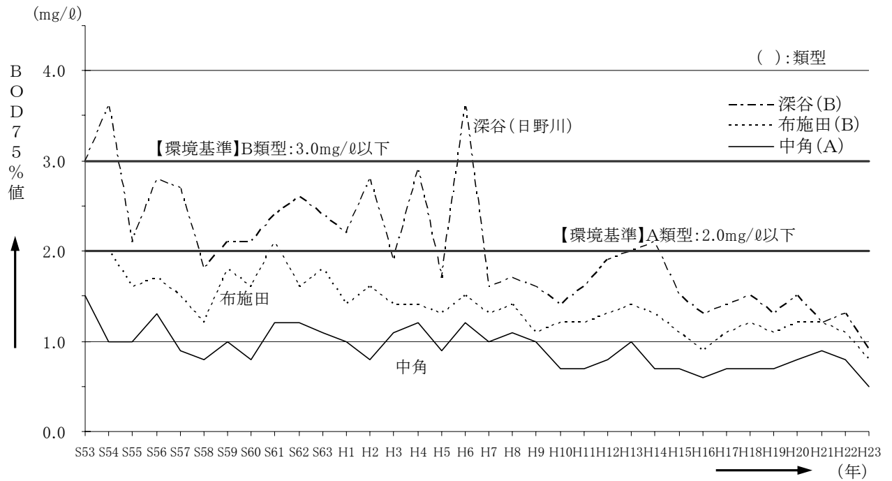
図-5.48 九頭竜川水系の環境基準地点の水質経年変化（BOD75%値）
