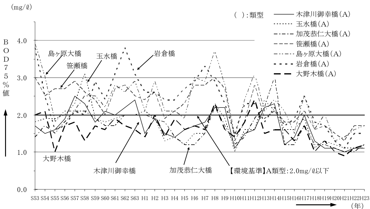
図-5.40 淀川水系（木津川）の環境基準地点の水質経年変化（BOD75%値）
