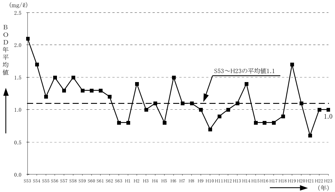
図-5.24 円山川の水質経年変化 (BOD年平均值)
