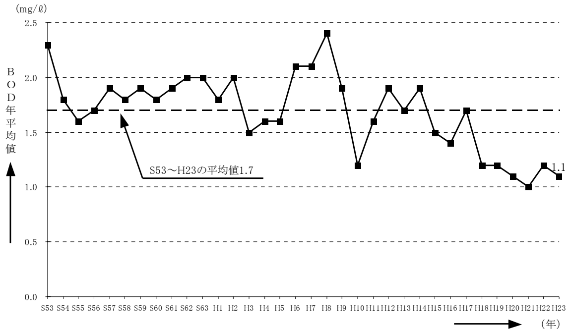
図-5.19 木津川の水質経年変化 (BOD年平均值)
