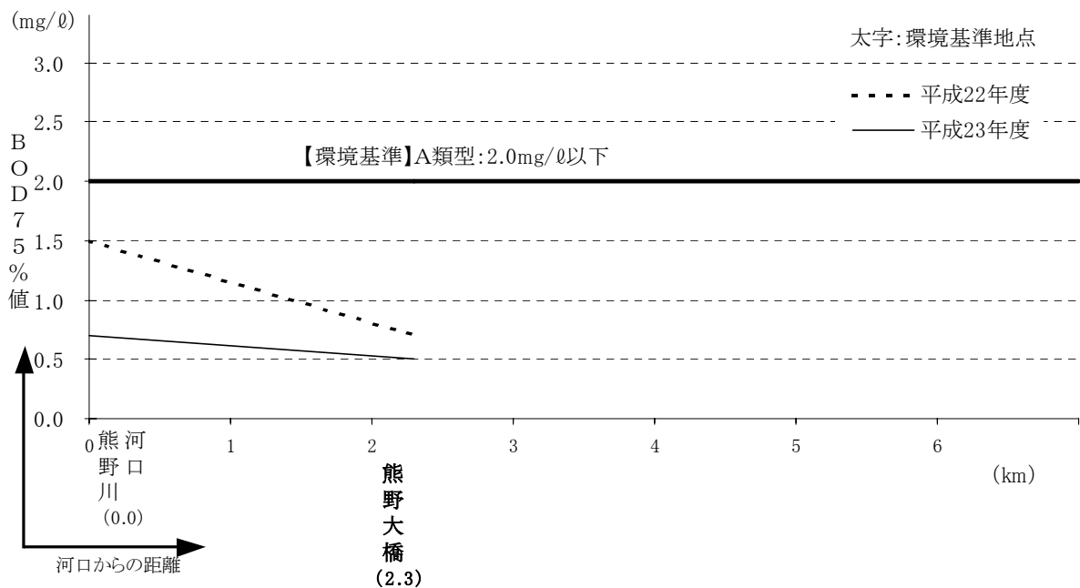
図-5.30 熊野川の水質縦断図 (BOD75%値)
