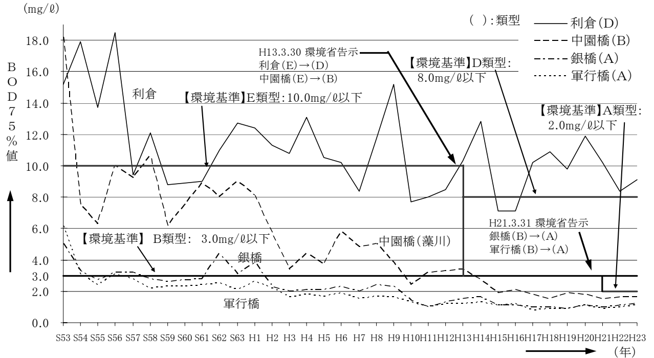
図-5.42 淀川水系（猪名川、藻川）の環境基準地点の水質経年変化（BOD75%値）
