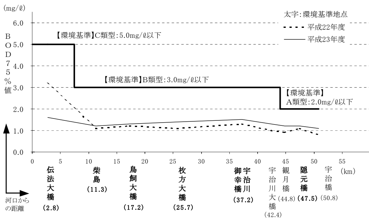
図-5.37 淀川（本川、宇治川）の水質縦断図（BOD75%値）
