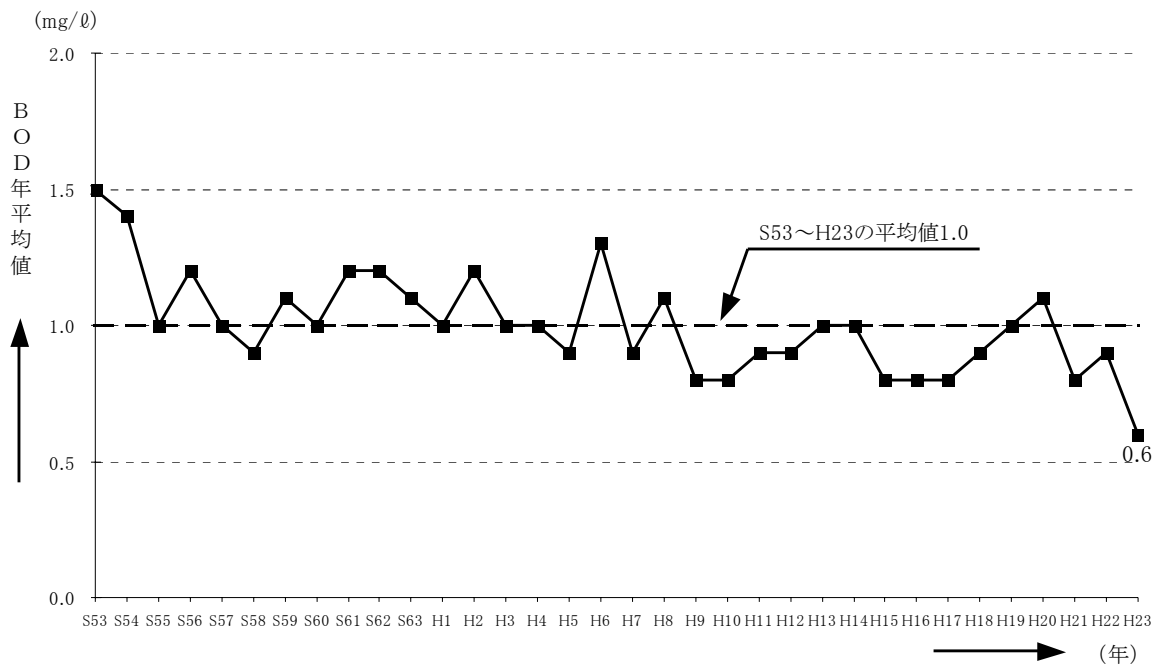
図-5.27 九頭竜川の水質経年変化 (BOD年平均值)
