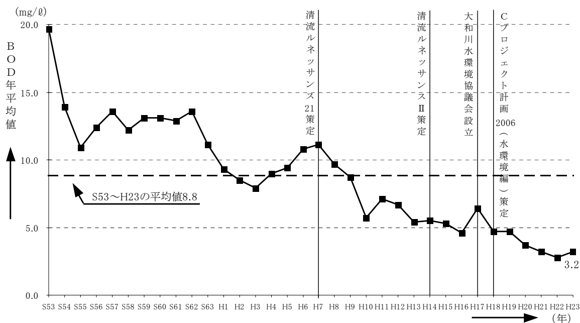
図-5.11 大和川の水質経年変化（BOD年平均値）
