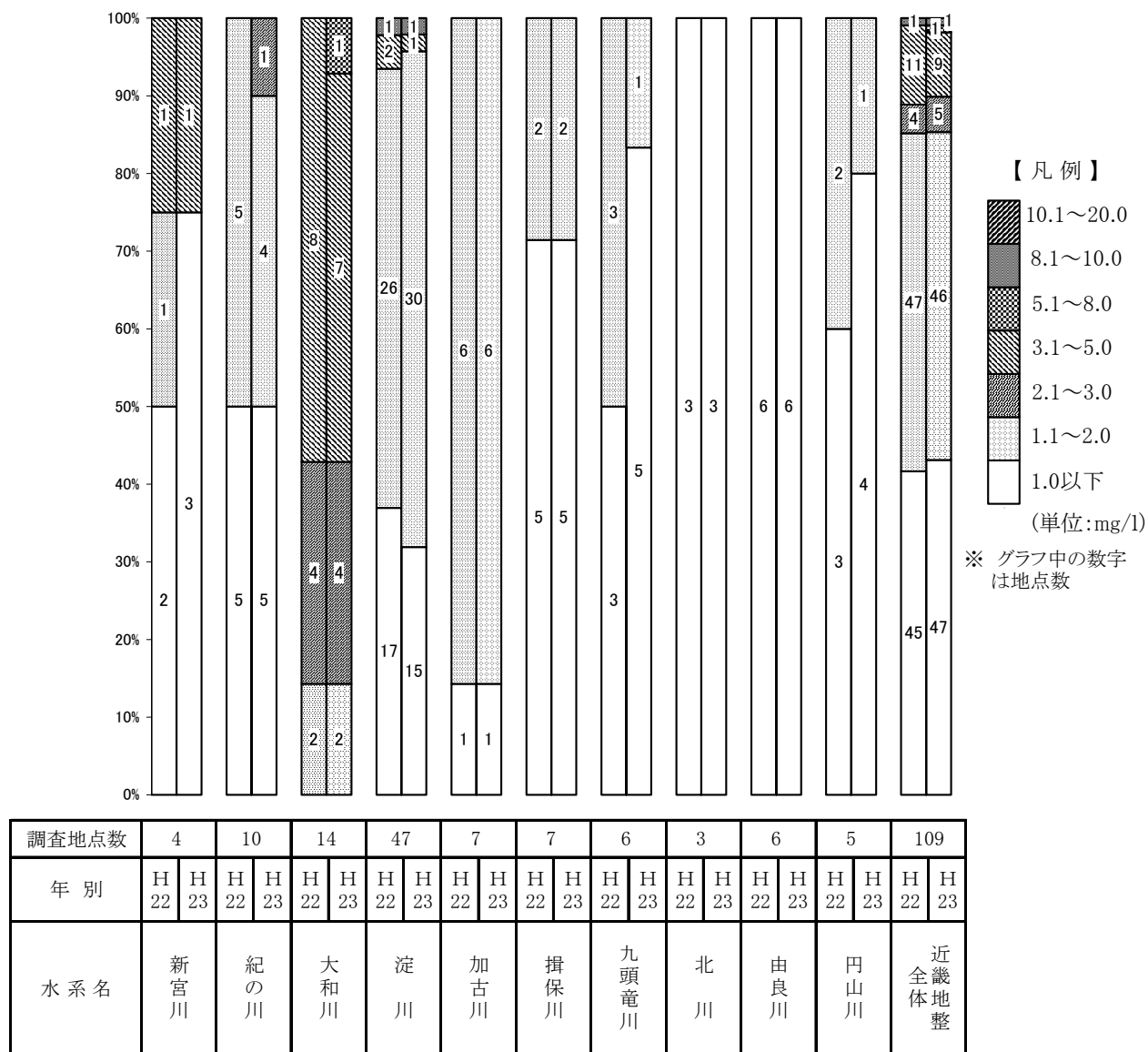
図-5.6 水系別BOD75%値のランク別割合（平成22年 108地点，平成23年 109地点）
