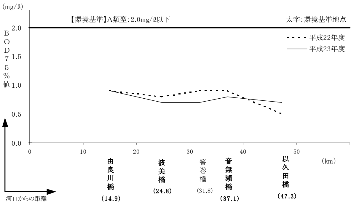
図-5.53 由良川の水質縦断面図（BOD75%値）
