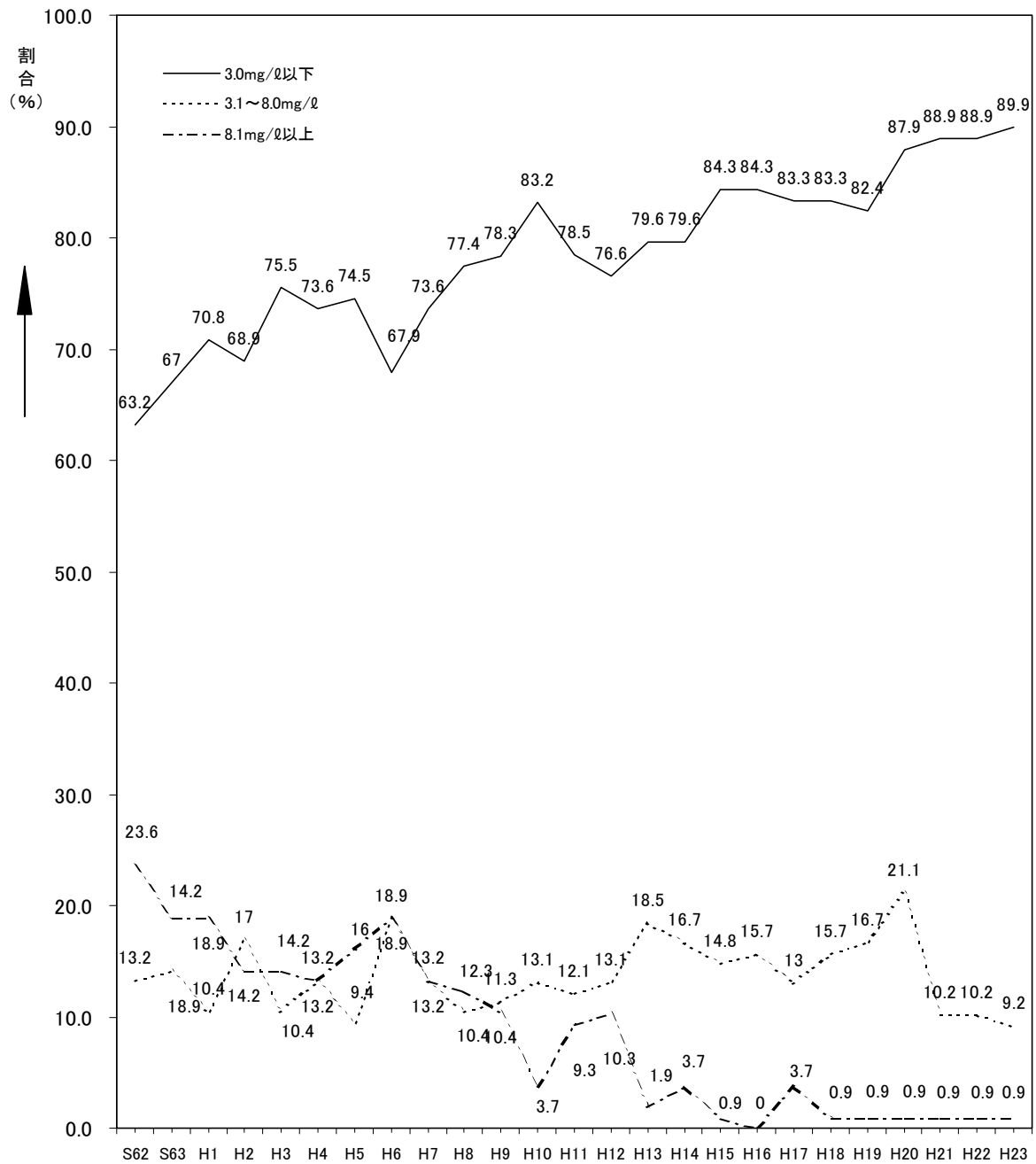
図-5.5 BOD75%値ランク別割合経年変化（109地点）
