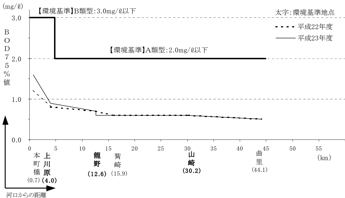
図-5.47 揖保川の水質縦断図（BOD75%値）
