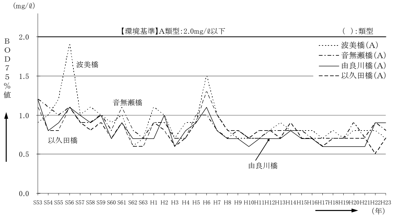
図-5.52 由良川水系（由良川）の環境基準地点の水質経年変化（BOD75%値）
