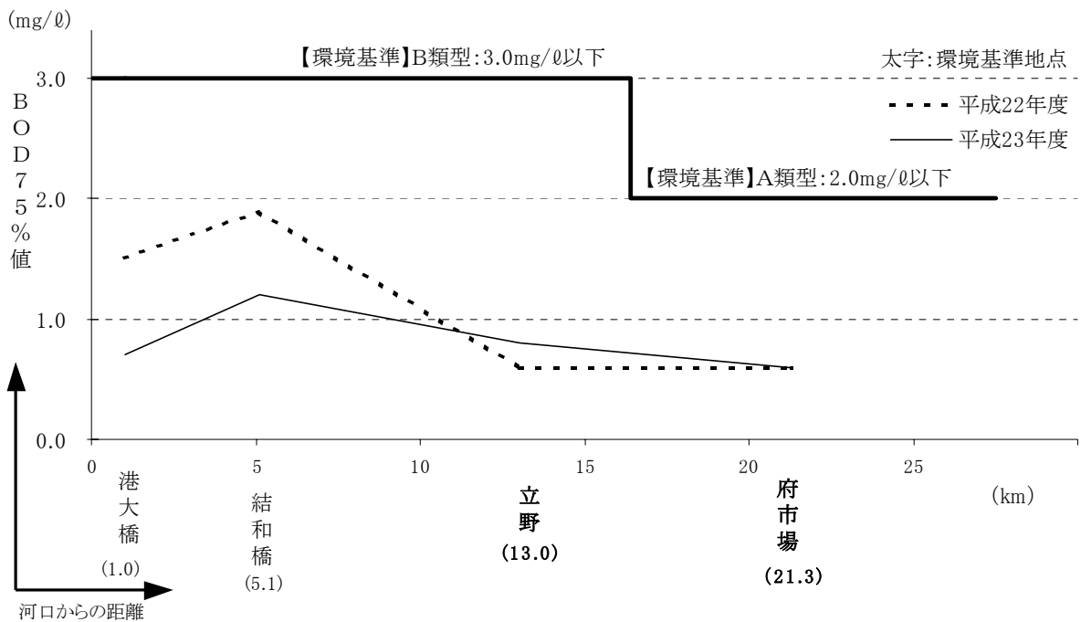
図-5.55 円山川の水質縦断図（BOD75%値）
