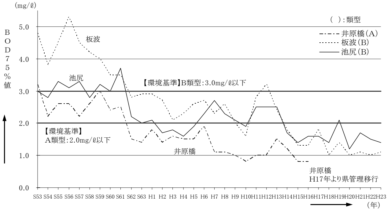
図-5.44 加古川水系の環境基準地点の水質経年変化（BOD75%値）
