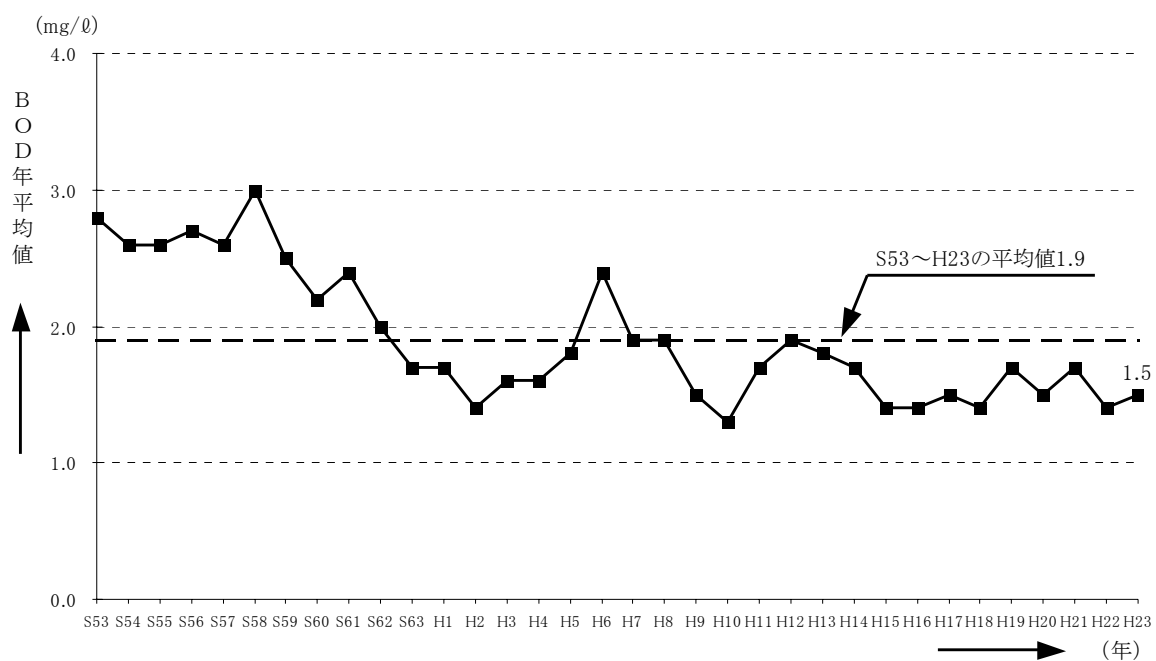
図-5.21 加古川の水質経年変化 (BOD年平均值)
