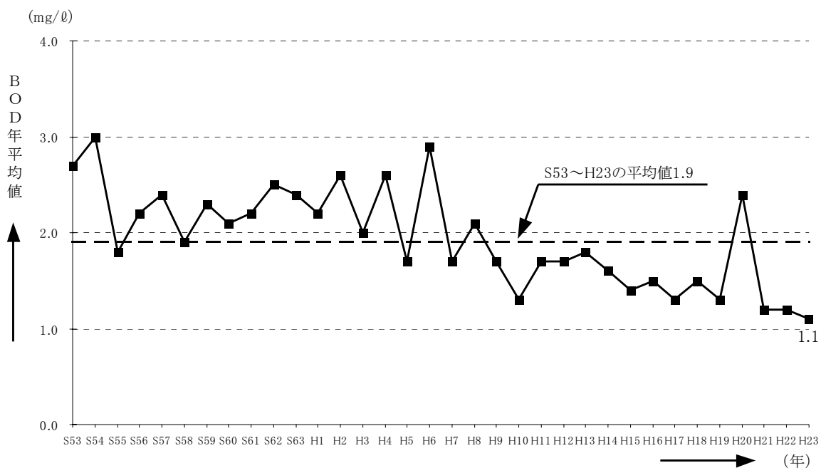
図-5.28 日野川の水質経年変化（BOD年平均值）
