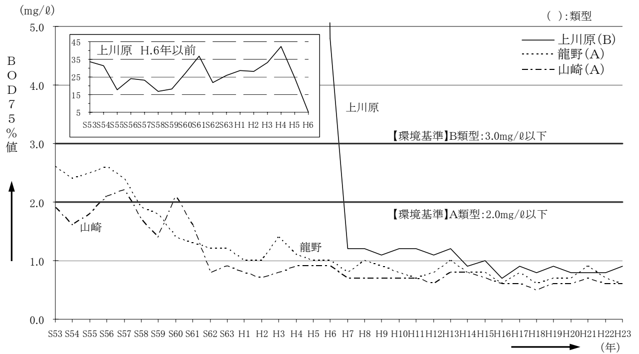
図-5.46 揖保川水系の環境基準地点の水質経年変化（BOD75%値）
