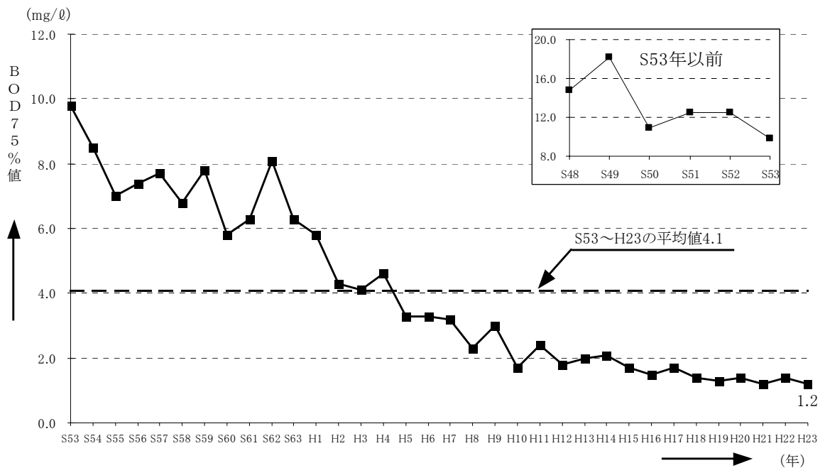
図-5.14 淀川水系桂川 宮前橋地点における水質の経年変化
