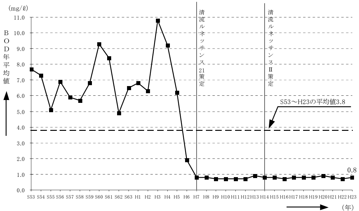
図-5.22 揖保川の水質経年変化（BOD年平均値）
