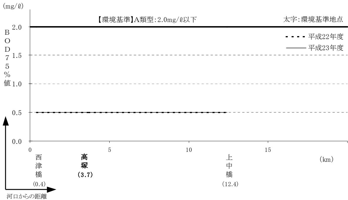
図-5.51 北川の水質縦断図（BOD75%値）
