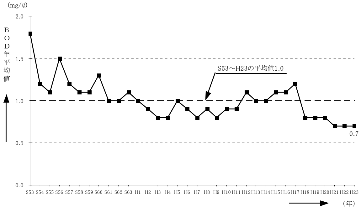
図-5.15 野洲川の水質経年変化 (BOD年平均値)
