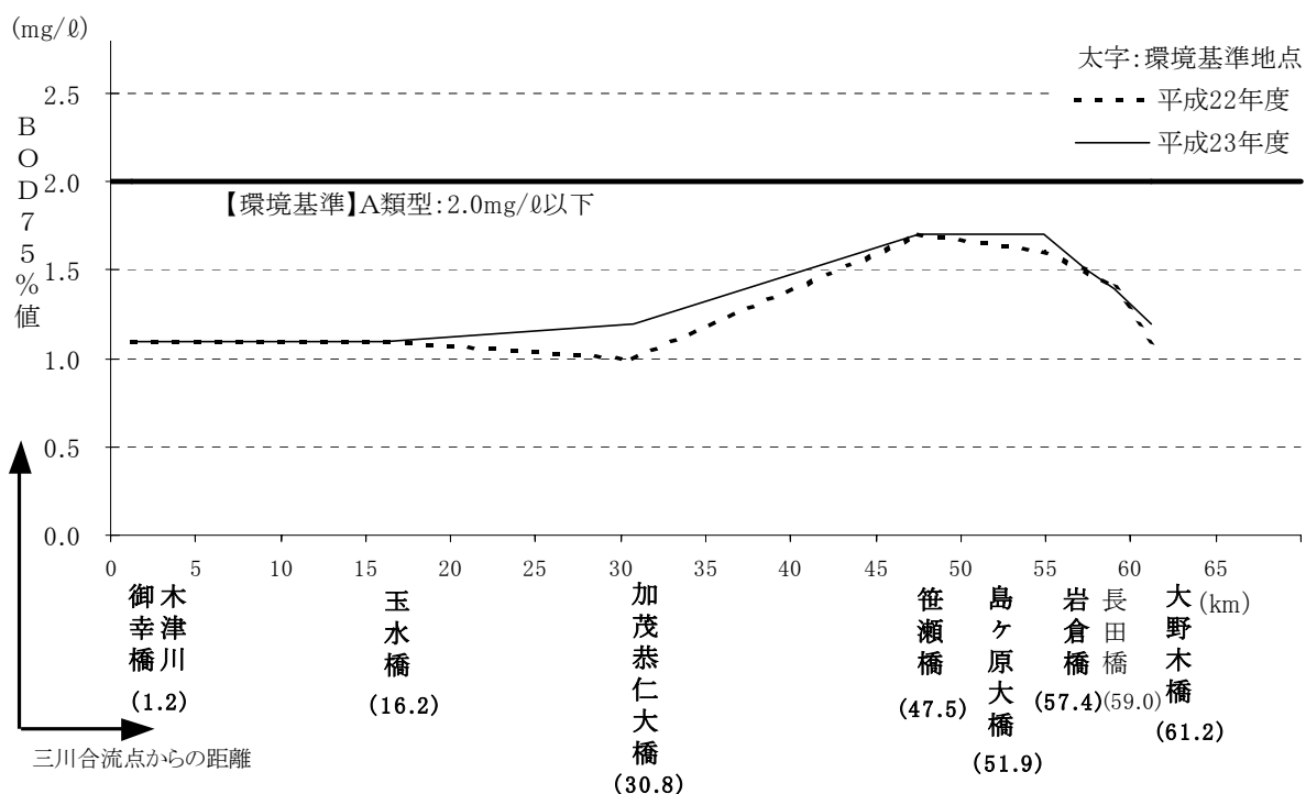
図-5.41 木津川の水質縦断図（BOD75%値）
