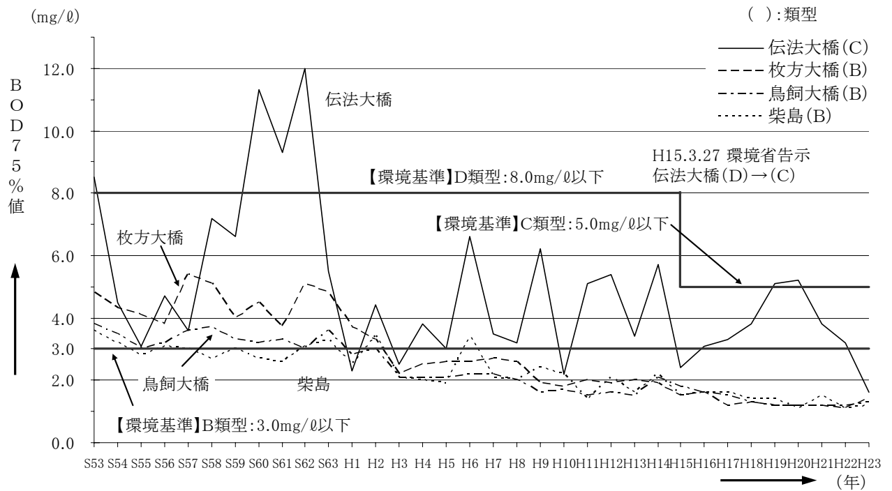
図-5.35 淀川水系（三川合流点下流）の環境基準地点の水質経年変化（BOD75%値）
