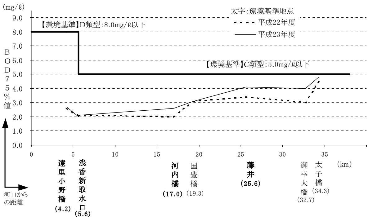
図-5.34 大和川の水質縦断図（BOD75%値）
