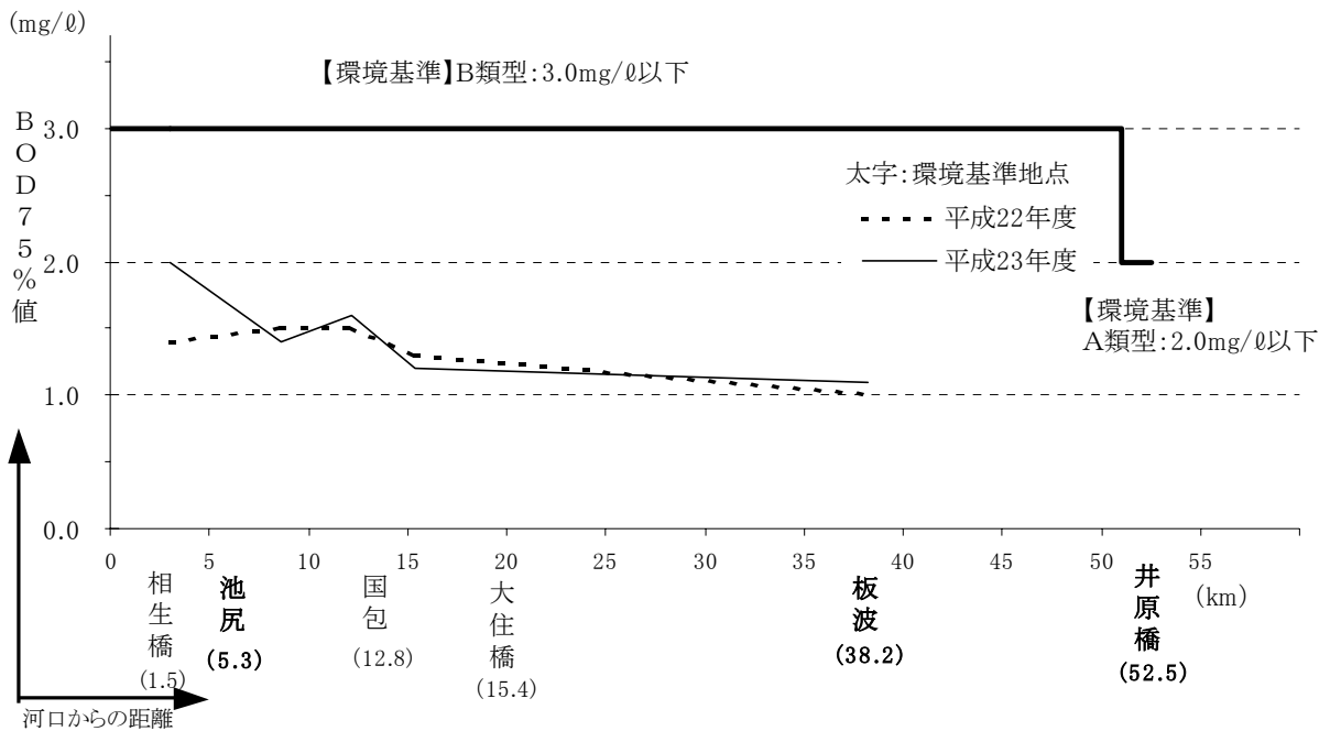
図-5.45 加古川の水質縦断図（BOD75%値）
