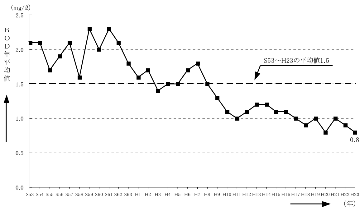
図-5.17 宇陀川の水質経年変化 (BOD年平均值)
