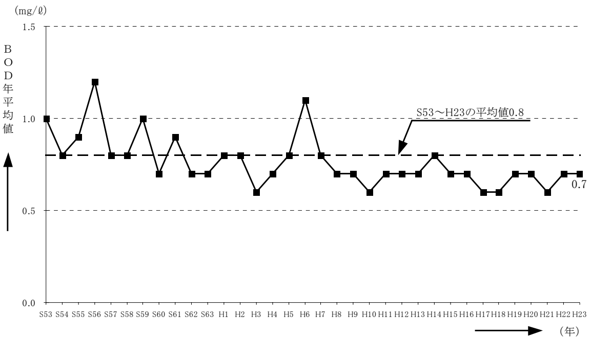
図-5.25 由良川の水質経年変化 (BOD年平均值)
