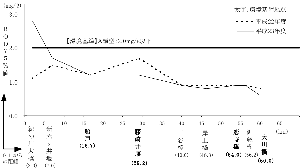
図-5.32 紀の川の水質縦断図（BOD75%値）
