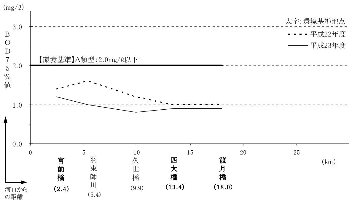
図-5.39 桂川の水質縦断図（BOD75%値）
