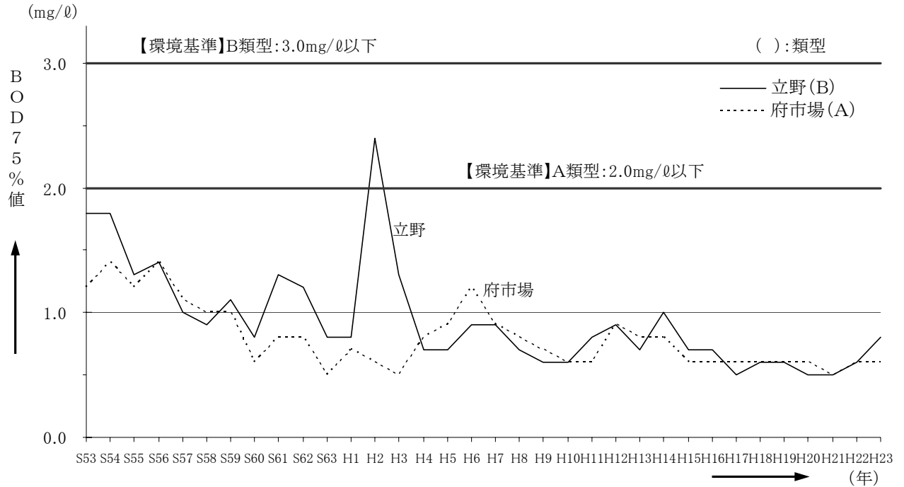
図-5.54 円山川水系の水質経年変化（BOD75%値）
