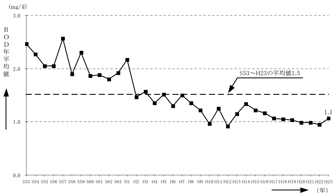
図-5.12 淀川本川（三川合流点上流）平均水質の経年変化
