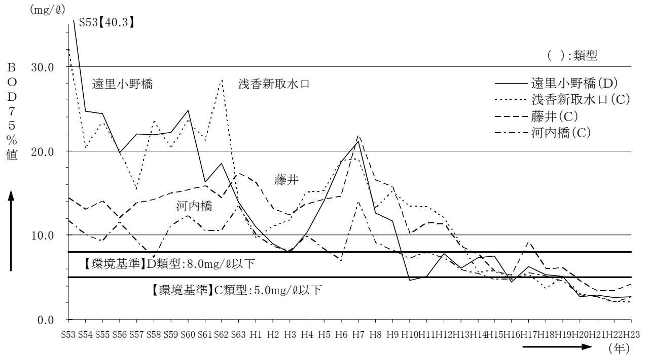
図-5.33 大和川水系（大和川）の環境基準地点の水質経年変化（BOD75%値）
