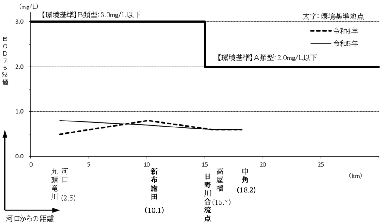
図-1.50 九頭竜川の水質縦断図（BOD75%値）
