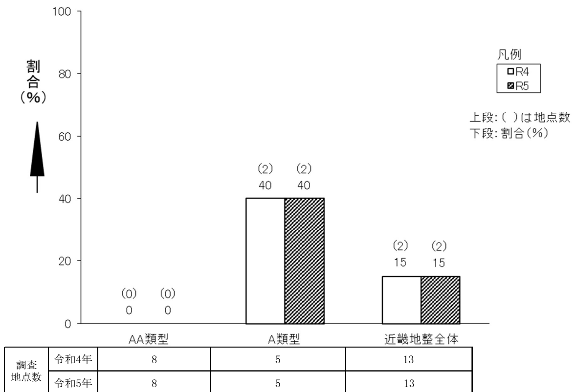
図-1.2 湖沼類型指定地点における類型別環境基準の満足状況 (令和4年、令和5年) (COD75%値)
