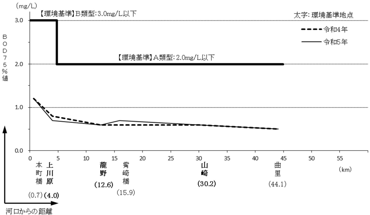
図-1.48 揖保川の水質縦断面図（BOD75%値）
