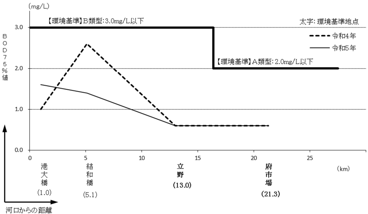
図-1.56 円山川の水質縦断図（BOD75%値）
