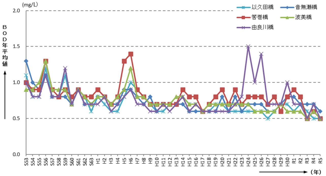
図一.26 由良川の水質経年変化（BOD年平均値）
