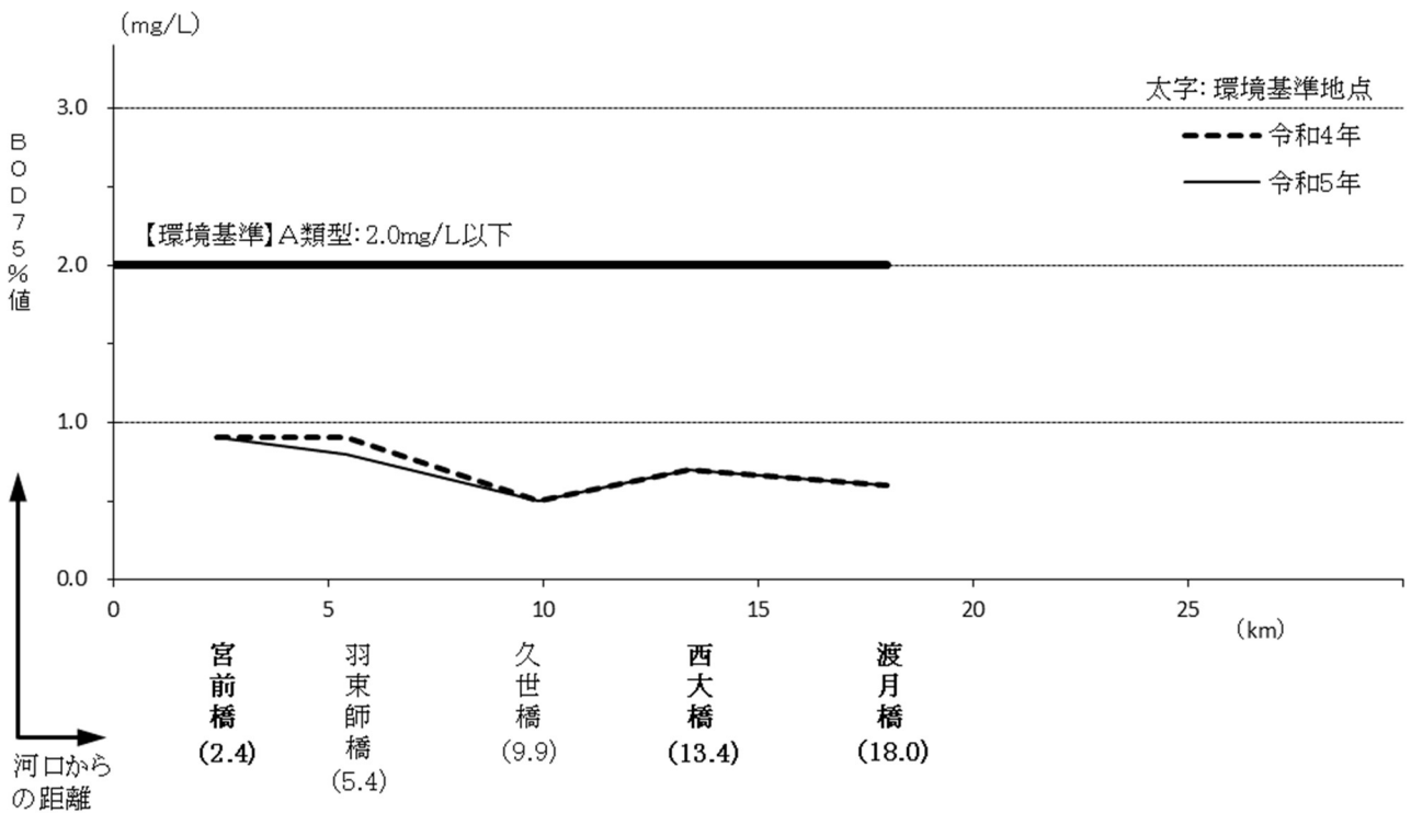
図-1.40 桂川の水質縦断図（BOD75%値）
