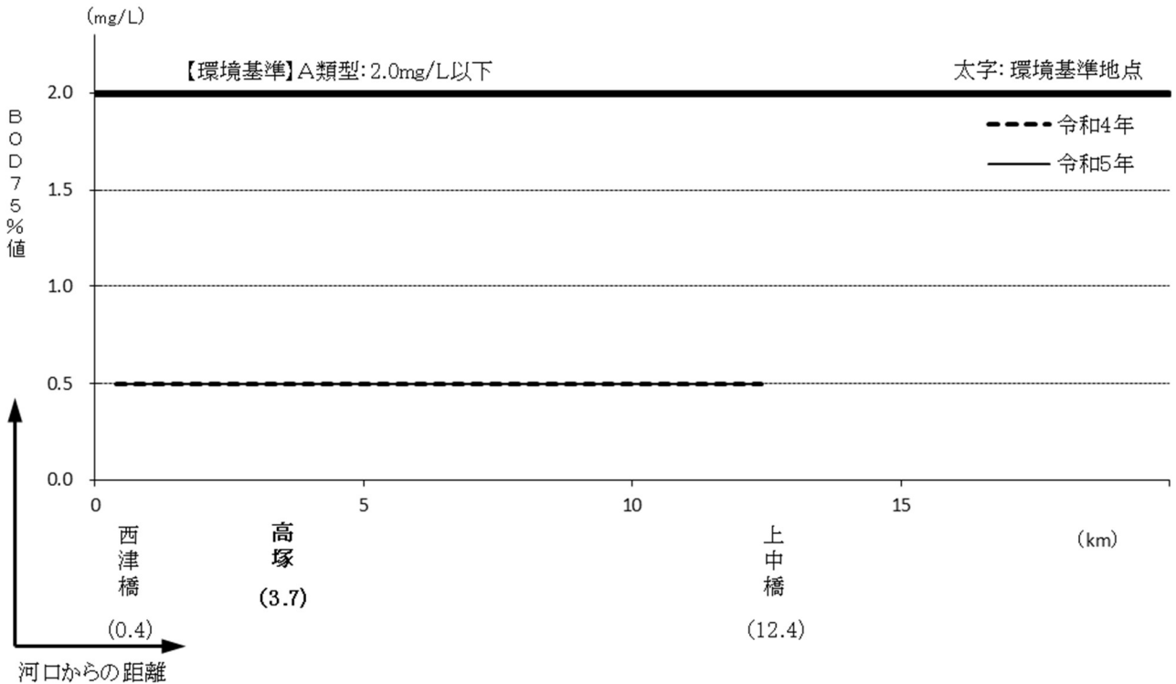
図-1.52 北川の水質縦断面図（BOD75%値）
