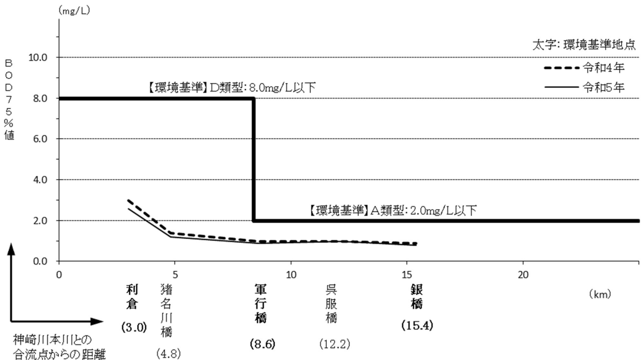
図-1.44 猪名川の水質縦断図（BOD75%値）
