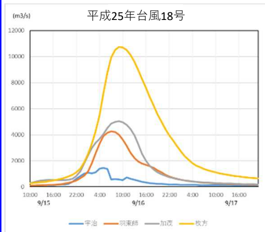
【各地点の流量ハイドログラフ】
