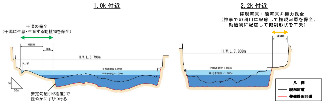
図-4.2 河道掘削イメージ (横断面)
