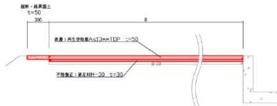
標準断面図
