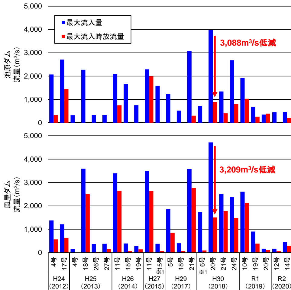
池原・風屋ダムにおける運用実績
