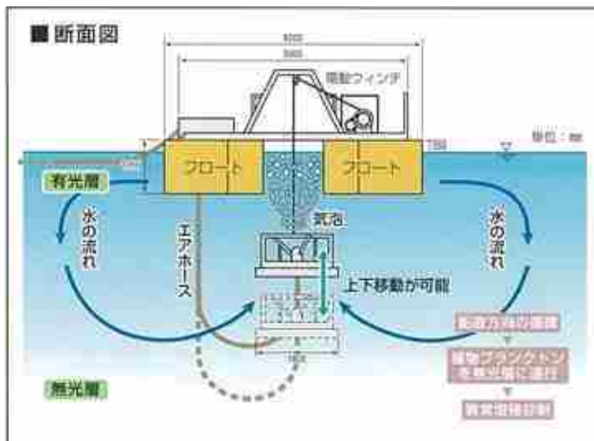
図 5.6.1-2 曝気循環設備
