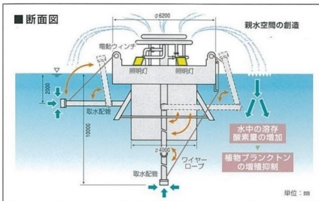
図 5.6.1-3 分画フェンス・噴水
