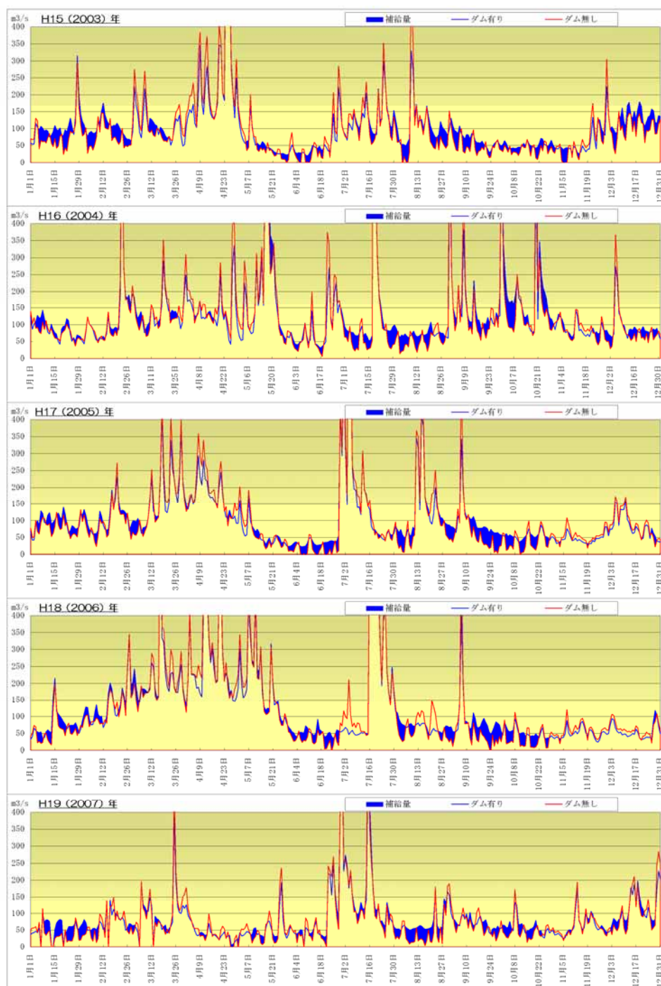
図 3.4 - 2 中角地点における九頭竜ダムからの発電放流の有無による流況の比較 (近5カ年(平成15年~平成19年))
