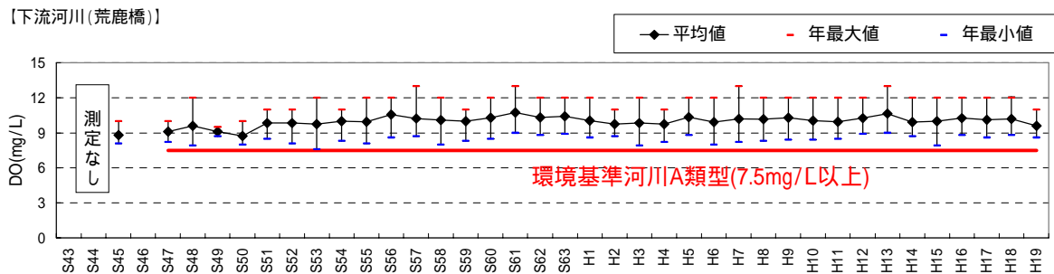
図 5.3-10(3) 各地点における流入河川、放流水及び下流河川の水質の経年変化 (DO) 河川的环境基準値 (AA 類型・A 類型: 同じ) をグラフ中に表示している。
