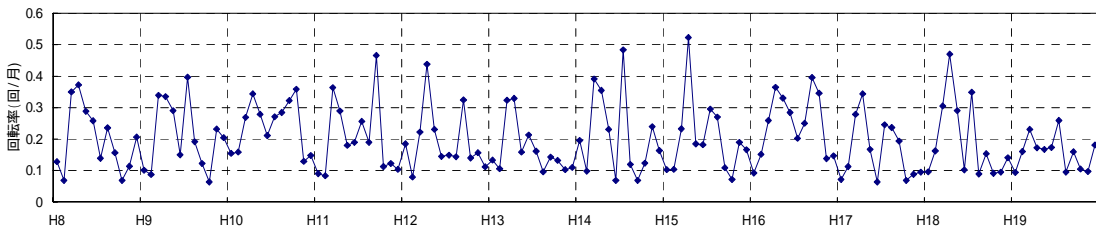
図 5.5-16(1) 貯水池表層の水温・月回転率と植物プランクトン(細胞数)の関係 (H8~H19)
