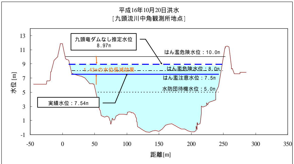
図 2.4 - 6 水位低減効果 (平成 16 年 10 月 20 日洪水)
