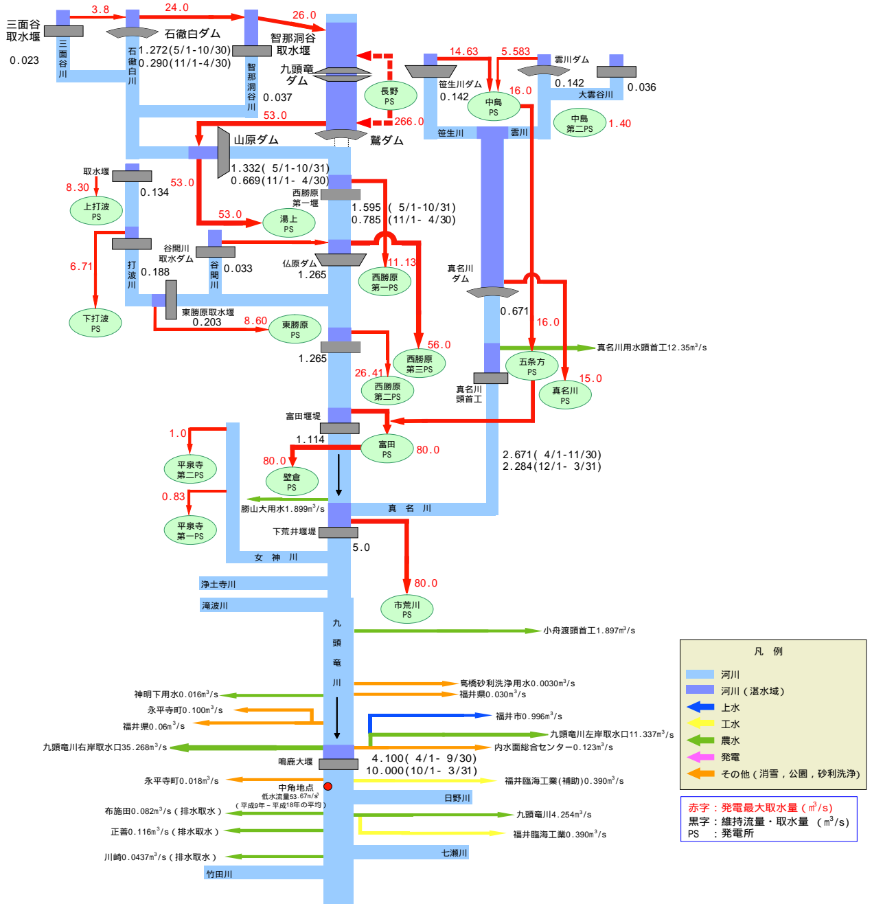
図 1.1 - 15 水利用の現況模式図
