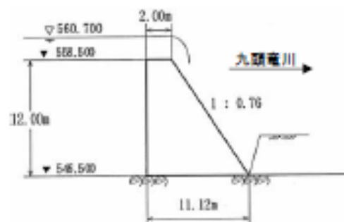
図 2-3 水質対策堰堤模式図
