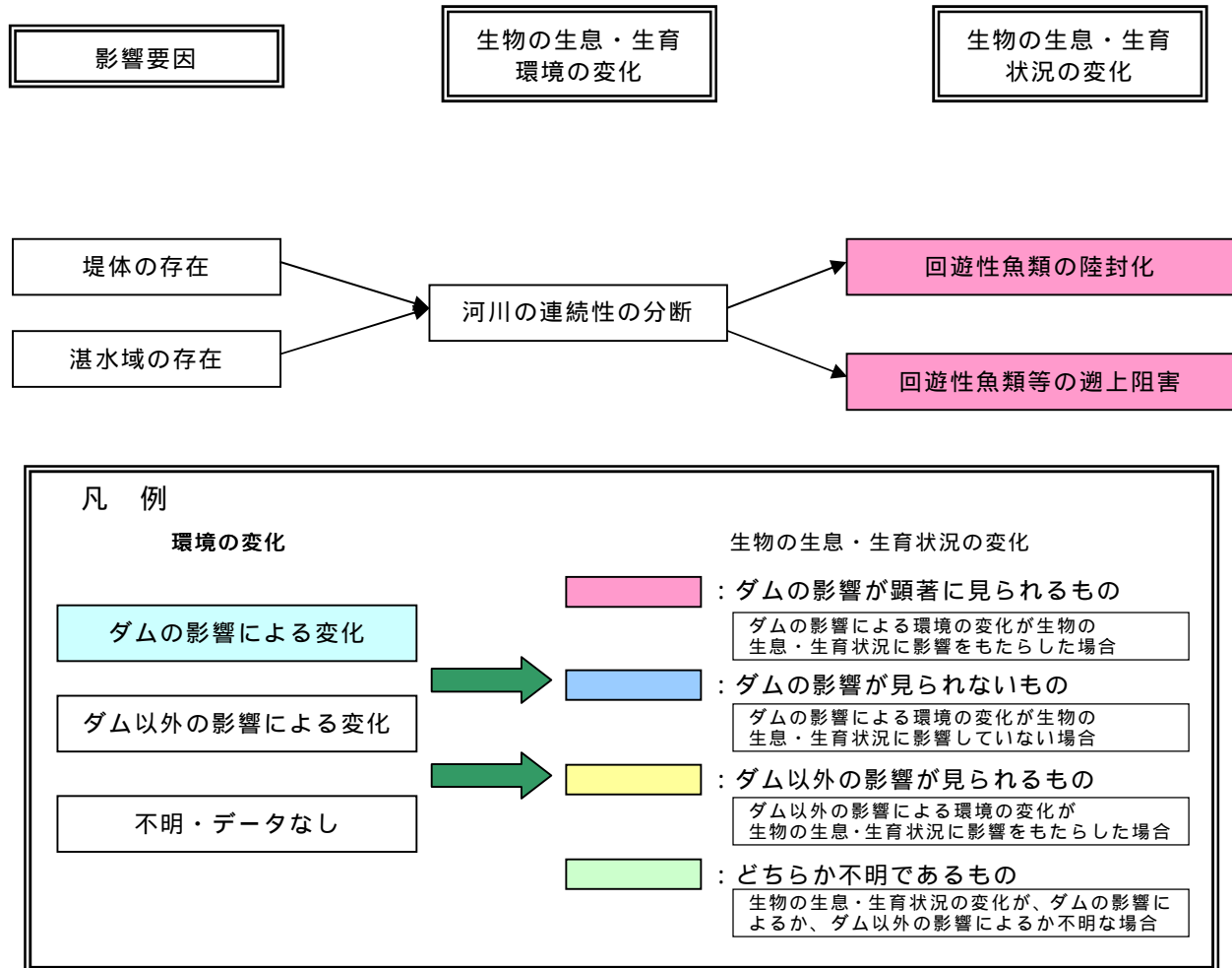
図 6.3-51 連続性の観点からみた生物の変化に対する影響の検証結果
