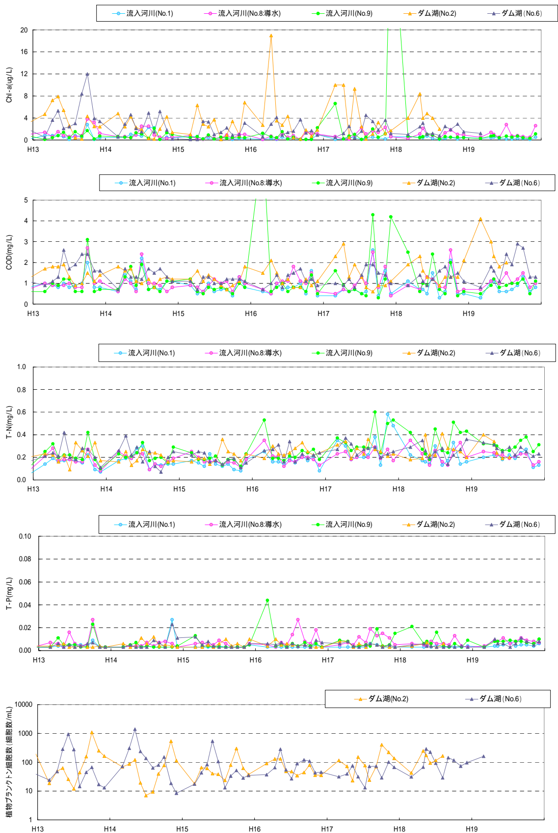
図 5.5-15(5) 富栄養化評価関連項目の経月変化(H13～H19)
