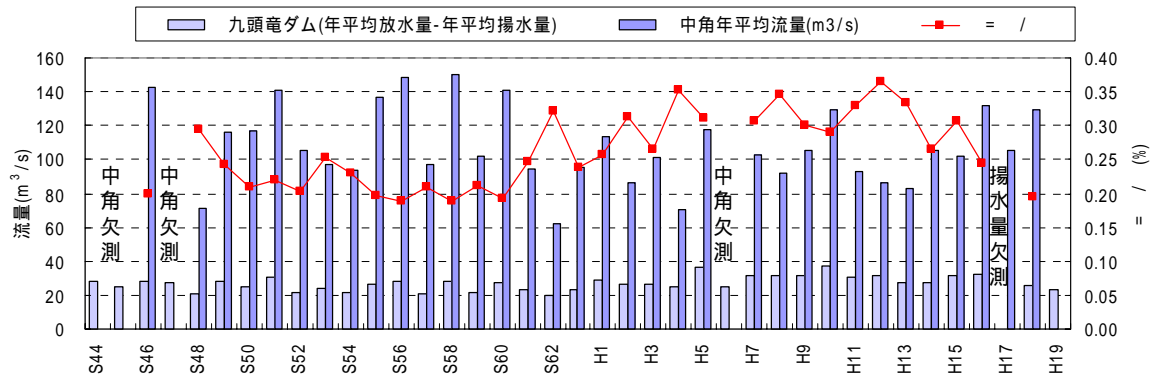
図 5.3-7 中角地点年平均流量と九頭竜ダム(年平均放流量 - 年平均揚水量)の比較
