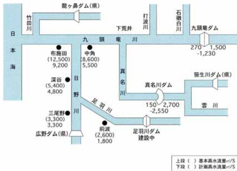
図 2.3 - 1 流量配分図
