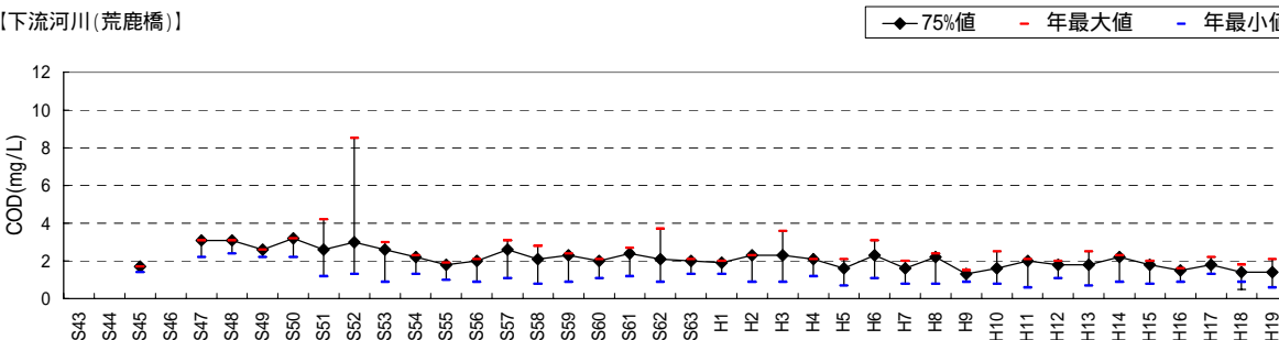
図 5.3-10(7) 各地点における流入河川、放流水及び下流河川の水質の経年変化 (COD)
