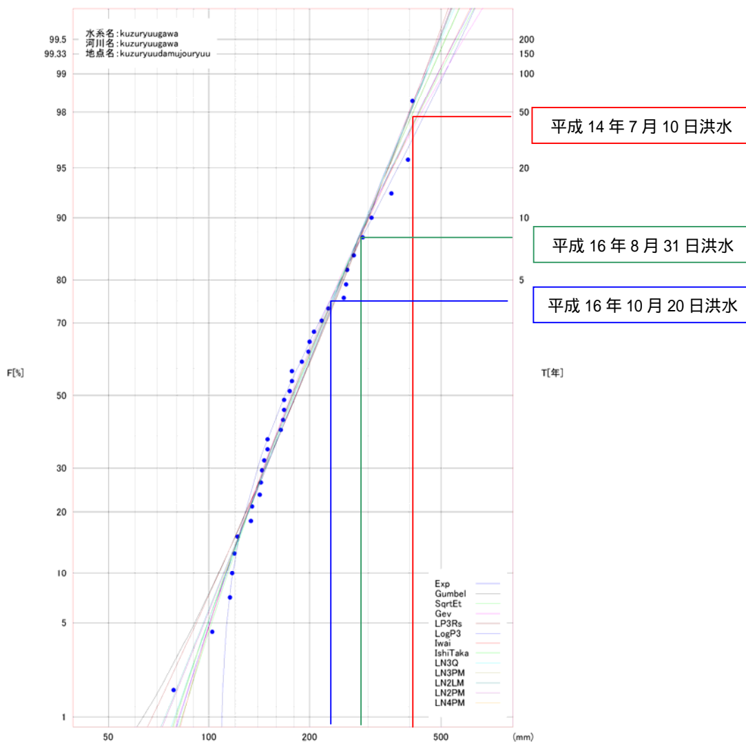
図2.3-5 九頭竜ダム地点における雨量確率評価
