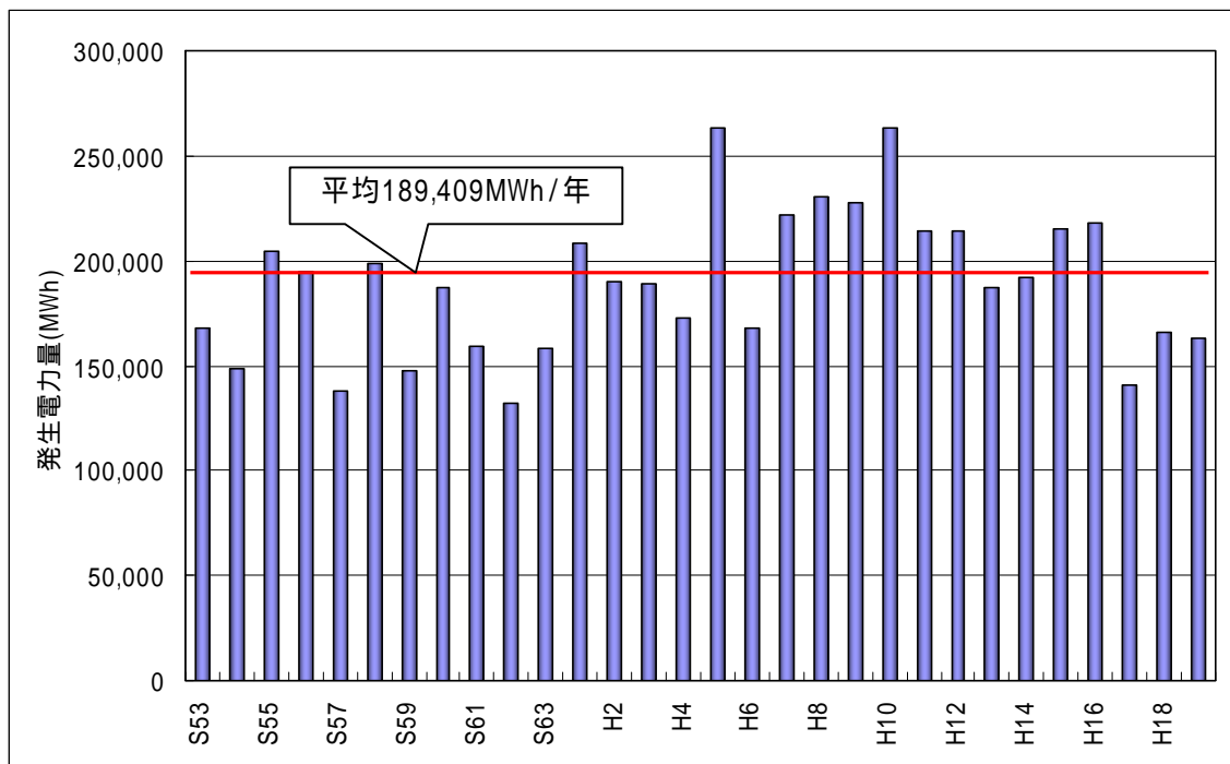
図 3.3 - 3 発電実績
