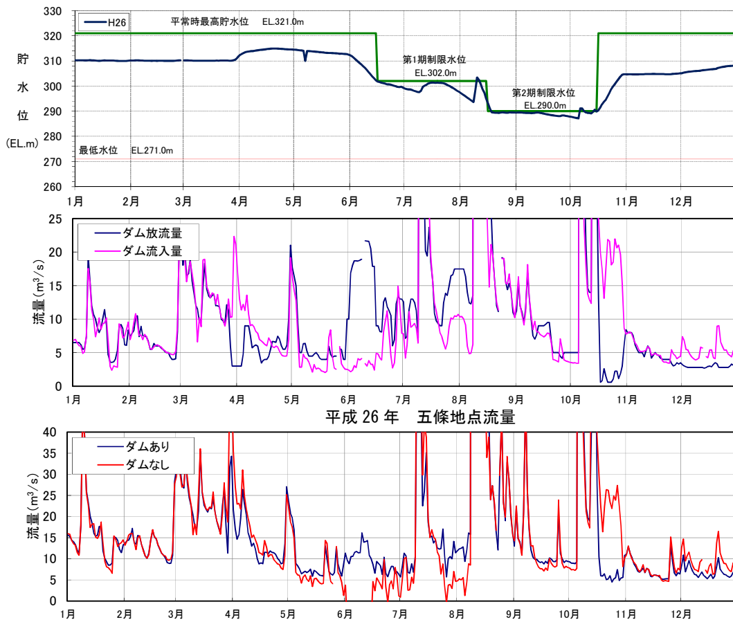
図 3.4.1-4 平成 26 年の大滝ダムの貯水位・流入量・放流量、五條地点の流量変化
