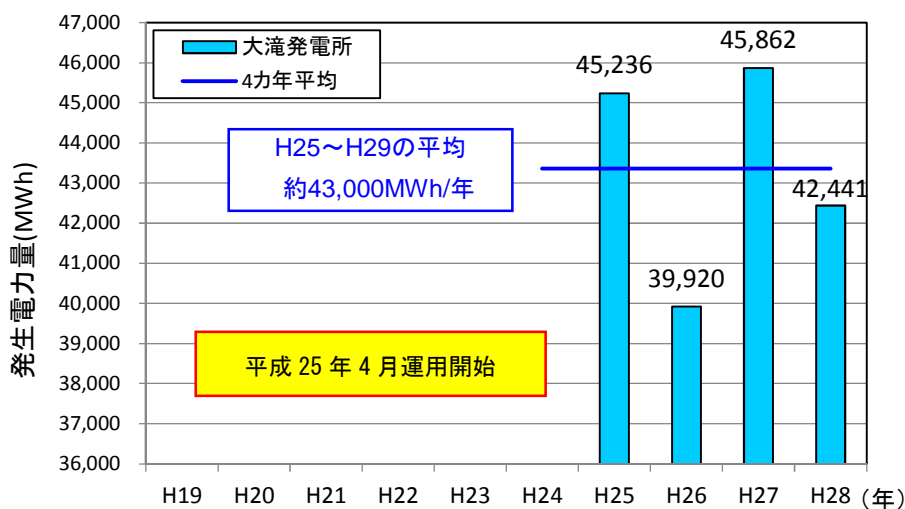
図 3.4.3-1 大滝ダムの発電実績
