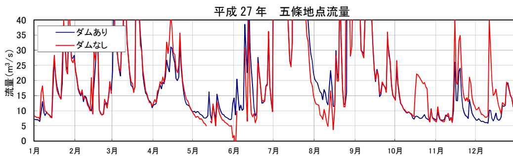
図 3.4.1-5 平成 27 年の大滝ダムの貯水位・流入量・放流量、五條地点の流量変化
