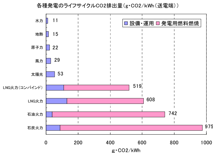
図 3.4.4-1 各種発電のライフサイクル CO 2 排出量
