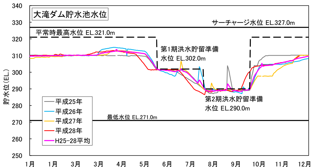
図 1.4.1-1 貯水容量図
