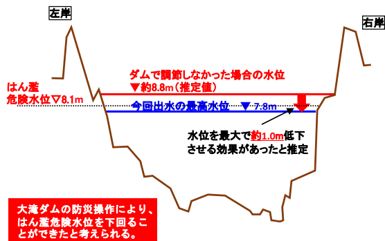
図 2.4.1-1 洪水調節効果図 (平成 25 年 9 月台風 18 号)
