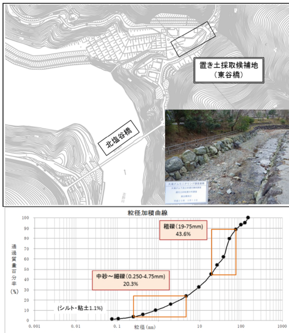
図 6.4.2-1 還元土砂採取候補地と河床の粒度
