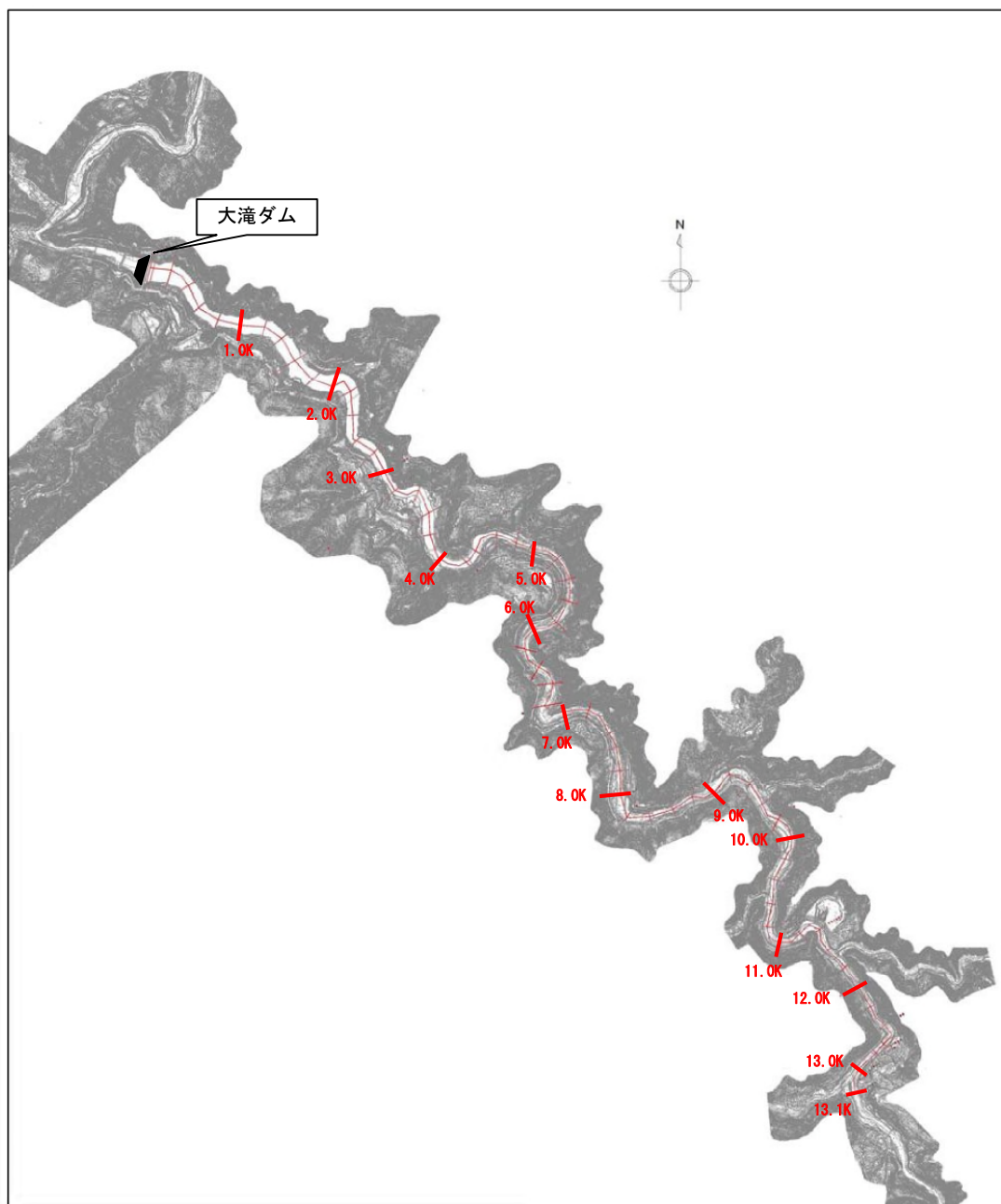
図 4.2.2-1 測線位置
