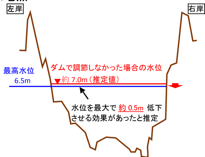
図 2.4.1-2 洪水調節効果評価図 (平成 26 年 8 月台風 11 号)
