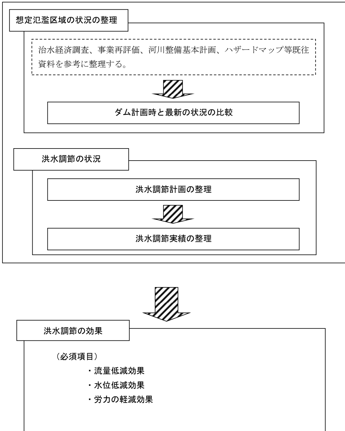
図 2.1.2-1 評価手順
