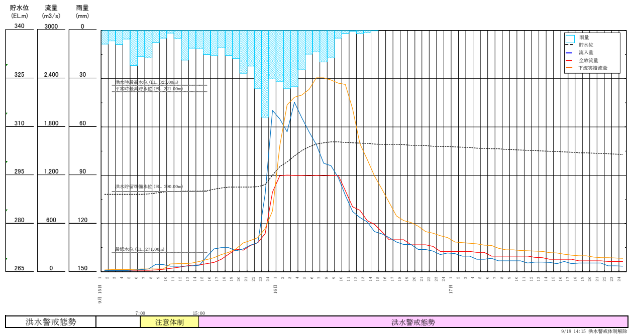
図 2.3.3-1 大滝ダム洪水調節実績図(平成25年9月台風18号)
