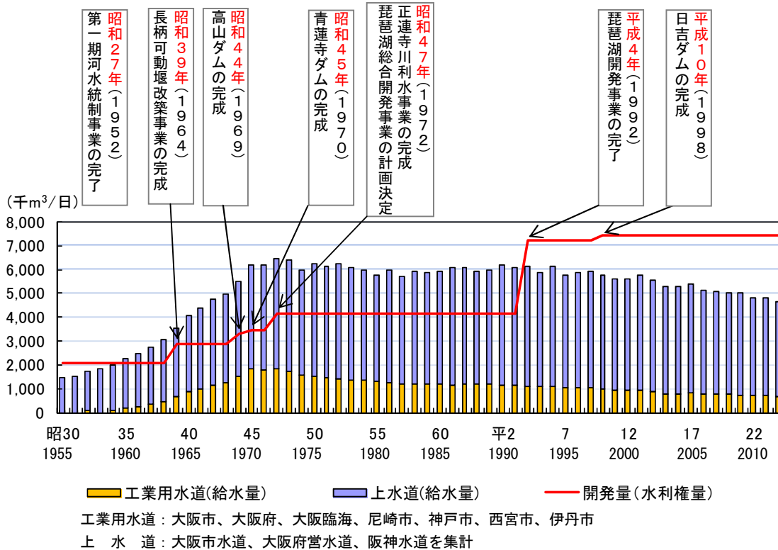
図 3.4-9 下流府県への都市用水給水量の推移※
