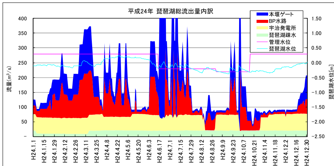
図 3.3-9 琵琶湖水位及び流出量内訳 (2012年(平成24年))
