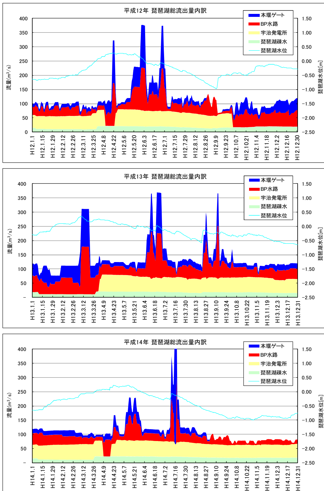
図 3.3-5 琵琶湖水位及び流出量内訳 (2000年(平成12年)～2002年(平成14年))
