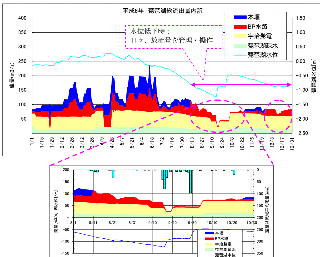
図 3.4-6 琵琶湖水位低下時におけるバイパス水路による放流量の微調整(1994年(平成6年))
