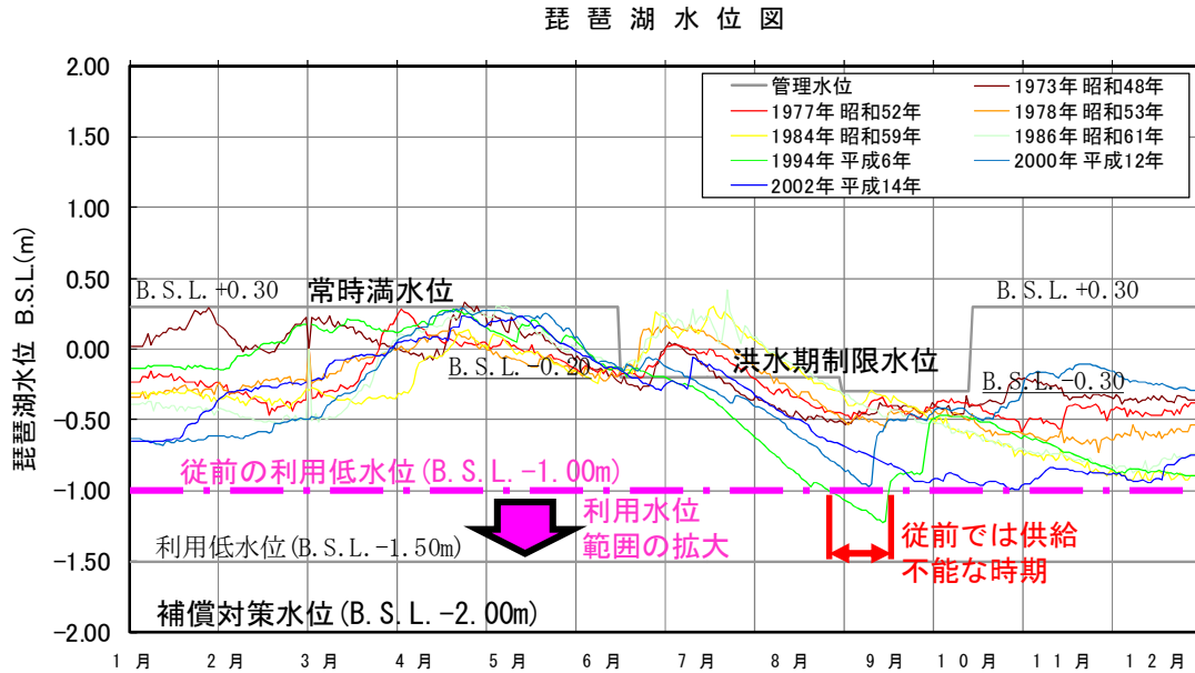
図 3.4-5 利用水位範囲の拡大による効果
