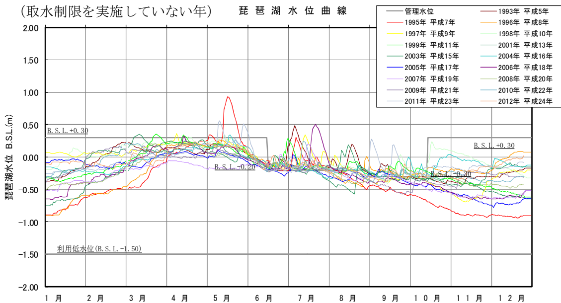
図 3.4-2(1) 琵琶湖水位の状況(1993年(平成5年)~2012年(平成24年)のうち、取水制限を実施した1994年(平成6年)、2000年(平成12年)、2002年(平成14年)を除く)
