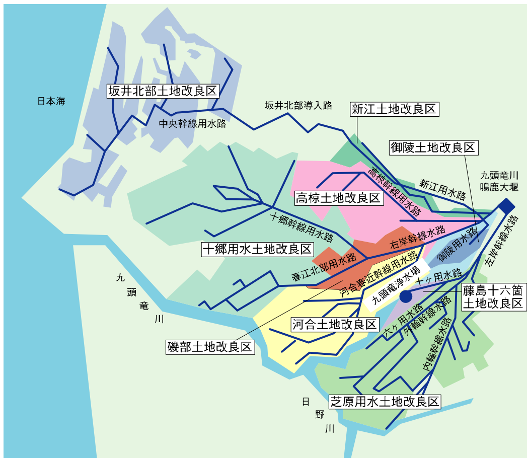
図 1.2-4 鳴鹿大堰かんがい区域
