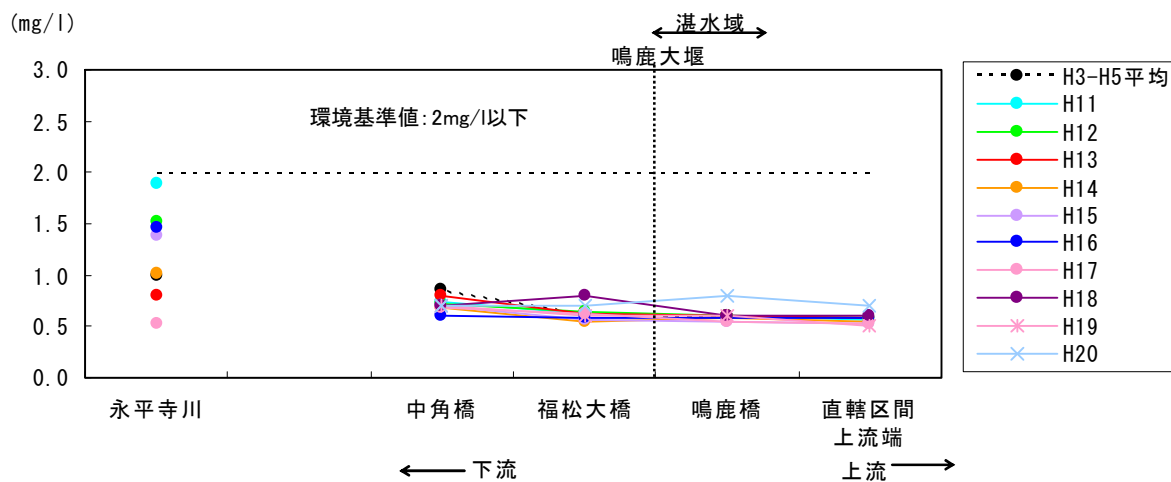
図 5.5-17 鳴鹿大堰年平均BODの縦断変化
