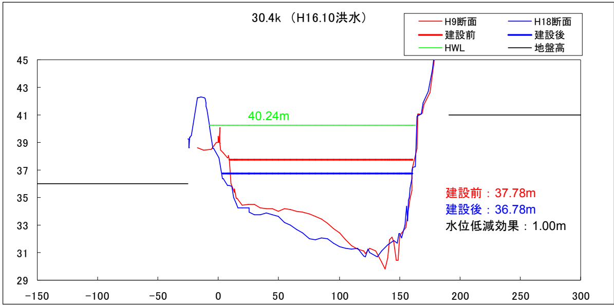
図 2.4-6 (2) H16.10洪水水位低減効果
