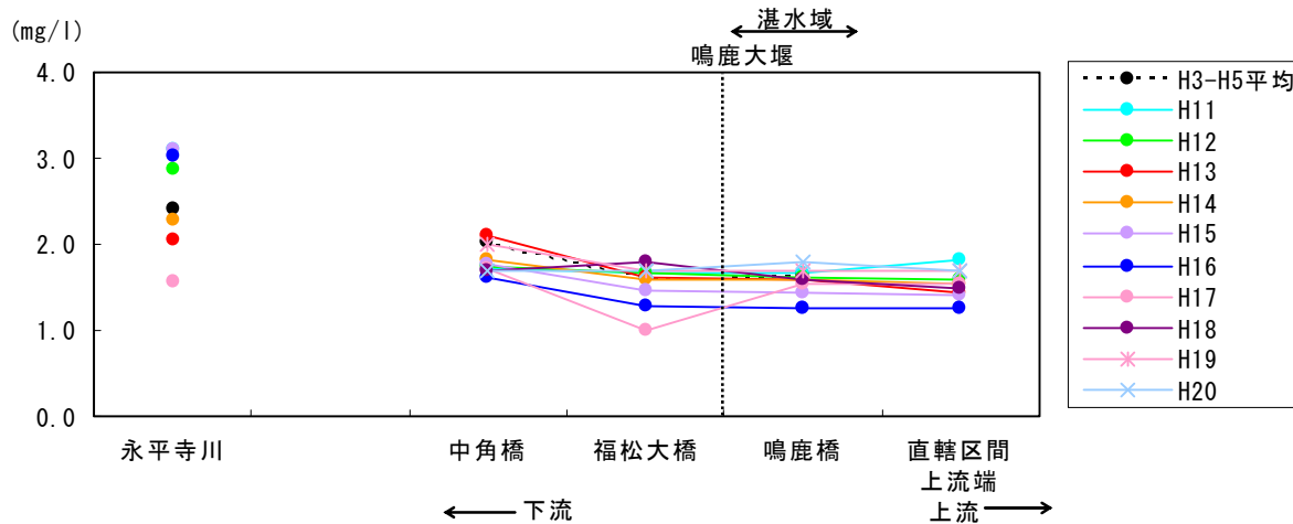
図 5.5-18 鳴鹿大堰年平均CODの縦断変化
