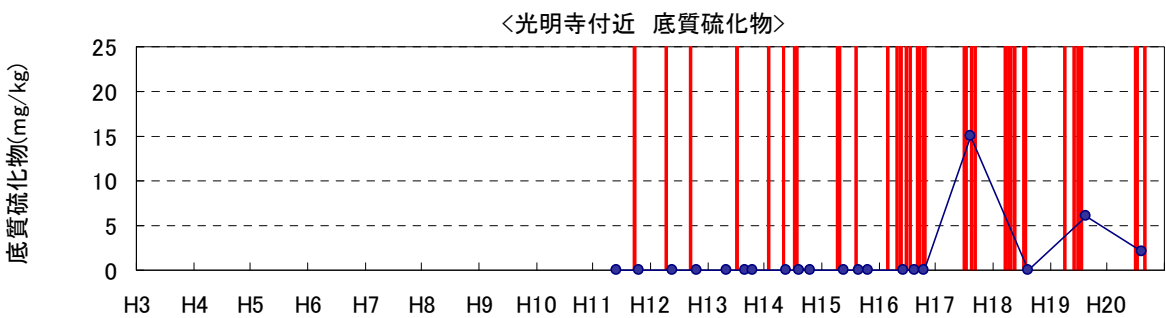
図 5.3-14 (1) 底質濃度の経年変化 (光明寺付近)
