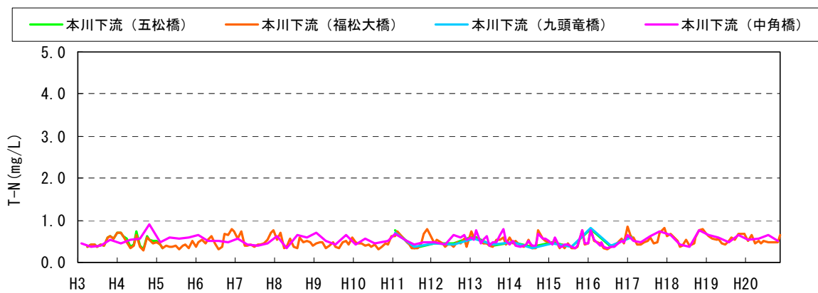
図 5.3-8 (8) 流入・湛水域・下流T-Nの経月変化
