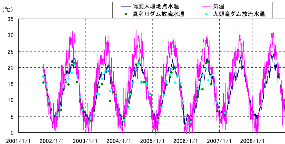
図 5.5-7 鳴鹿大堰地点における日平均水温と日平均気温の関係
