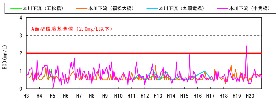
図 5.3-8 (6) 流入・湛水域・下流BODの経月変化
