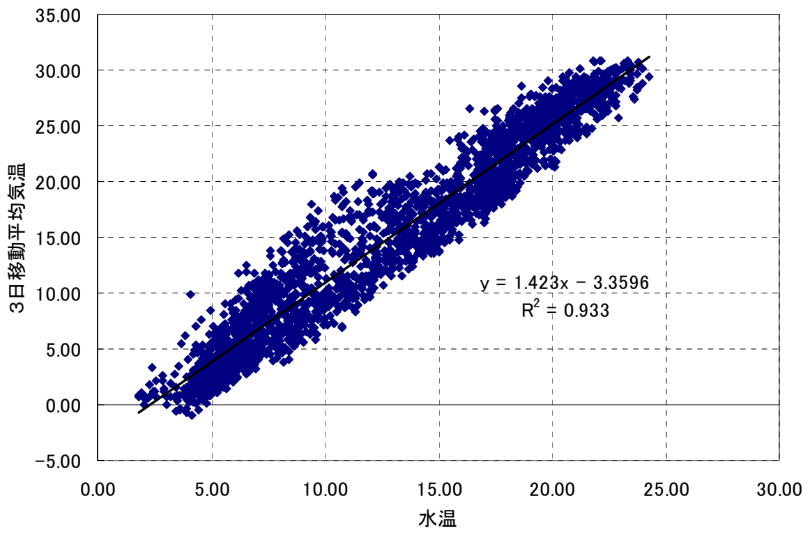
図 5.5-9 日平均水温と3日移動平均気温の相関
