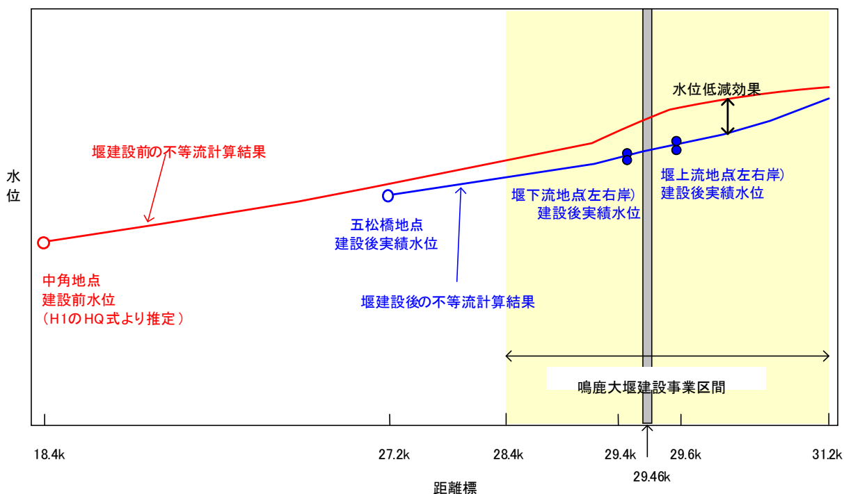
図 2.4-2 水位低減効果算定の模式図
