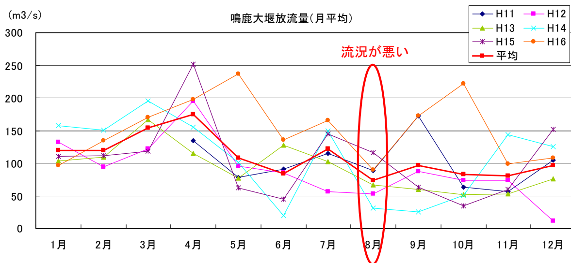
図 5.5-22 鳴鹿大堰における月平均放流量
