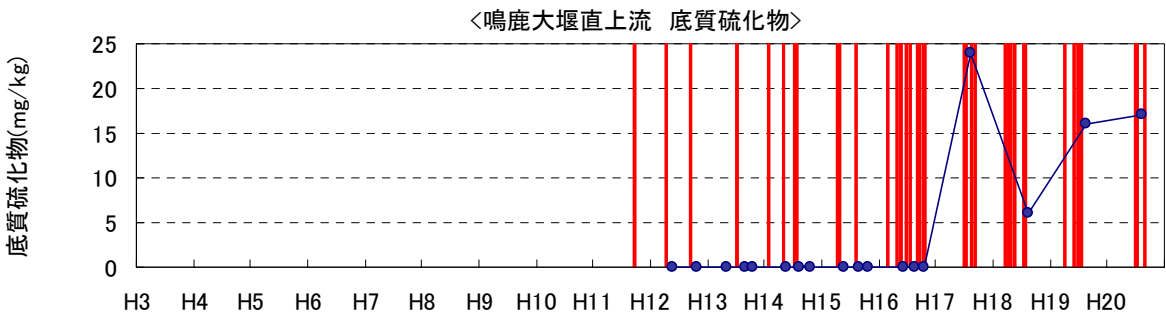
図 5.5-12 底質濃度の経年変化 (鳴鹿大堰直上流)
