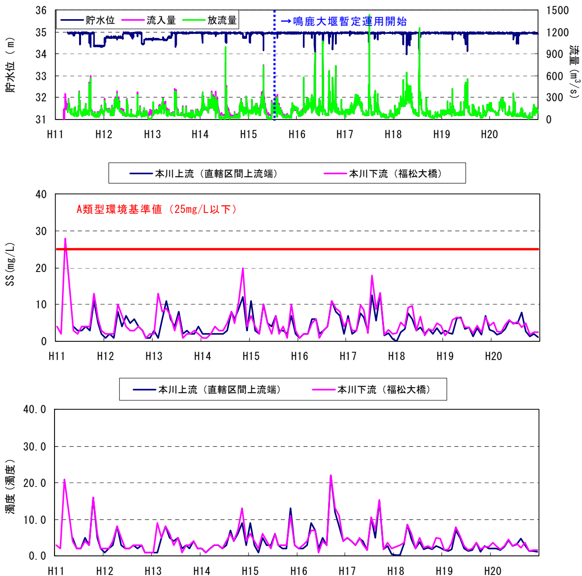
図 5.5-10 流入河川と下流河川のSSと濁度の経年変化
