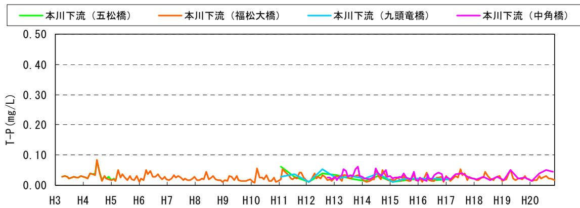
図 5.3-8 (9) 流入・湛水域・下流T-Pの経月変化
