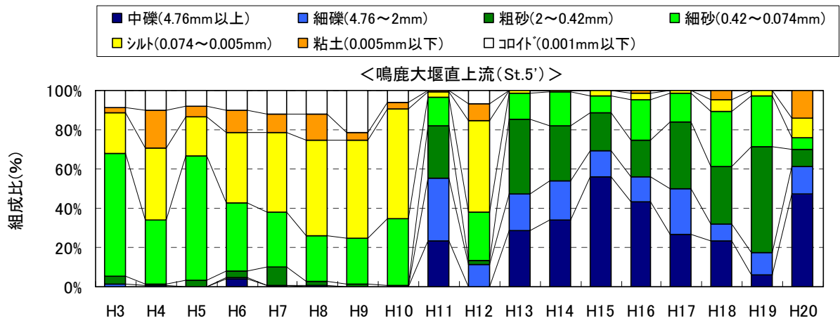
図 5.5-13 底質粒度組成の経年変化 (鳴鹿大堰直上流)
