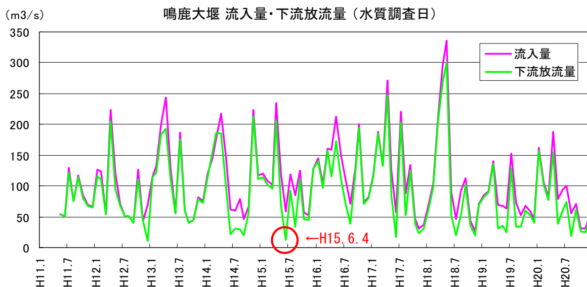
図 5.5-26 鳴鹿大堰における水質調査日の流入量・下流放流量
