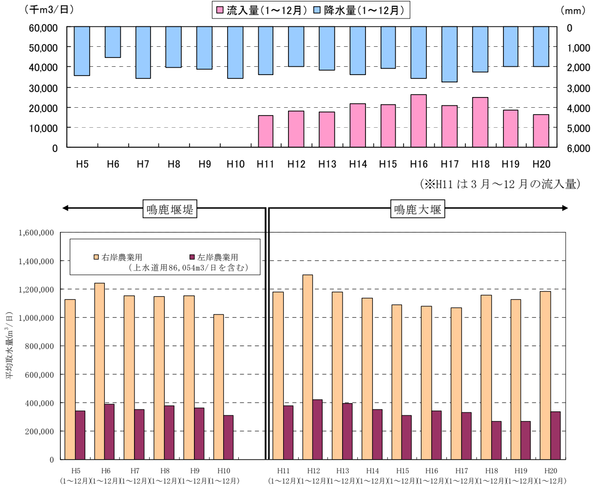
図 3.2-1 各年の取水状況
