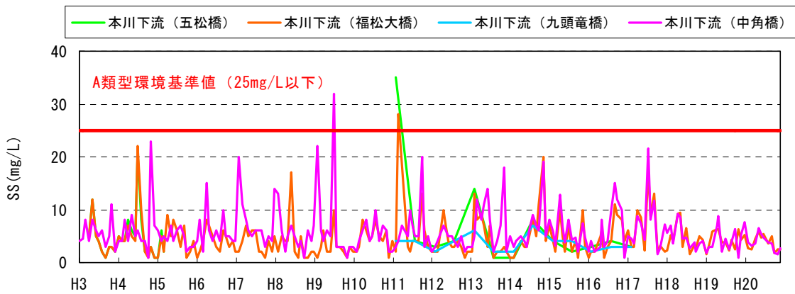
図 5.3-8 (2) 流入・湛水域・下流SSの経月変化
