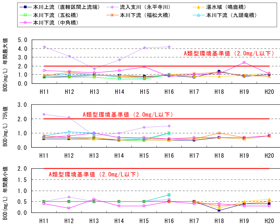
図 5.5-2 流入河川、湛水域および下流河川のBOD
