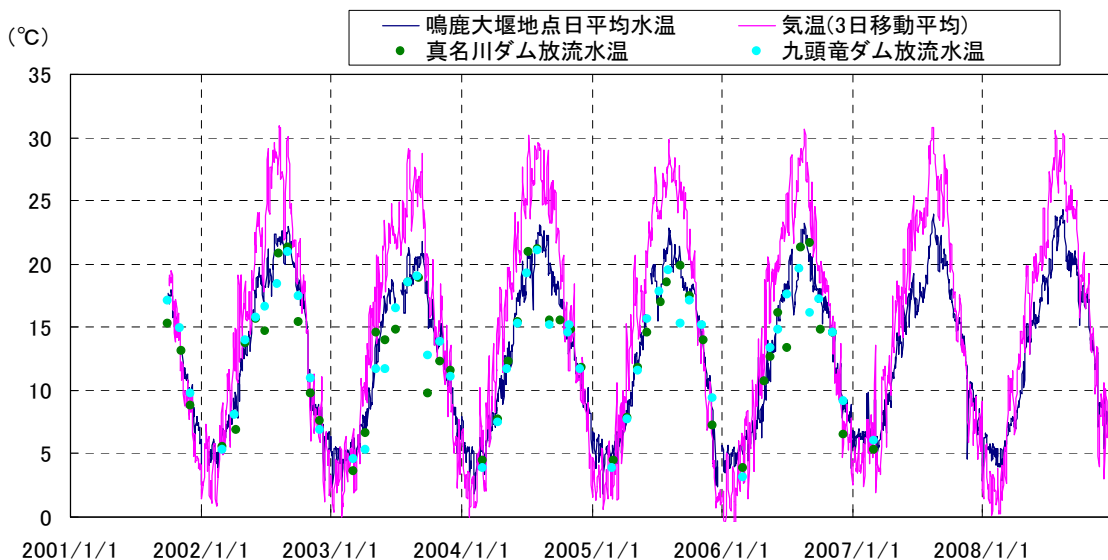
図 5.5-8 鳴鹿大堰地点における日平均水温と3日移動平均気温の関係
