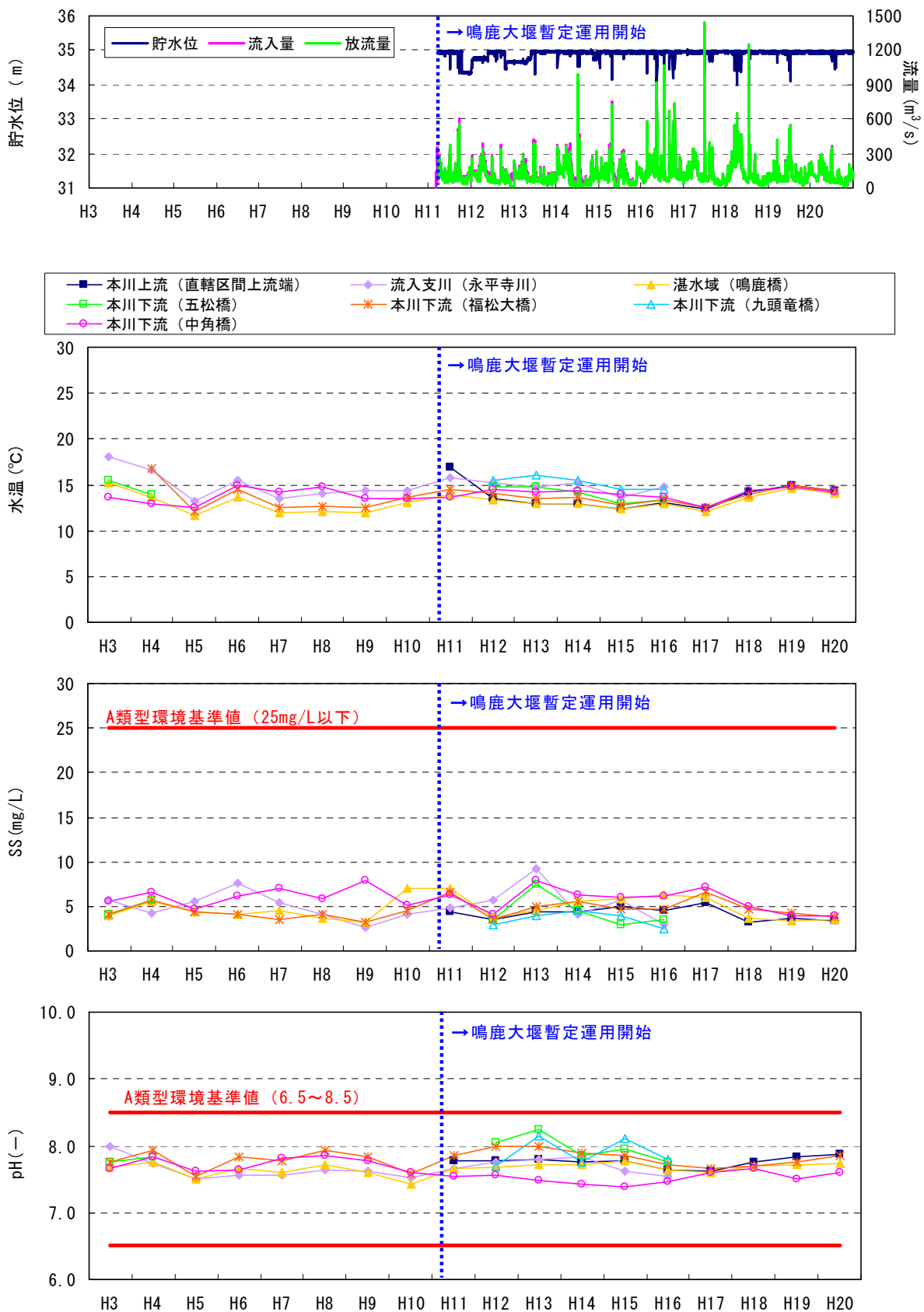
図 5.3-6 (1) 流入・湛水域・下流水質の経年変化
