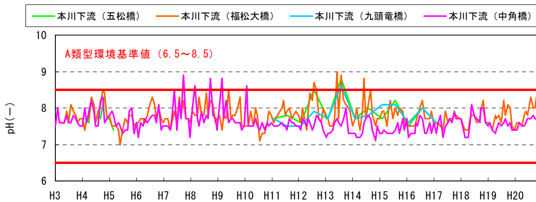
図 5.3-8 (3) 流入・湛水域・下流pHの経月変化
