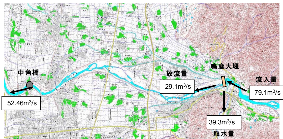
図 5.5-23 平成14年8月7日の流況
