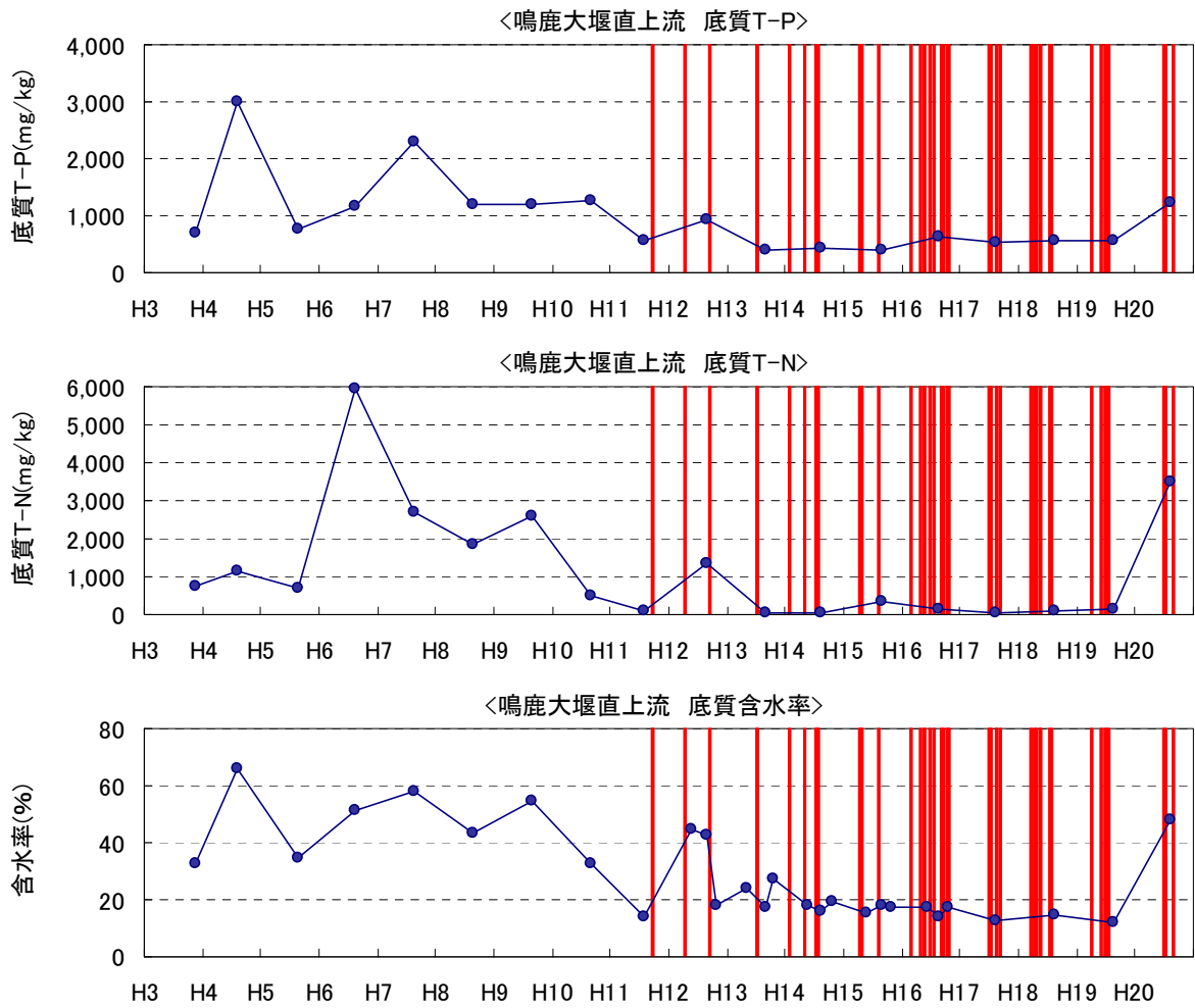
図 5.5-12 (2) 底質濃度の経年変化 (鳴鹿大堰直上流)
