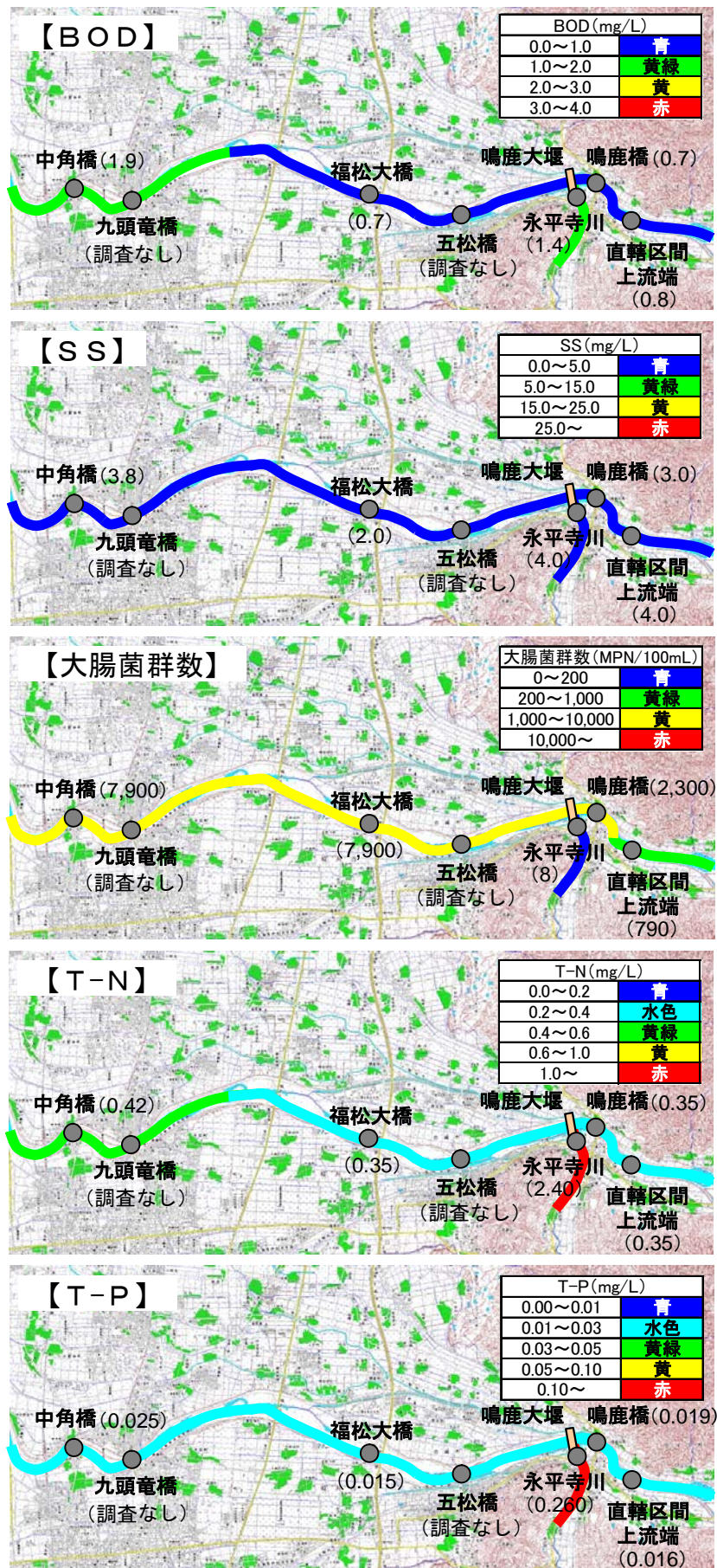
図 5.5-28 平成15年6月4日の水質縦断変化図
