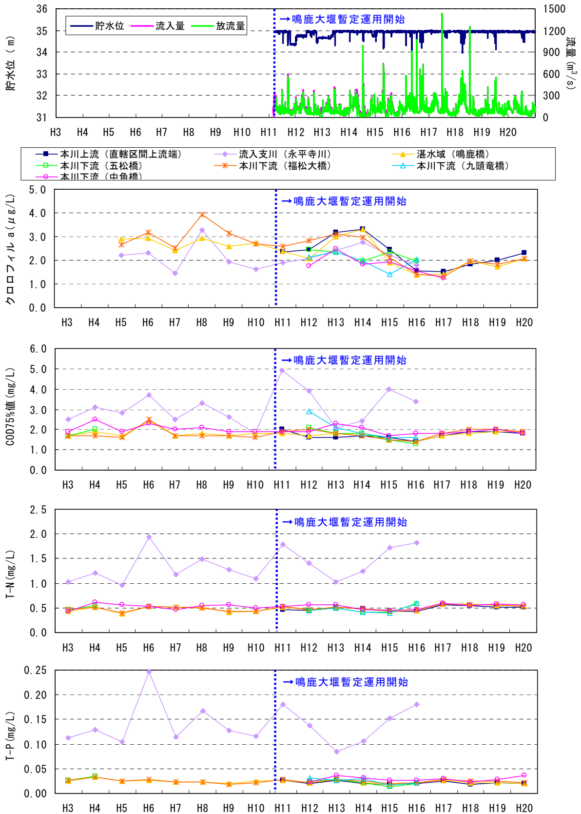
図 5.5-11 富栄養化評価関連項目の経年変化
