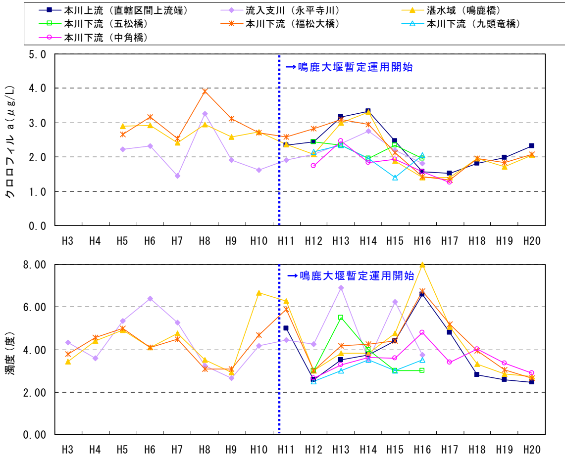
図 5.3-6 (4) 流入・湛水域・下流水質の経年変化
