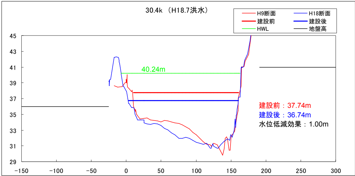
図 2.4-8 (2) H18.7洪水水位低減効果
