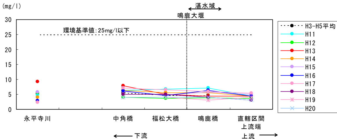
図 5.5-14 鳴鹿大堰年平均SSの縦断変化
