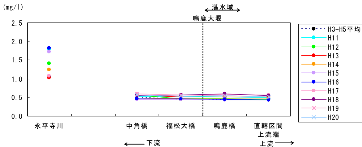
図 5.5-19 鳴鹿大堰年平均全窒素の縦断変化
