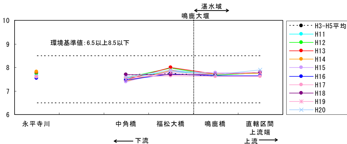
図 5.5-15 鳴鹿大堰年平均pHの縦断変化
