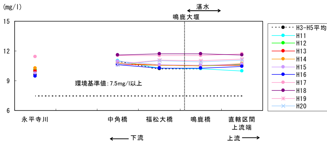
図 5.5-16 鳴鹿大堰年平均DOの縦断変化
