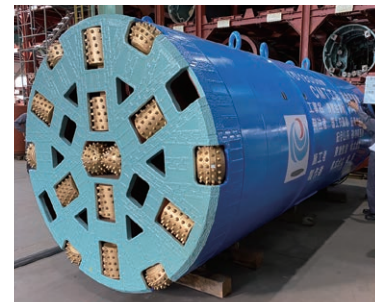
排水トンネル工事に使用する掘削機
