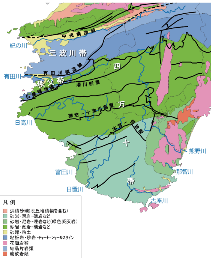
図3 紀伊山地地質図 (50万分の1 土地分類基本調査 GIS データ、他より作成)
