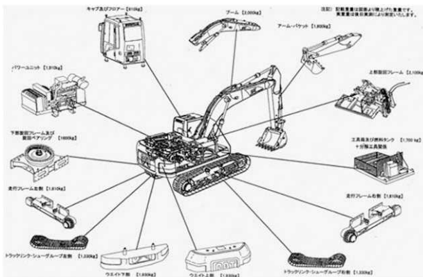
図 16 13 個のパーツに分解 (分解型油圧ショベル (中部地方整備局所有))
