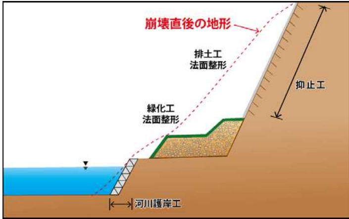
図 12 斜面对策
