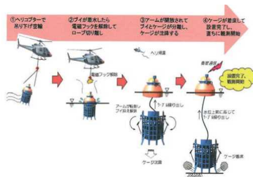
図 15 水中投下の仕組み
