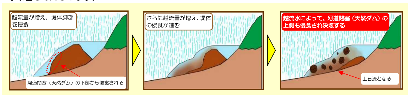
図8 崩壊過程（越流侵食）
