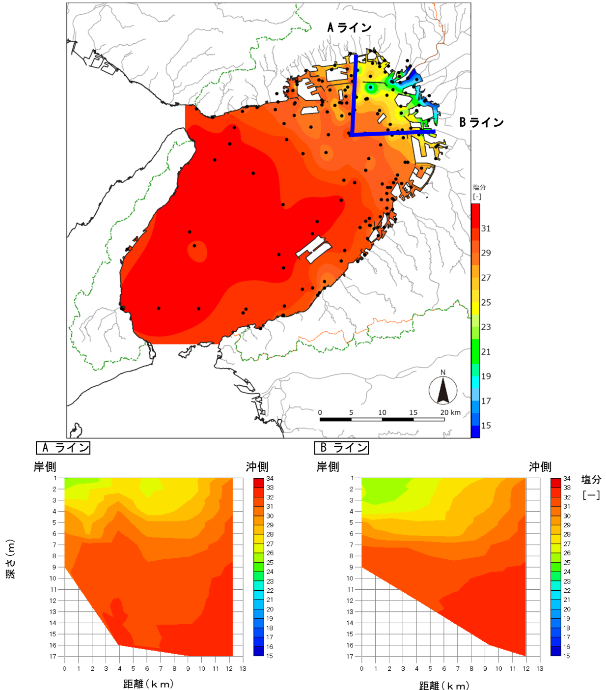
図 9 塩分の調査結果
