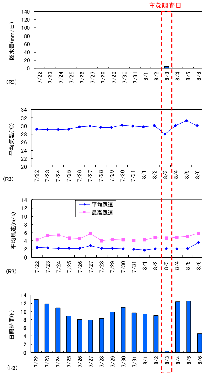
図 2 調査日前後の気象状況（大阪管区气象台）
