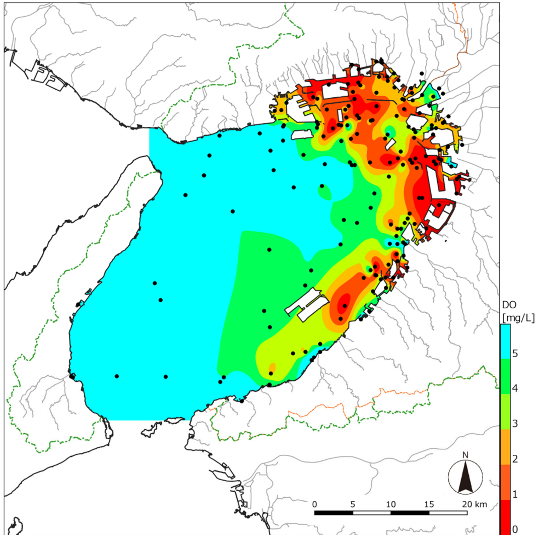
図 3 水質の水平分布（底層：DO）
