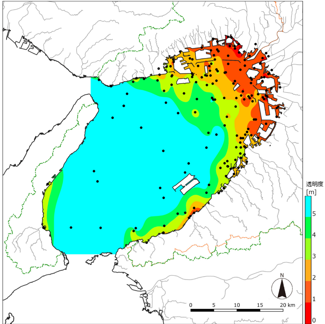
図 7 水質の水平分布（透明度）
