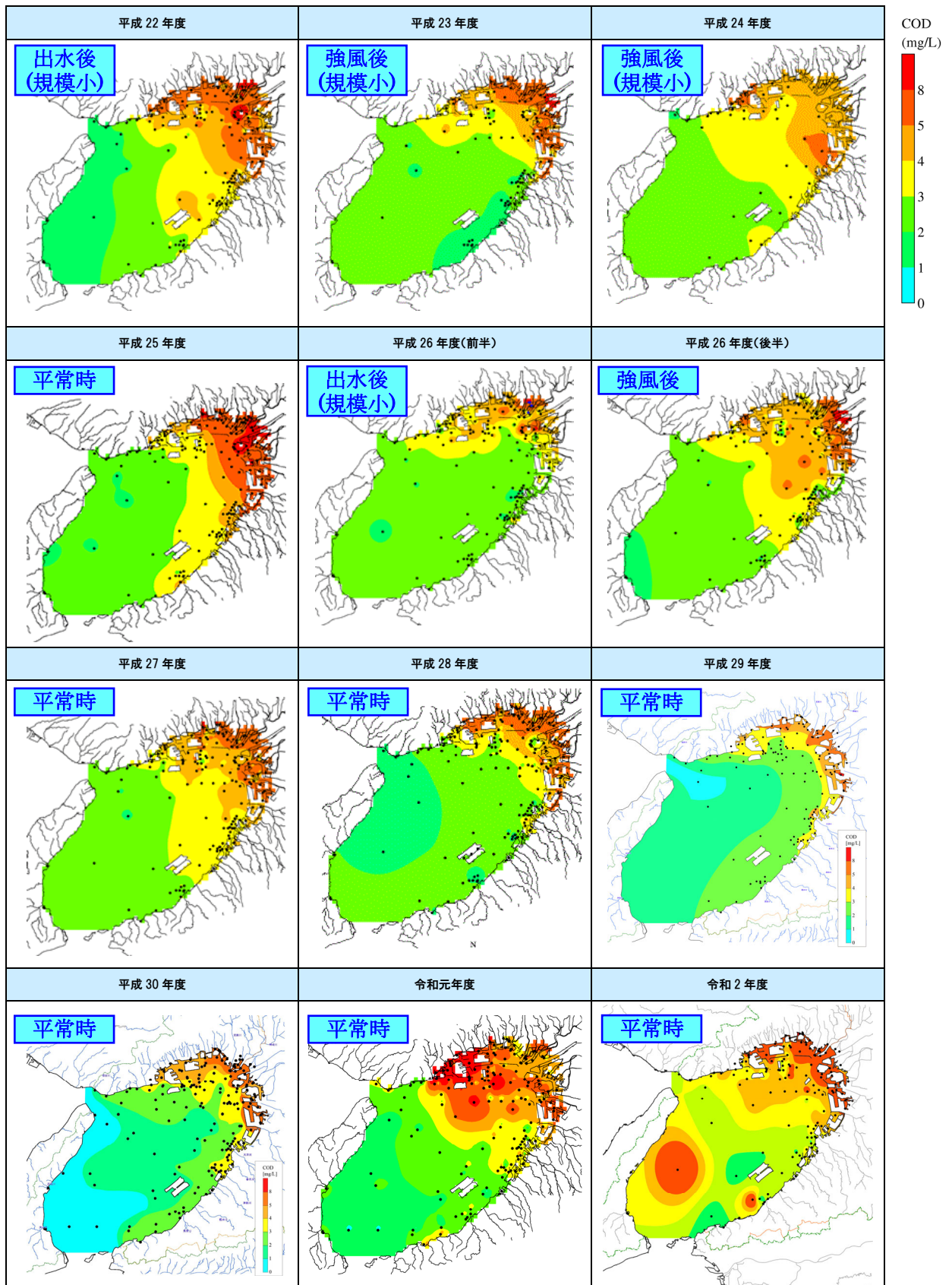
図 13 (2) 表層CODの水平分布図
