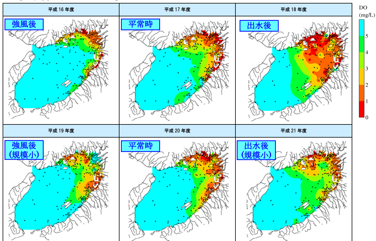
図 11 (1) 底層DOの水平分布図
