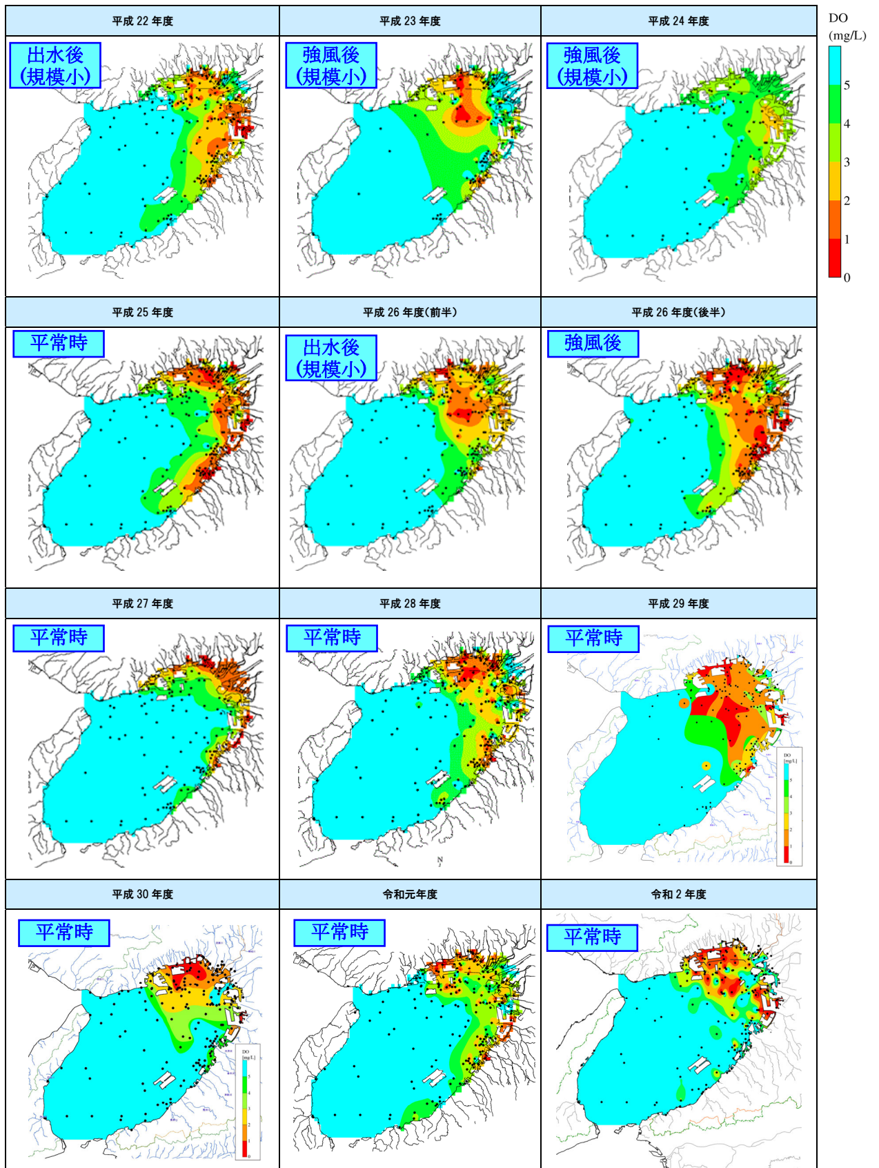
図 11 (2) 底層DOの水平分布図
