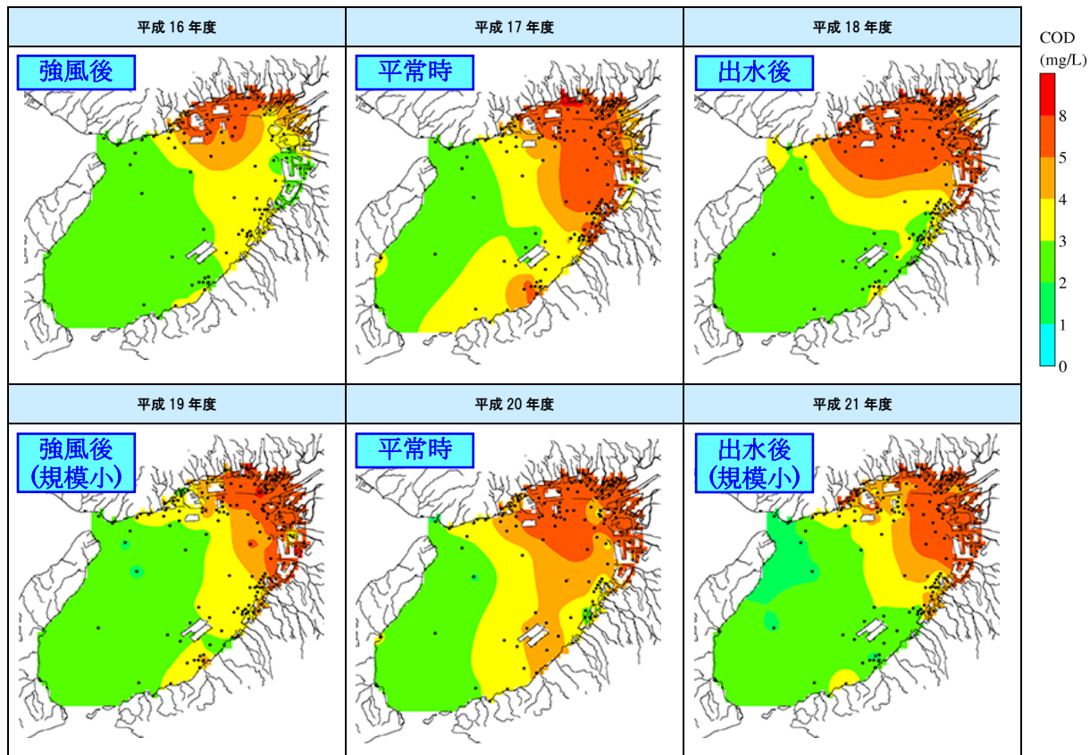
図 13 (1) 表層CODの水平分布図
