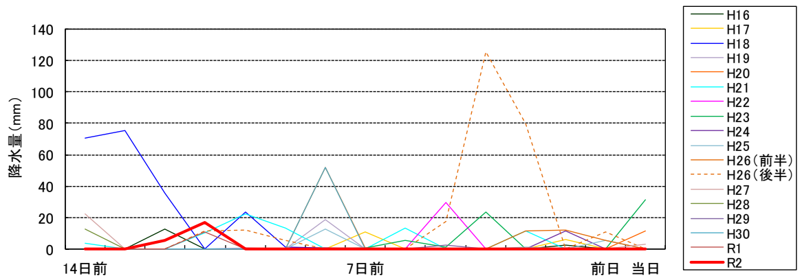
図 10 調査日前後の気象状況 (大阪管区气象台)
