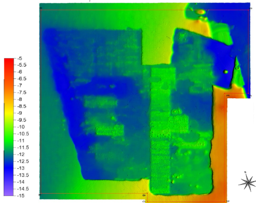
水深図(測量日:令和2年2月3~4日)
