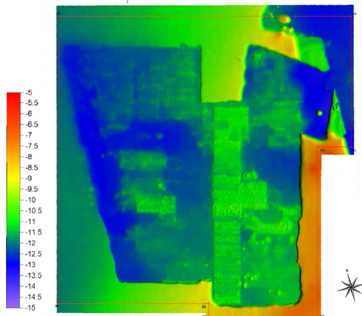
図 55 窪地の埋め戻し実施場所
