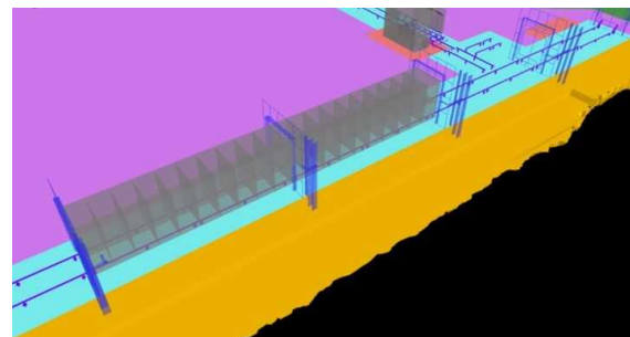
図-3 施工 CIM による PCa 部材管理 (基礎通廊)
