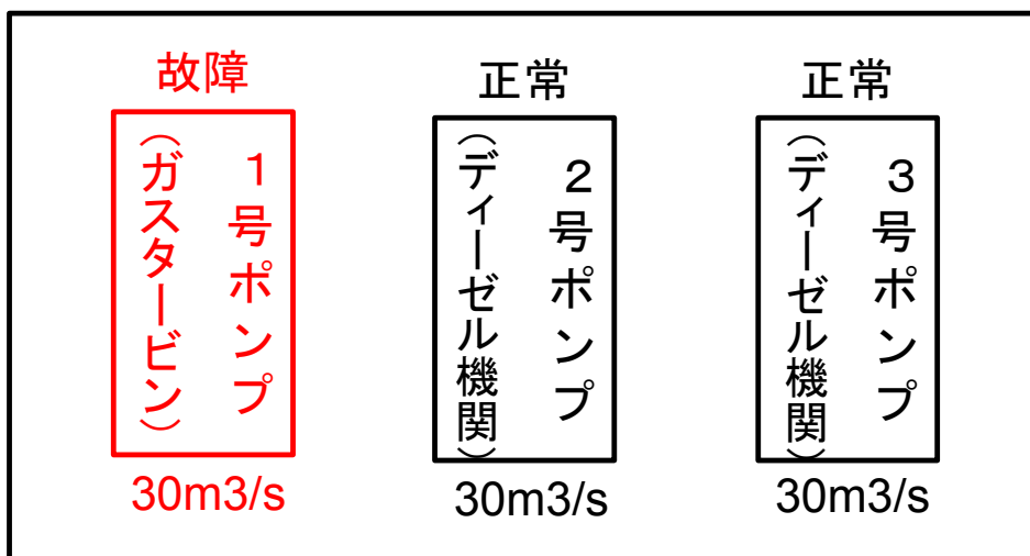
久御山排水機場ポンプ配置図
