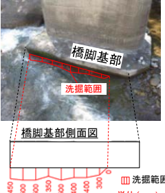
橋脚の洗掘
