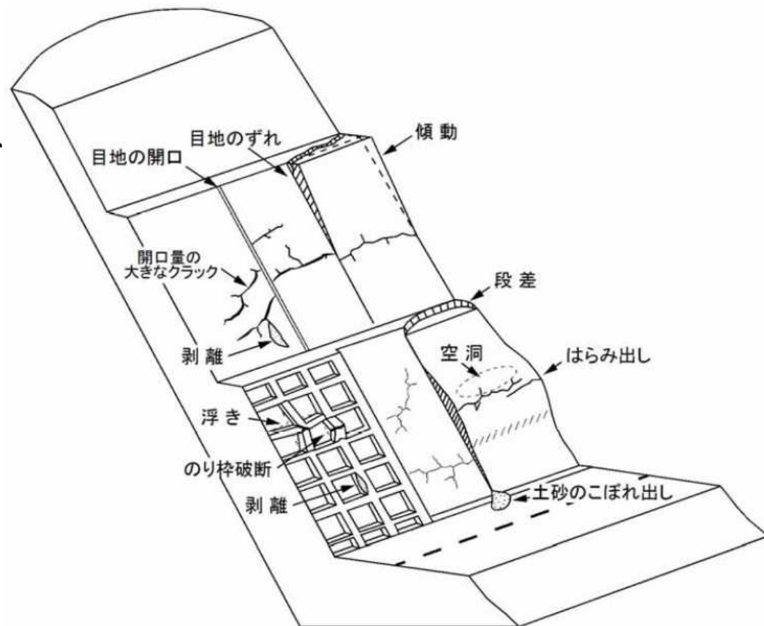
図 切土のり面の点検の着眼点 4725
