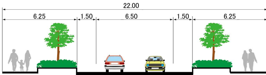
標準断面図 (単位：m)
