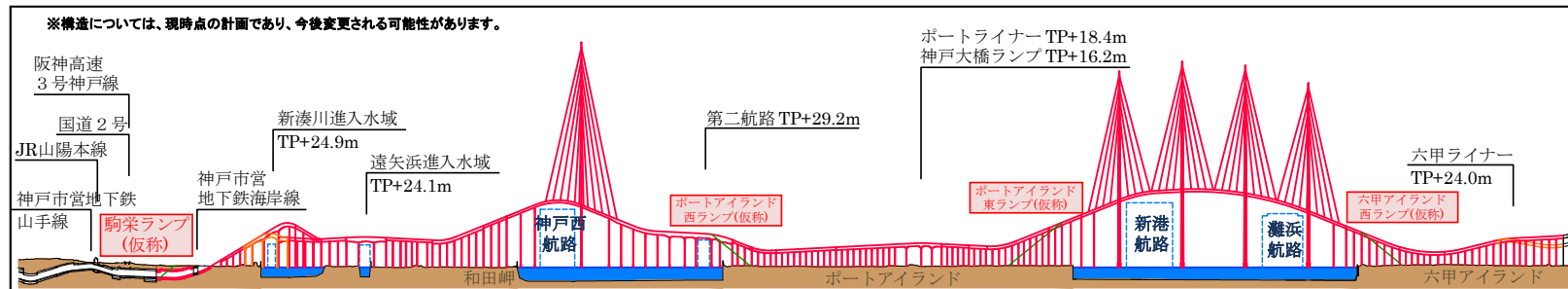
[ 縦断面図 ]
