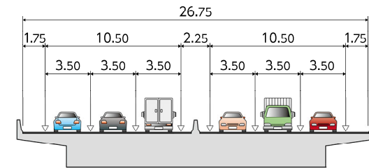
[ 標準断面図 ]
