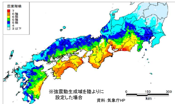
南海トラフ巨大地震の深度分布
