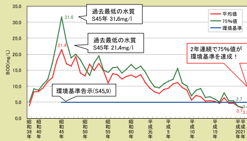
ようやく環境基準レベルにまで改善した水質(BOD値) 提供: 近畿地方整備局
