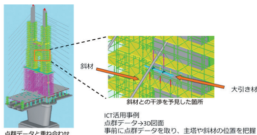
3次元モデル活用による施工計画
