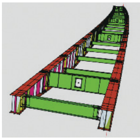
シミュレーション仮組
