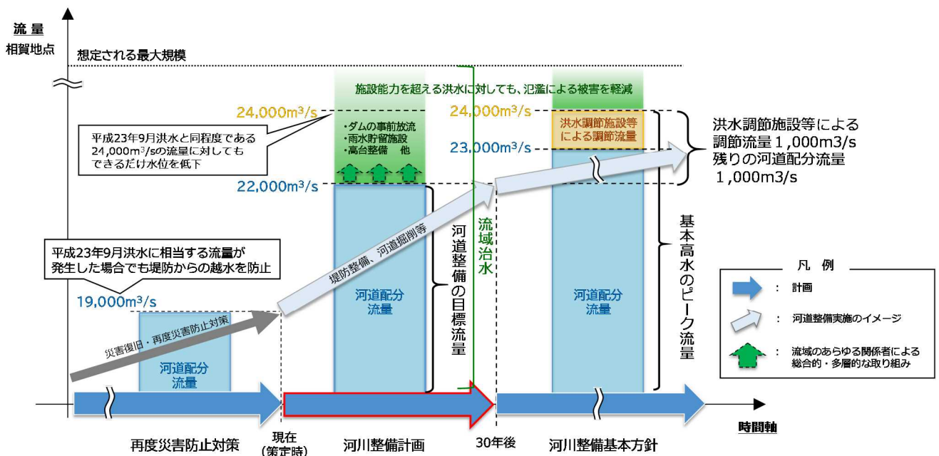
図-3.3 新宮川水系河川整備基本方針の目標に向けた段階的な整備イメージ図
