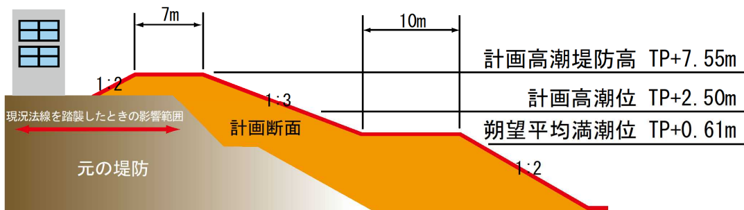
図-2.2 高潮堤防整備イメージ
