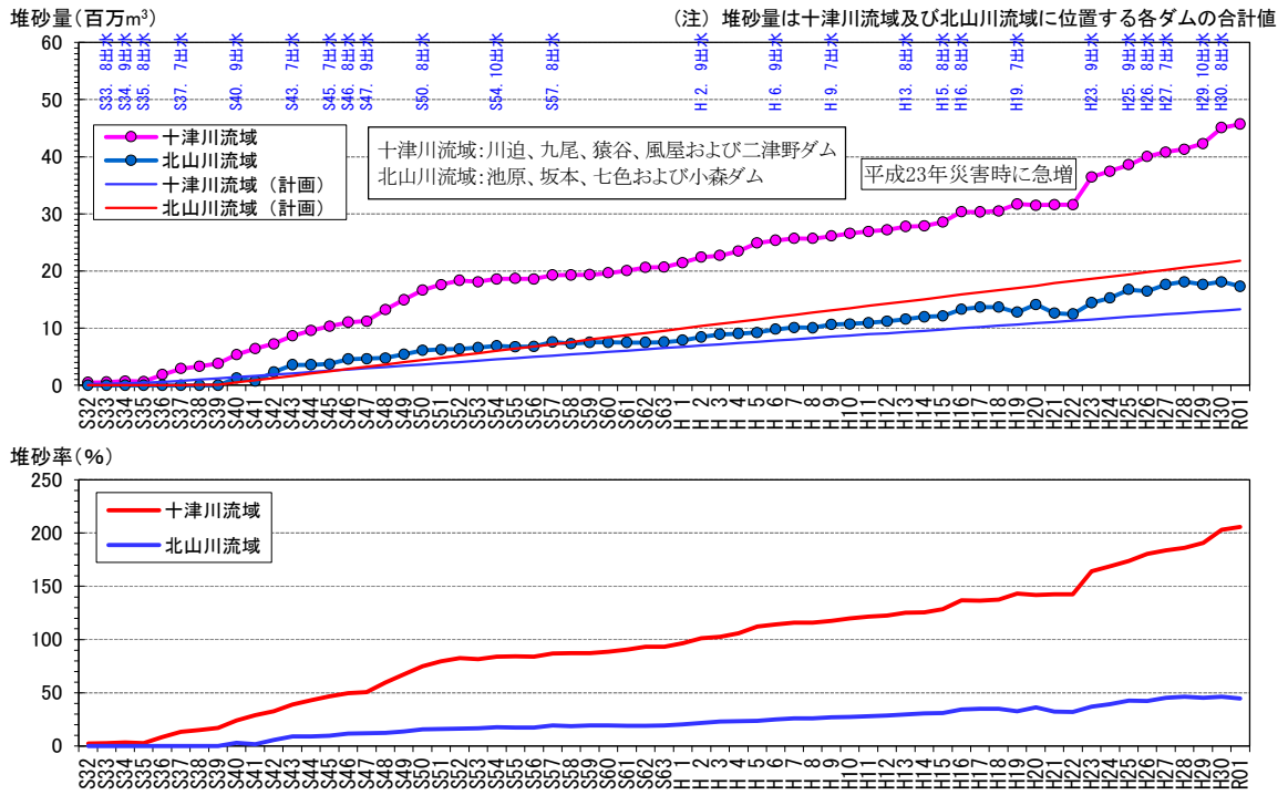
※堆砂率：十津川流域及び北山川流域ごとの堆砂量を計画堆砂量で除した割合 図-2.17 ダム堆砂量の経年変化
