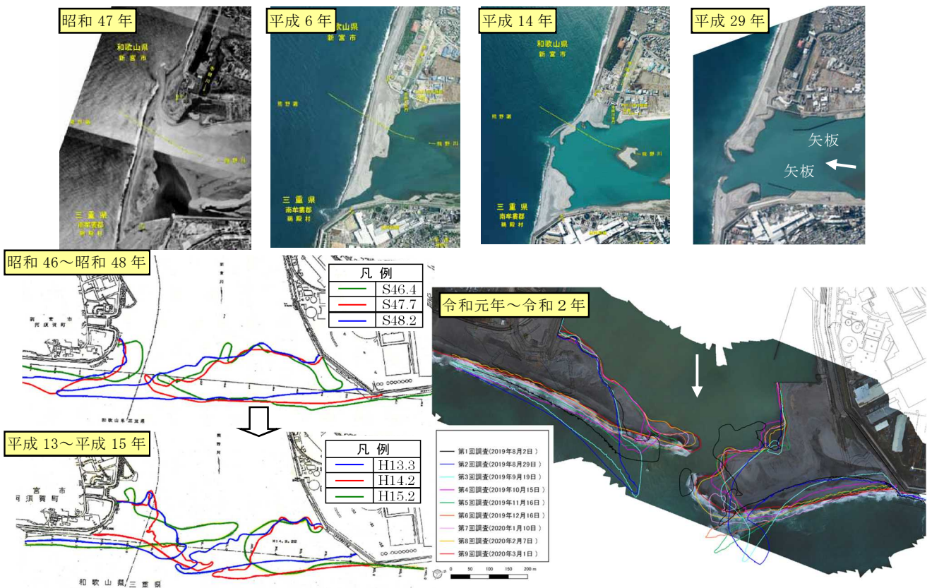
図-2.18 熊野川河口部砂州の経年変化
