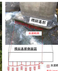
橋脚の洗掘
