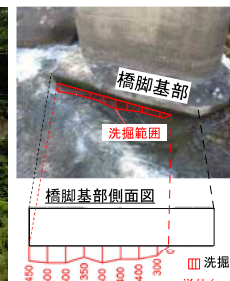
橋脚の洗掘
