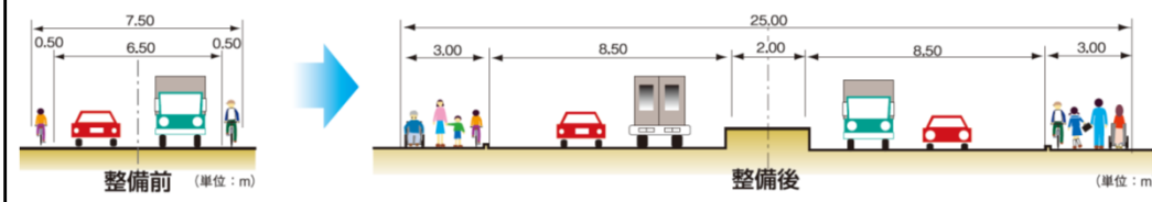
【標準横断面】
