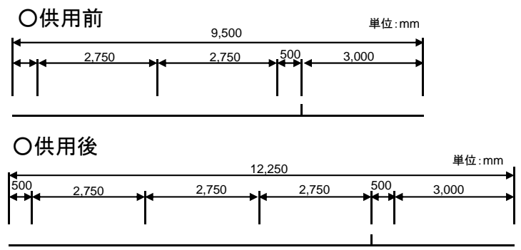
【標準横断図】
