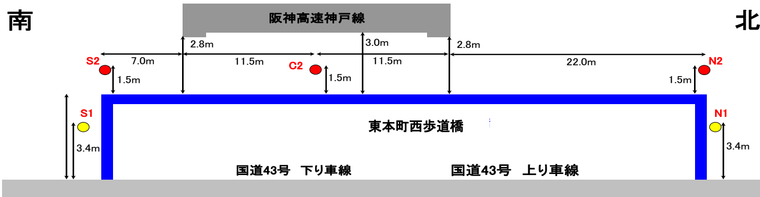
断面図
