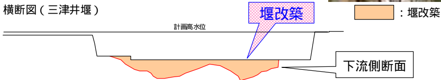
図-4.1.11 岸田地区の河川整備イメージ
