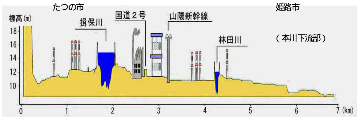
図-2.1.1 揖保川流域の横断構造(本川下流部 8.0k 付近)
