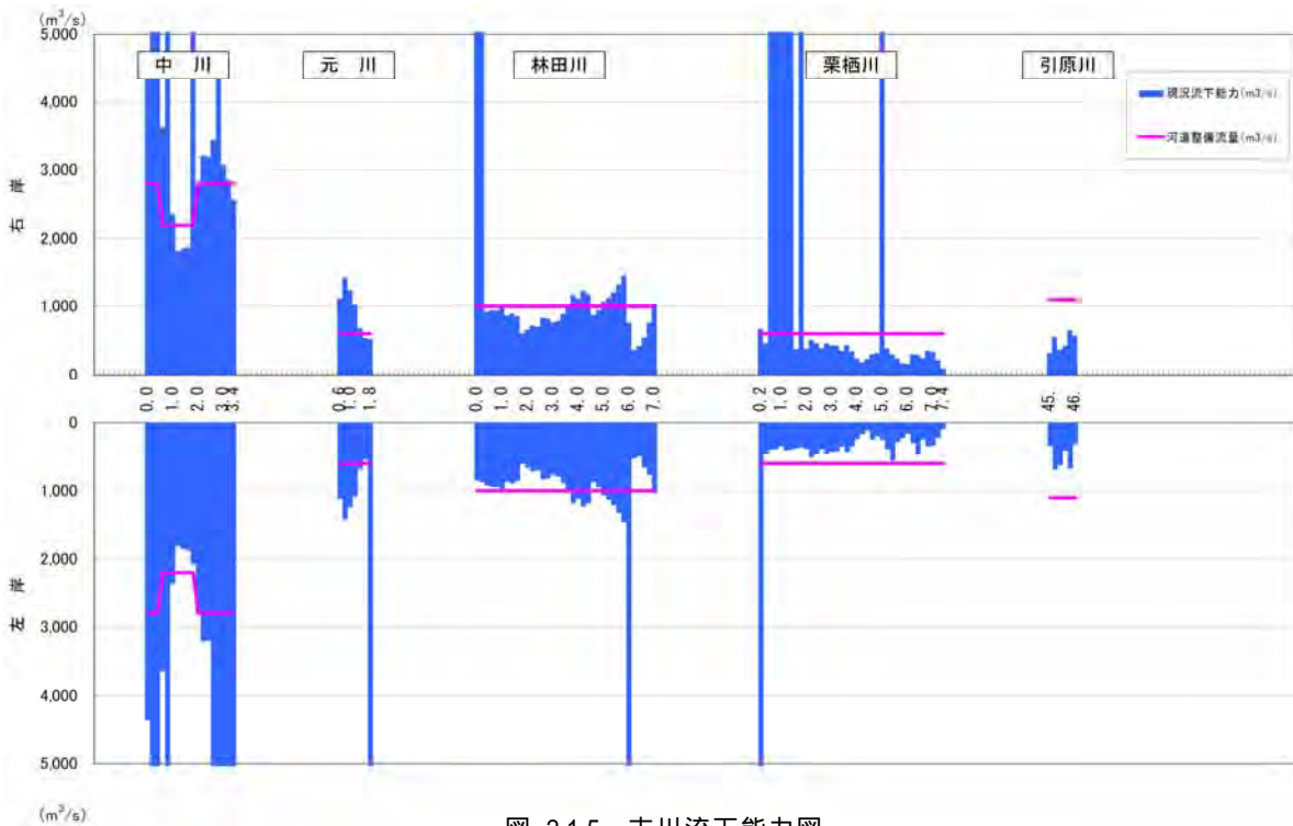
図-2.1.5 支川流下能力図
