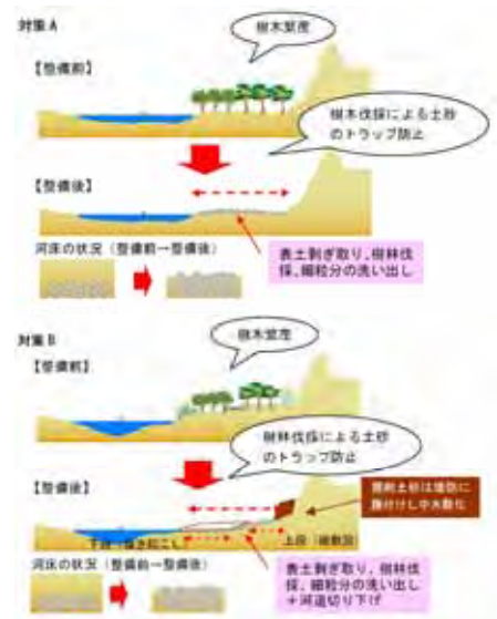
図-4.3.2 樹林化対策例
