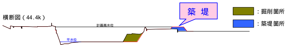
図-4.1.14 関賀地区の河川整備イメージ
