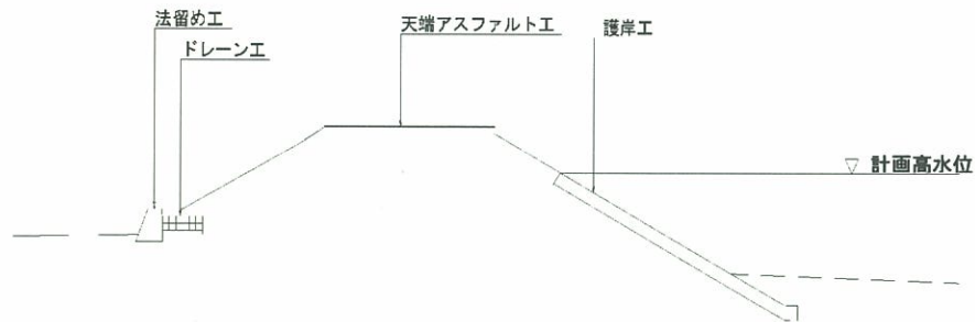
一般部堤防強化の例
