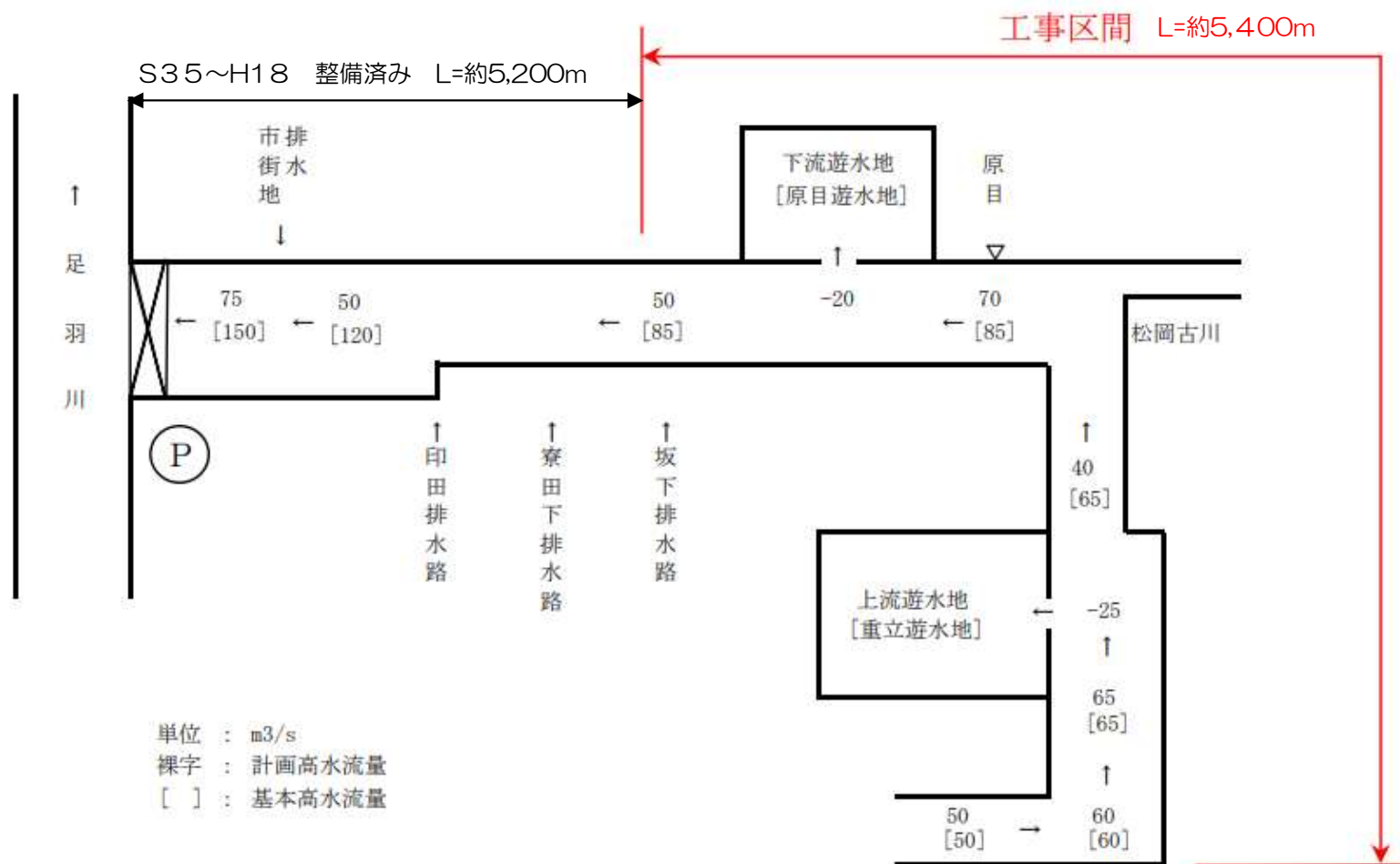
計画流量配分図(河川整備計画目標1/30)
