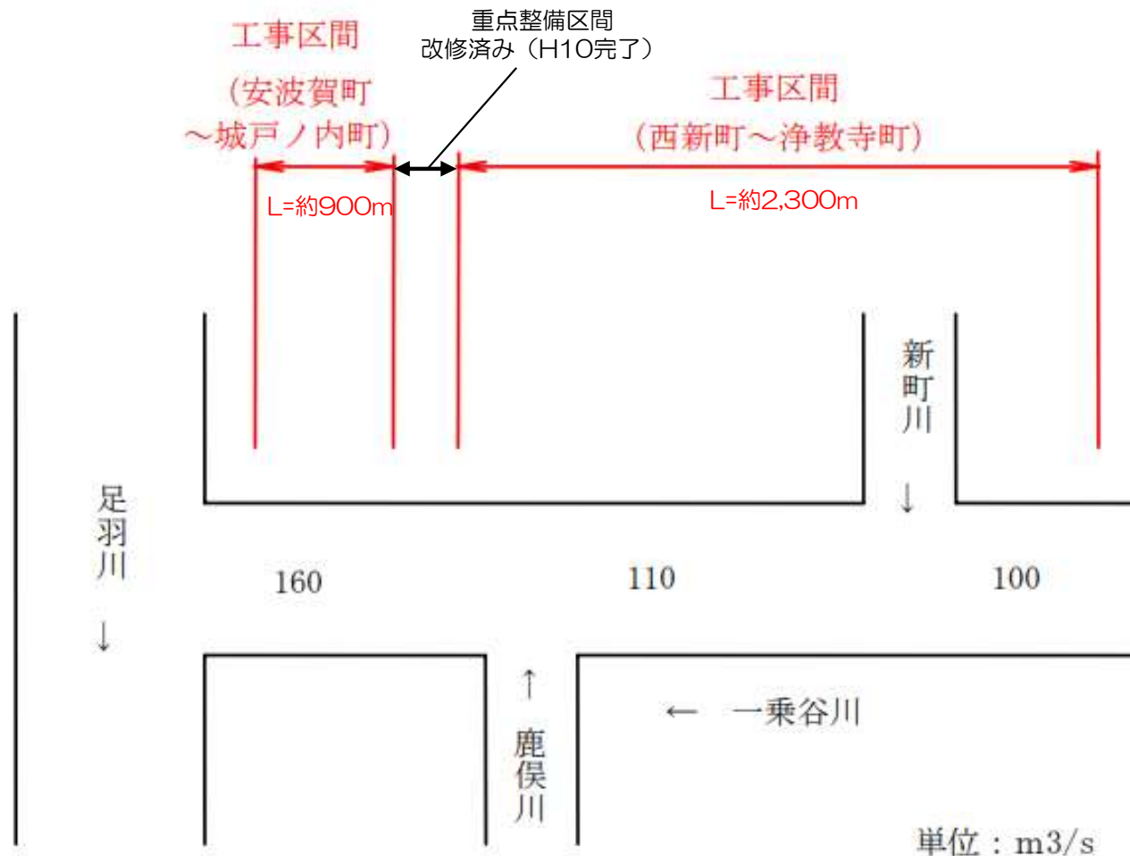
計画流量配分図(河川整備計画目標1/10)
