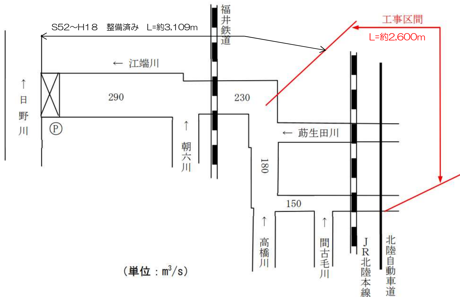
計画流量配分図(河川整備計画目標1/50)
