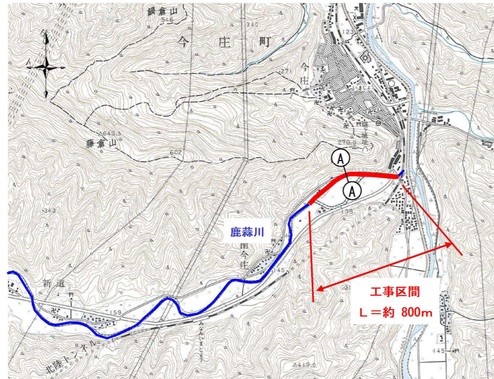
図 5.32 平面図
