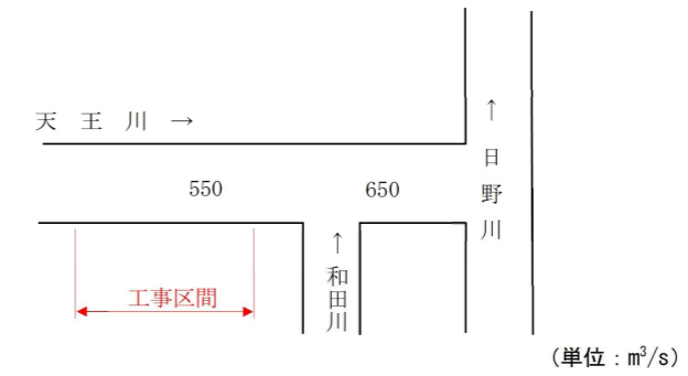
図 5.21 計画流量配分図
