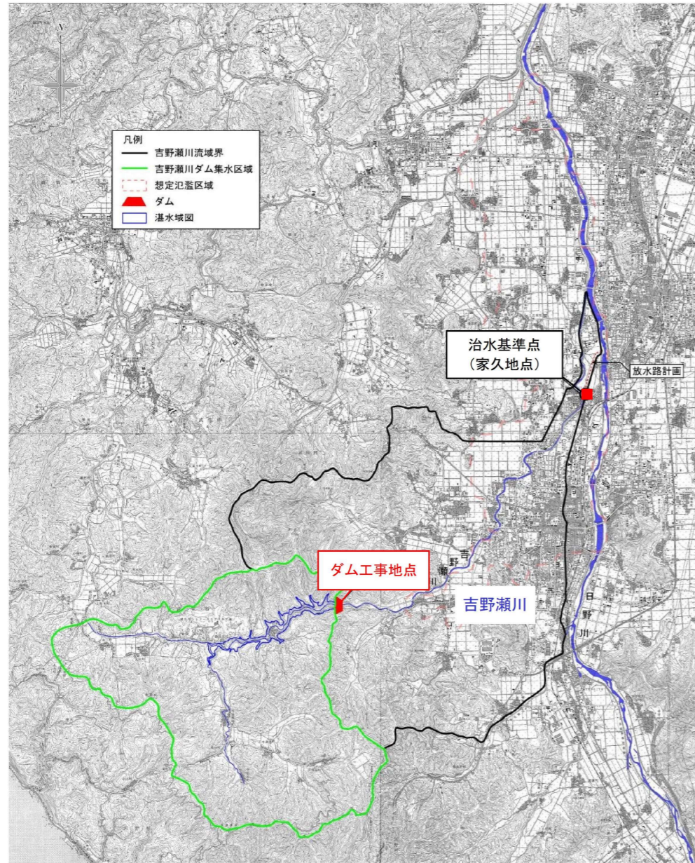
図 5.26 ダム位置図
