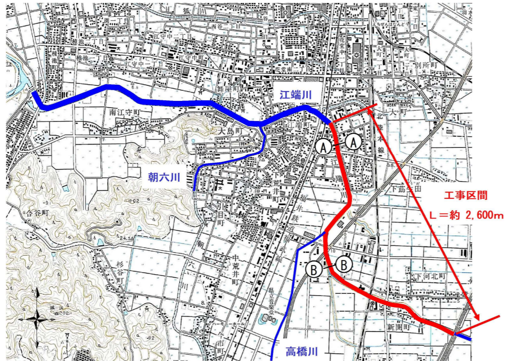
図 5.13 平面図
