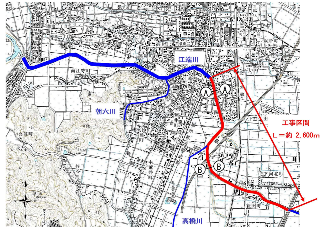
図 5.13 平面図
