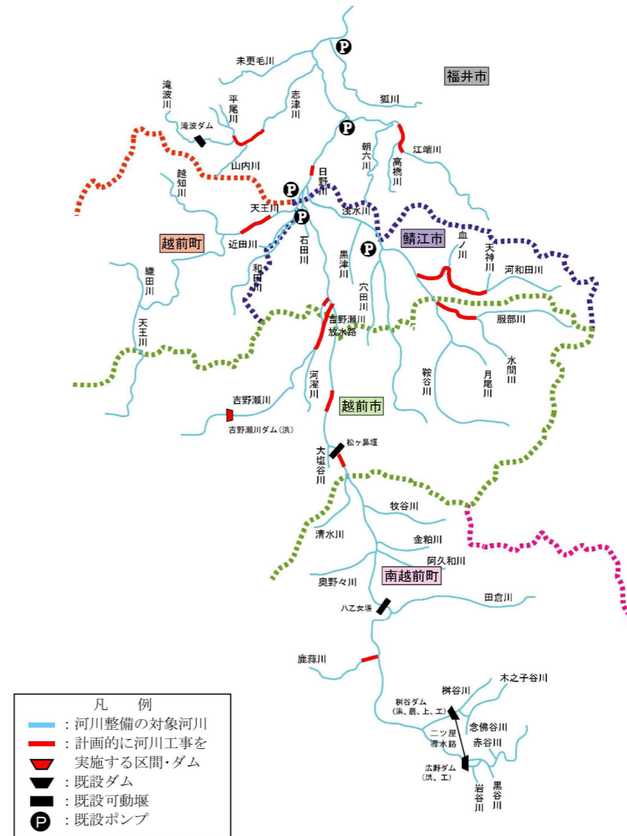
図 5.1 計画的に河川工事を実施する区間
