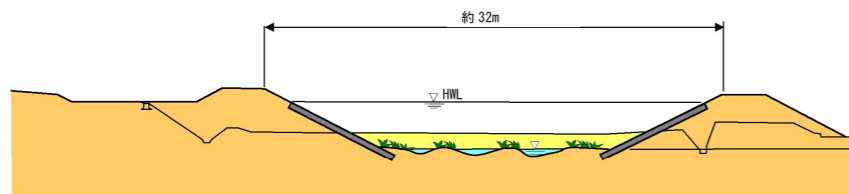
図 5.33 横断面(イメージ)
