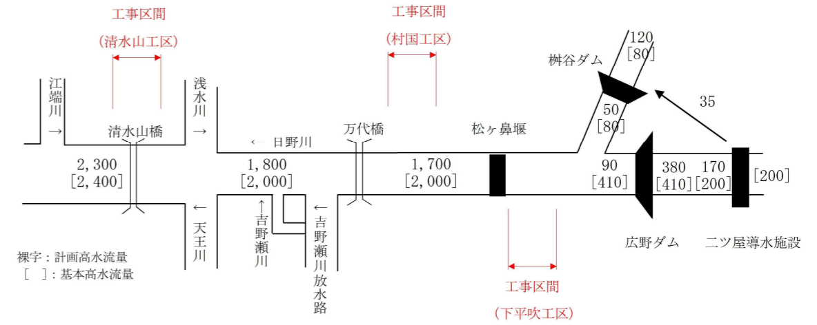
図 5.2 計画流量配分図
