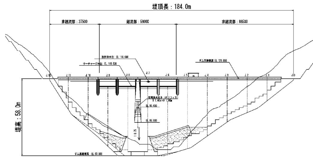
図 5.28 下流面図
