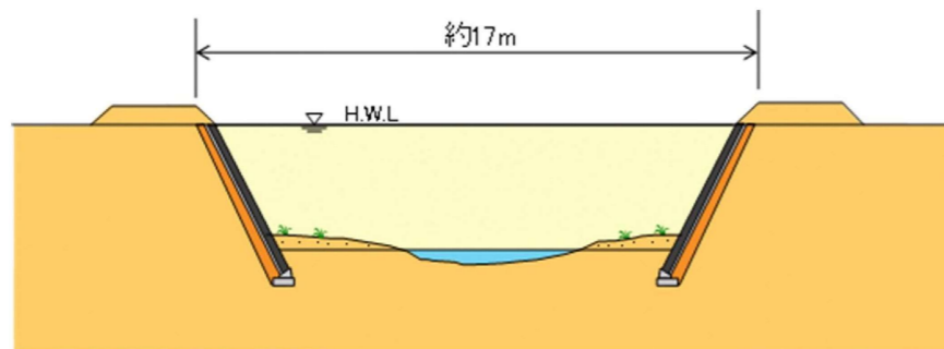
図 5.20 横断面図(イメージ)
