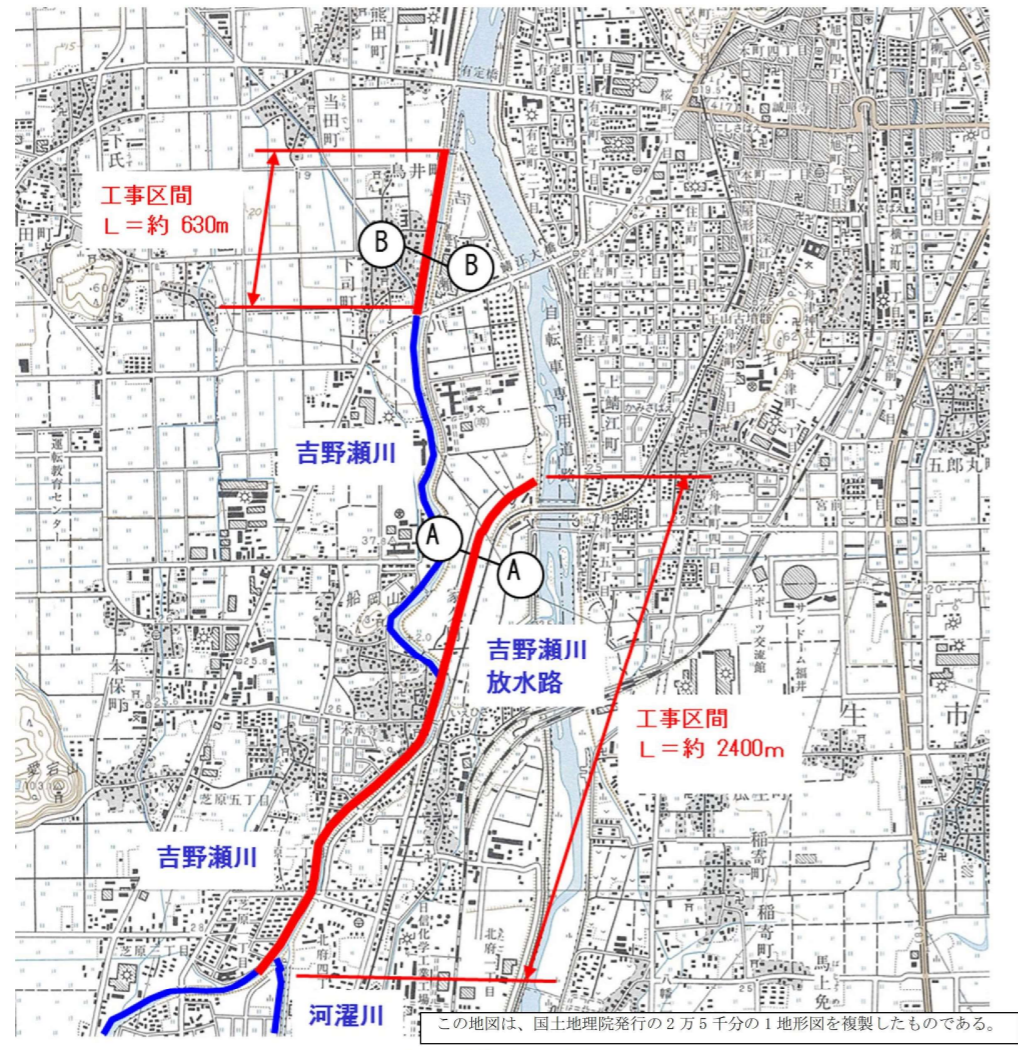
図 5.29 平面図
