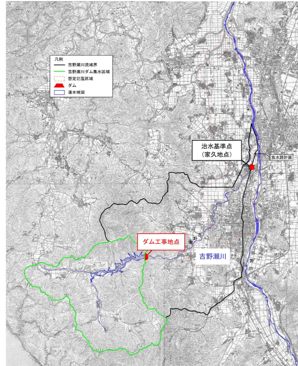
図 5.26 ダム位置図
