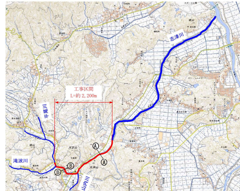
図 5.10 平面図
