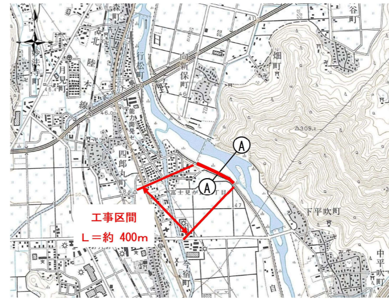
図 5.7 平面図
