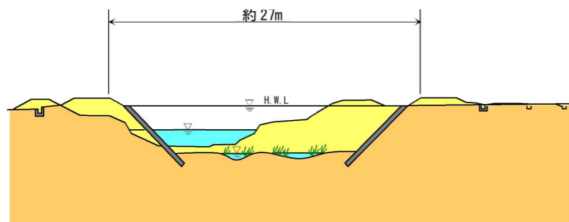
図 5.17 横断面(イメージ)
