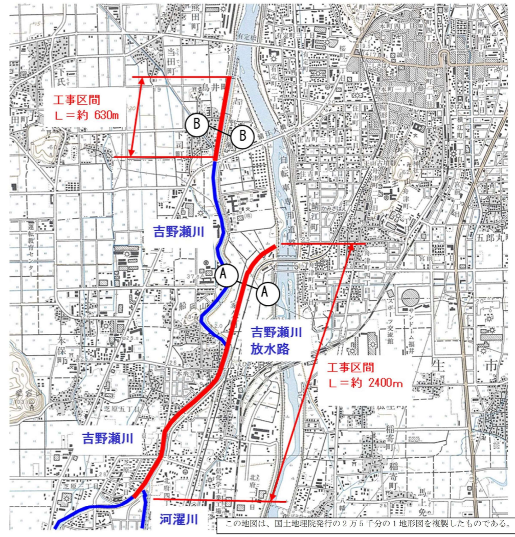
図 5.29 平面図
