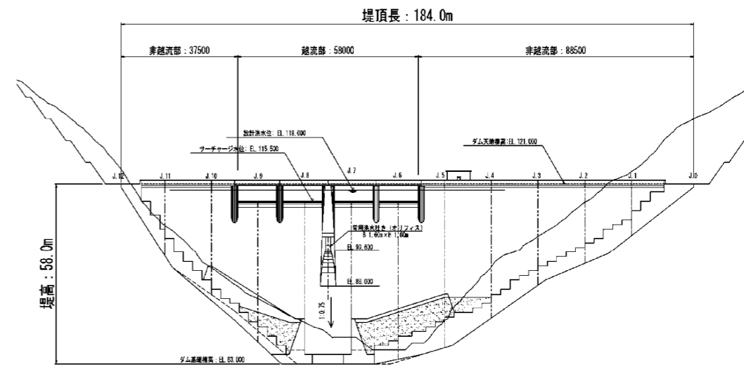
図 5.28 下流面図
