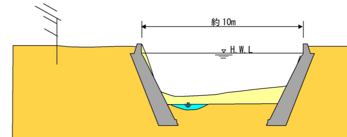
図 5.11 横断面図(イメージ)
