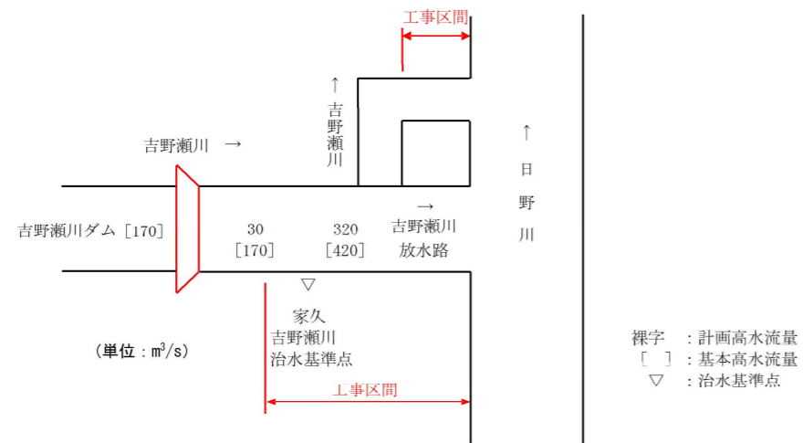
図 5.24 計画流量配分図
