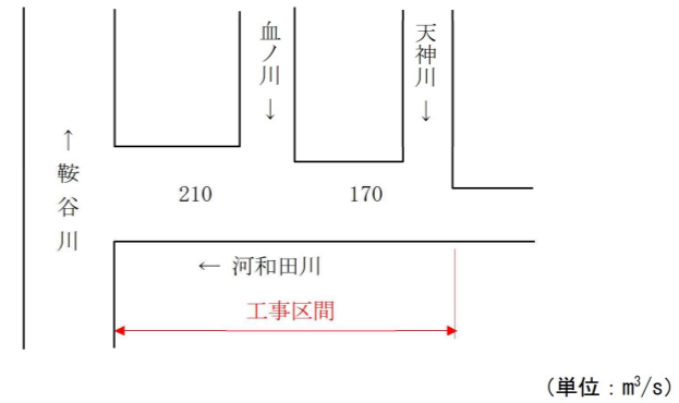
図 5.15 計画流量配分図
