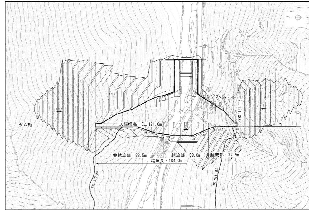
図 5.27 平面図
