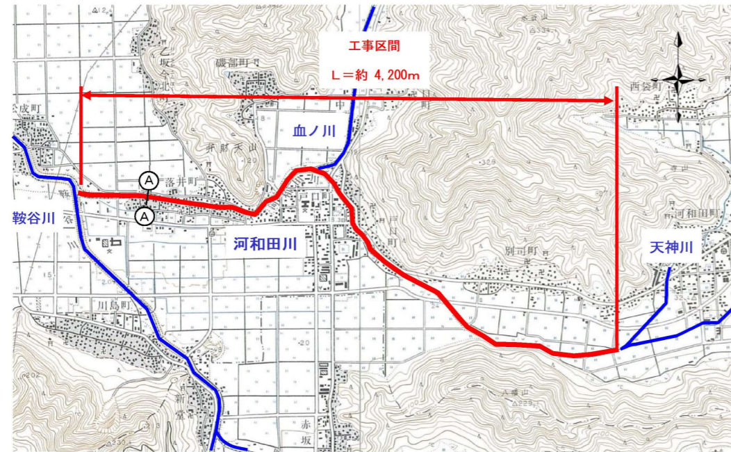
図 5.16 平面図
