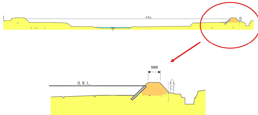
図 5.6 横断面(イメージ)
