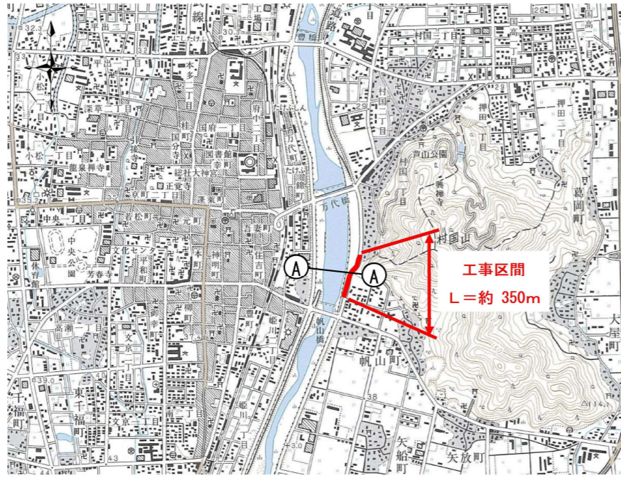
図 5.5 平面図
