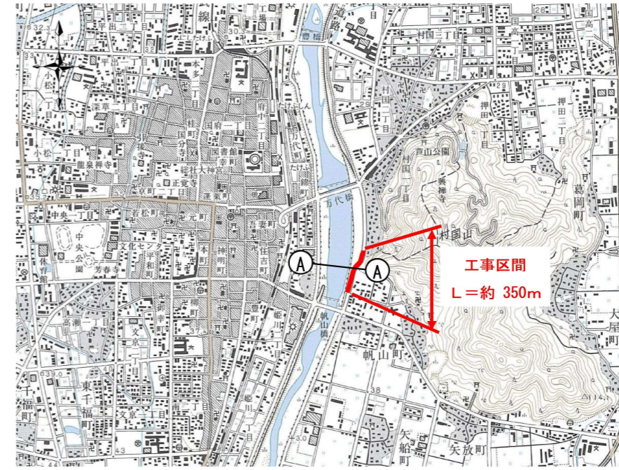
図 5.5 平面図
