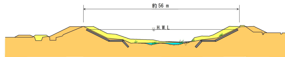
図 5.23 横断面(イメージ)
