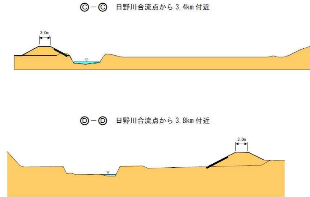
図 5.34 横断面(イメージ)
