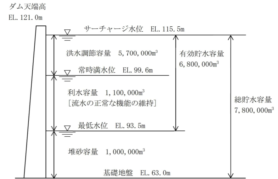
図 5.25 ダム容量配分図
