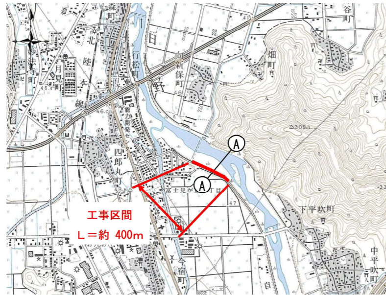
図 5.7 平面図
