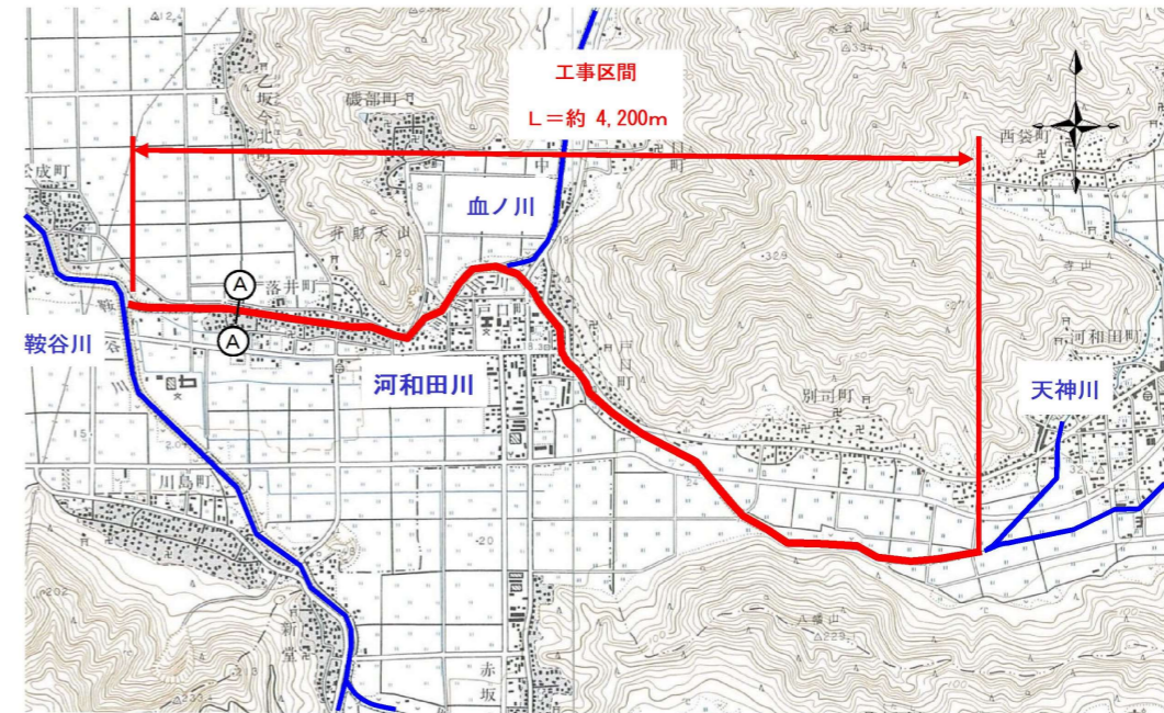
図 5.16 平面図
