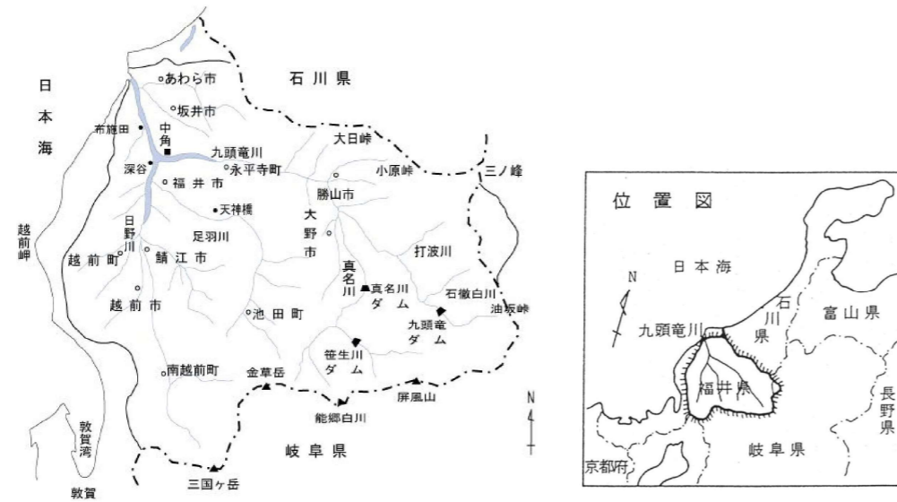
図 1.1 九頭竜川水系概要図
