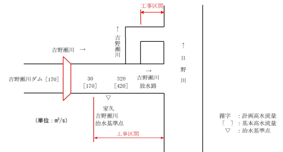
図 5.24 計画流量配分図
